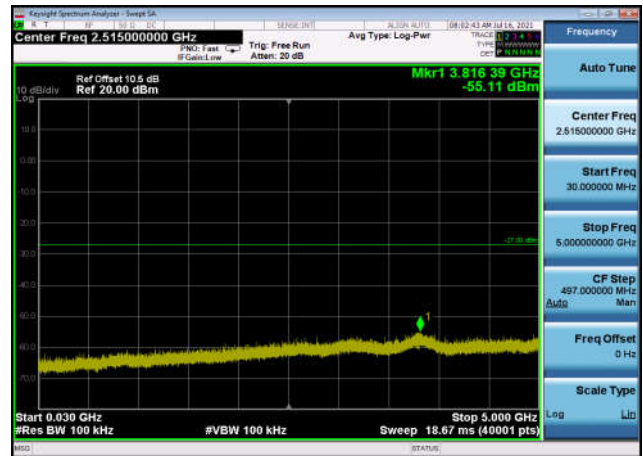
U-NII-3 ,Plot 2,30MHz~5000MHz-802.11n (20MHz),5825MHz,Ant0
