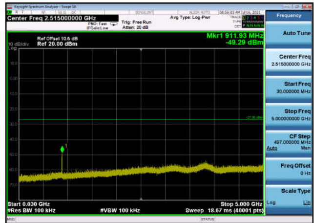
U-NII-3 ,Plot 2,30MHz~5000MHz-802.11a c(40MHz),5755MHz,Ant0
