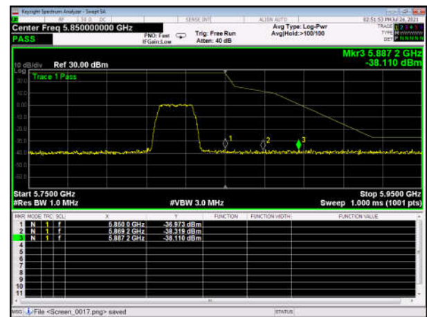
U-NII-3 ,Plot 1,Band Edge-802.11ac(20 MHz),5825MHz,Ant0
