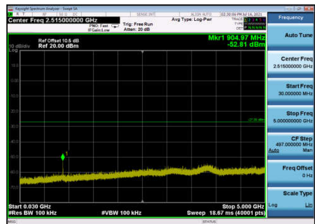
U-NII-3 ,Plot 2,30MHz~5000MHz-802.11a x(40MHz),5755MHz,Ant0
