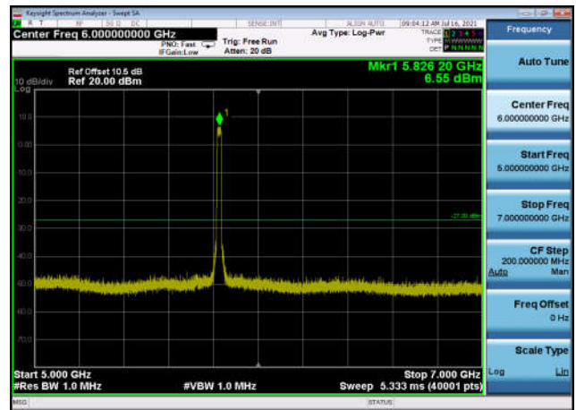
U-NII-3 ,Plot 3,5000MHz~7000MHz-802.1 1ac(40MHz),5795MHz,Ant0
