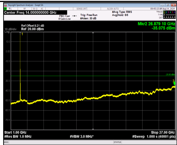
7-7-10MHz-20MHz-QPSK-QPSK-20805-20949-1RB#0-0RB #0-1000~27000MHz-PASS
