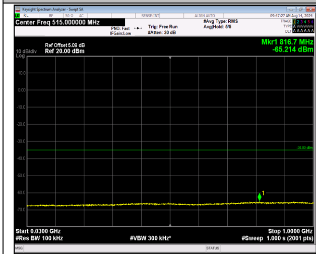
7-7-10MHz-20MHz-QPSK-QPSK-20805-20949-1RB#0-1 RB#99-30~1000MHz-PASS
