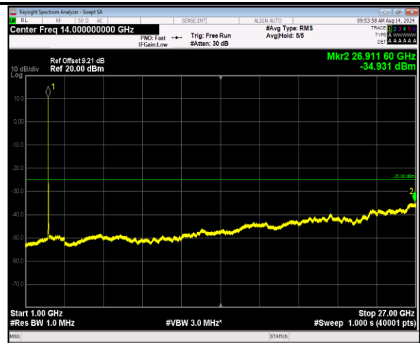
7-7-10MHz-20MHz-QPSK-QPSK-21006-21150-50RB#0-100RB#0-1000~27000MHz-PASS
