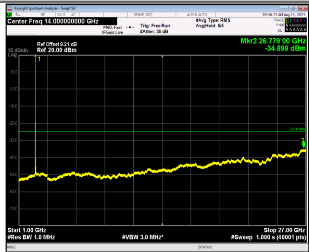
7-7-10MHz-20MHz-QPSK-QPSK-20805-20949-1RB#49-0R B#0-1000~27000MHz-PASS
