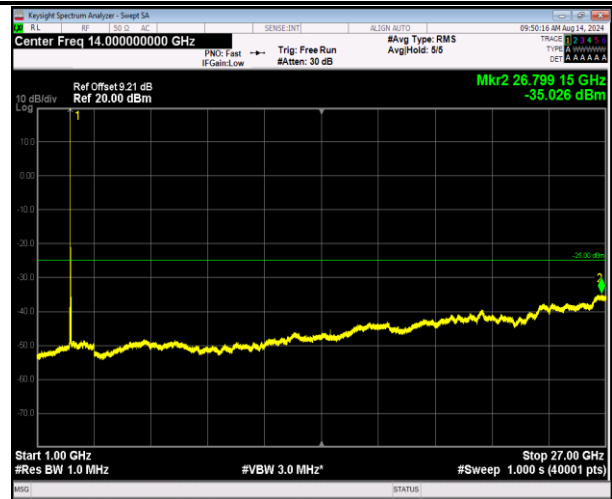
7-7-10MHz-20MHz-QPSK-QPSK-21006-21150-1RB#0-0RB #0-1000~27000MHz-PASS
