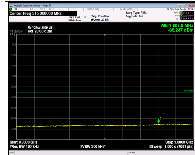
7-7-10MHz-20MHz-QPSK-QPSK-21206-21350-50RB#0-100RB#0-30~1000MHz-PASS
