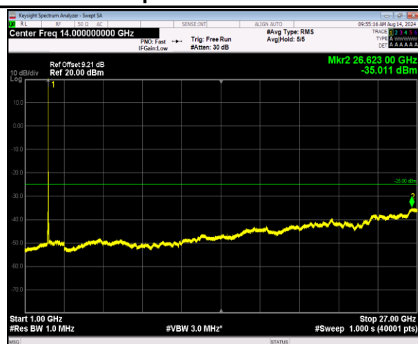
7-7-10MHz-20MHz-QPSK-QPSK-21206-21350-1RB#0-0RB #0-1000~27000MHz-PASS
