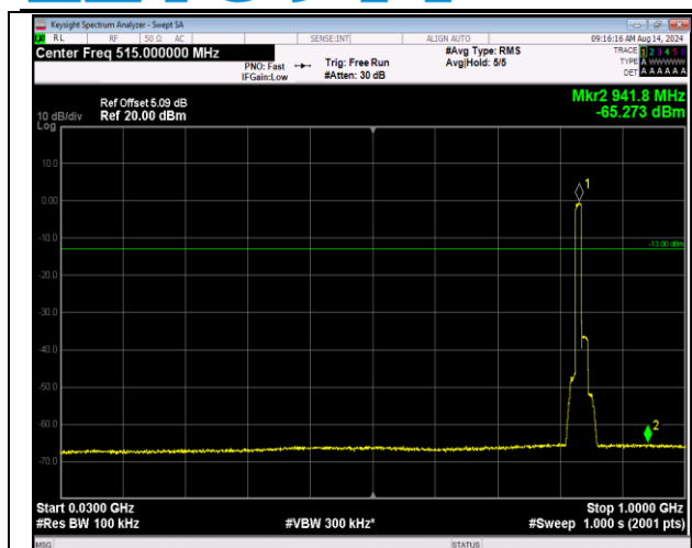
5-5-10MHz-10MHz-QPSK-QPSK-20501-20600-50RB#0-50RB#0-30~1000MHz-PASS
