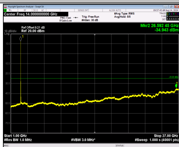
7-7-10MHz-20MHz-QPSK-QPSK-21206-21350-1RB#0-1RB #99-1000~27000MHz-PASS
