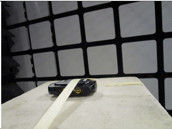
EUT Flat
