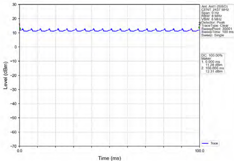
802.11b_MCH_2437MHz_Ant1 (SISO)_NTNV
