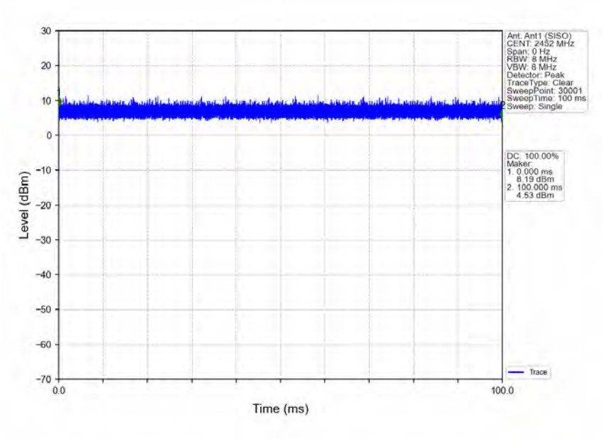
802.11n(HT40)_HCH_2452MHz_Ant1 (SISO)_NTNV
