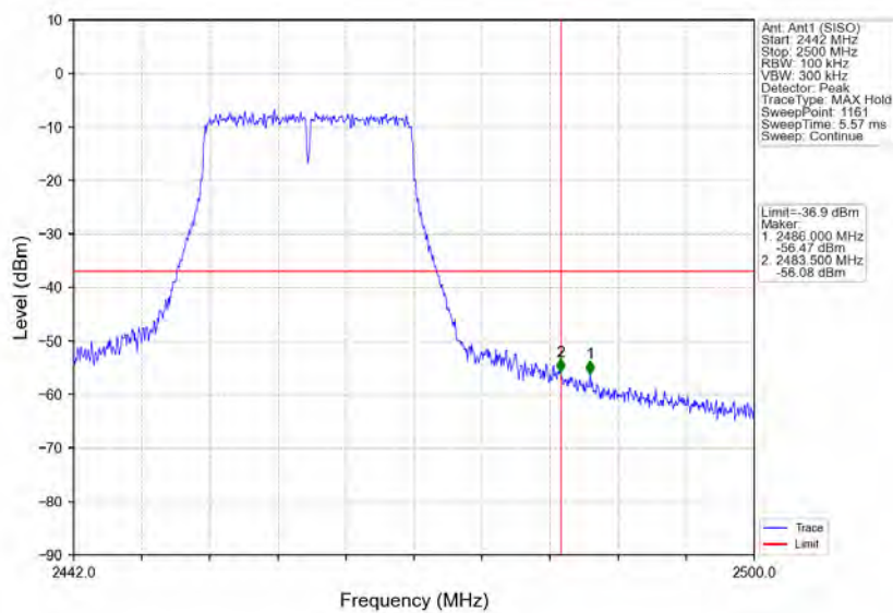
802.11n(HT20)_HCH_2462MHz_Ant1 (SISO)_NTNV
