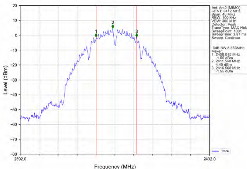
802.11b_LCH_2412MHz_Ant2 (MIMO)_NTNV
