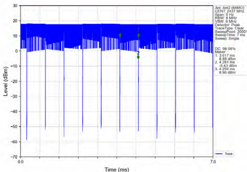
802.11b_MCH_2437MHz_Ant2 (MIMO)_NTNV
