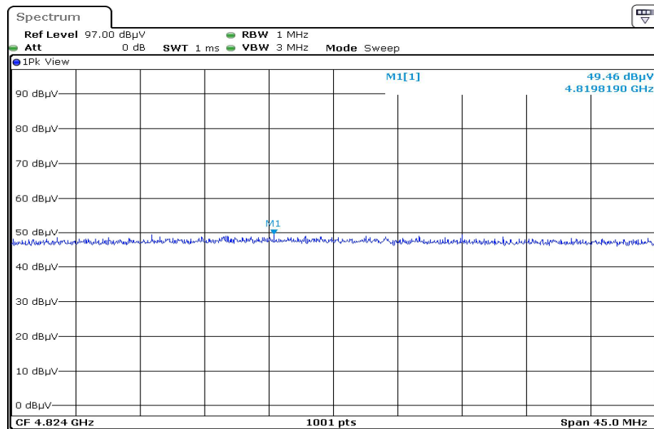
F1 X2 4824.0 Harmonic Horizontal PEAK
