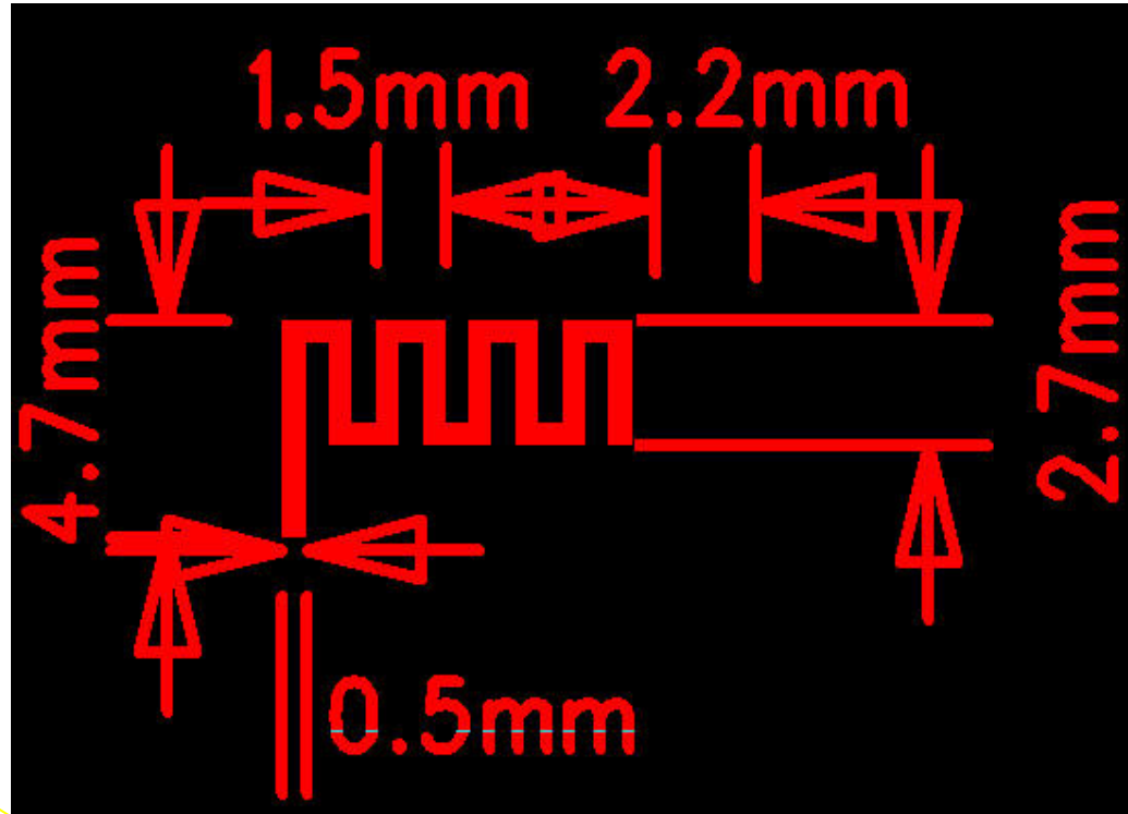
Antenna
