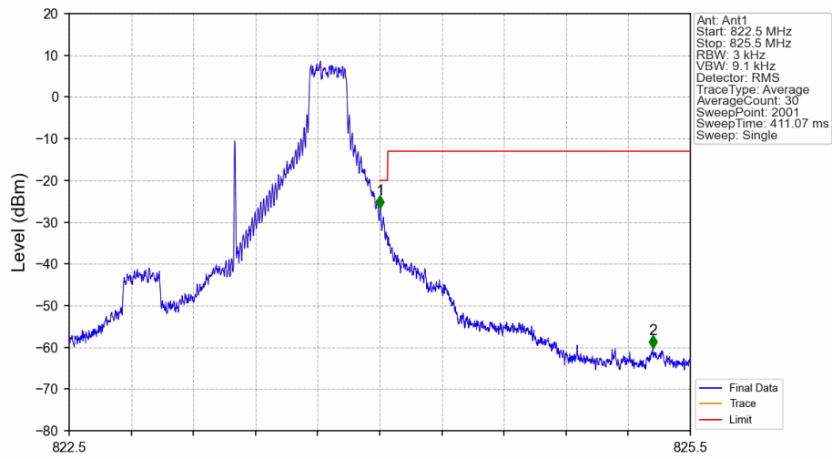
Band26a 1.4MHz QPSK HCH 823.3MHz RB 1 5 NTNV
