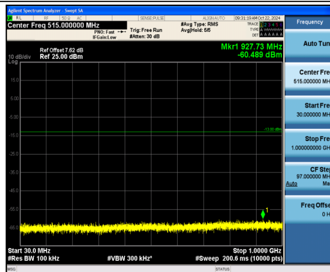
Band2-3MHz-QPSK-18615-1-0-Low-30-1000--60.49-PASS
