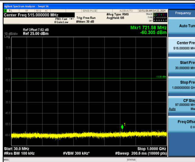
Band2-10MHz-QPSK-18900-1-0-Low-30-1000--60.31-PASS
