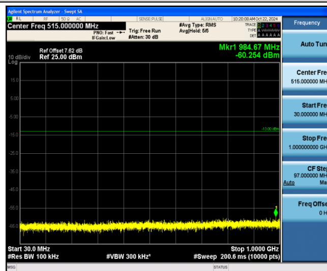
Band2-5MHz-QPSK-18900-1-0-Low-30-1000--60.25-PASS
