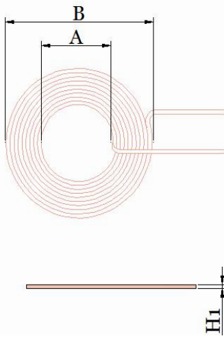
图一、线圈
