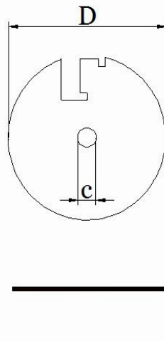
图二、硬磁片
