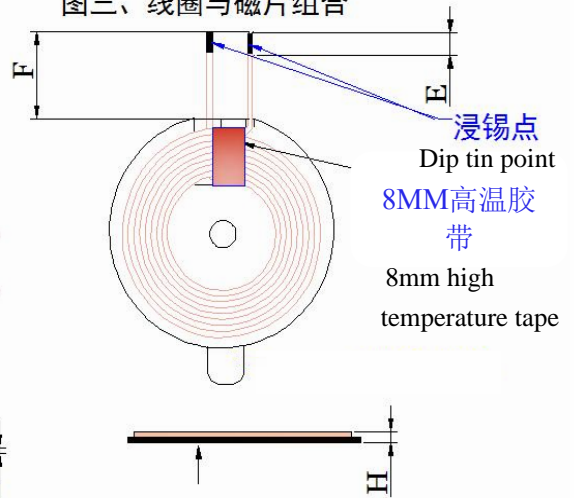
图三、线圈与磁片组合
