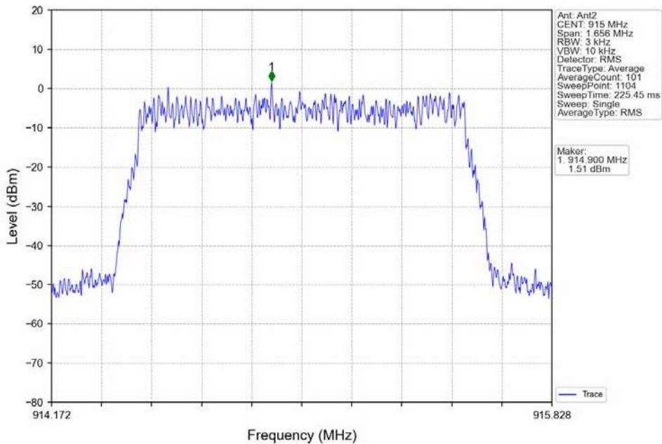
QPSK 1.4MHz_MCH_915MHz_MIMO_NTNV
