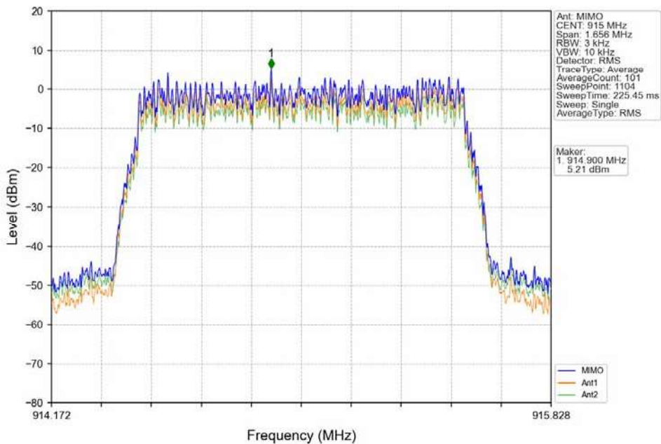
QPSK 1.4MHz_MCH_915MHz_MIMO_NTNV
