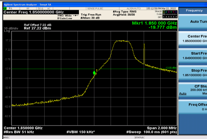
Band2-5MHz-QPSK-18625-1RB#0
