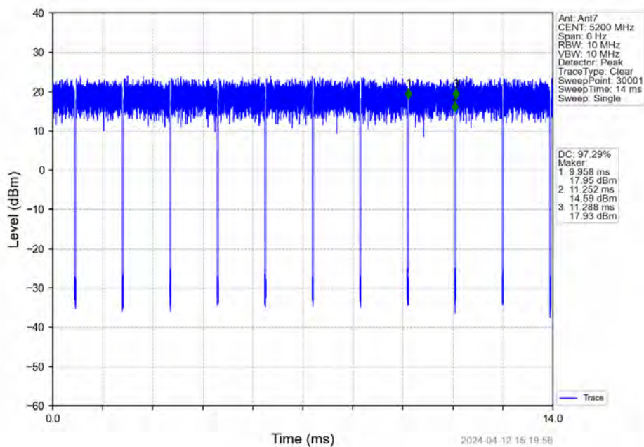
802.11n(HT20) MCH_5200MHz_Ant7_NTNV
