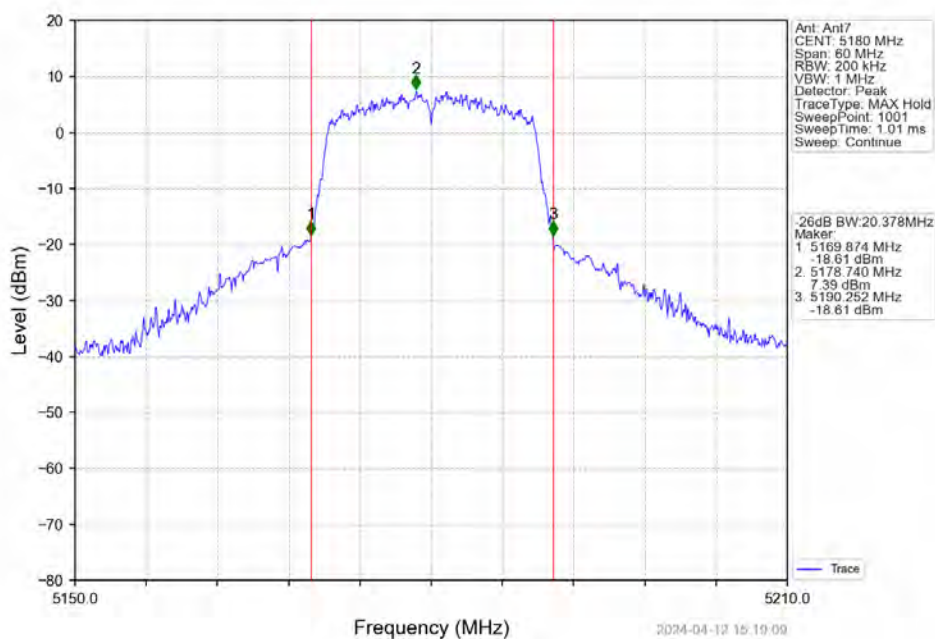
802.11n(HT20)_LCH_5180MHz_Ant7_NTNV
