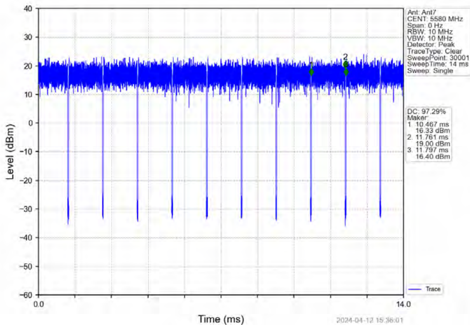
802.11n(HT20) MCH_5580MHz_Ant7_NTNV
