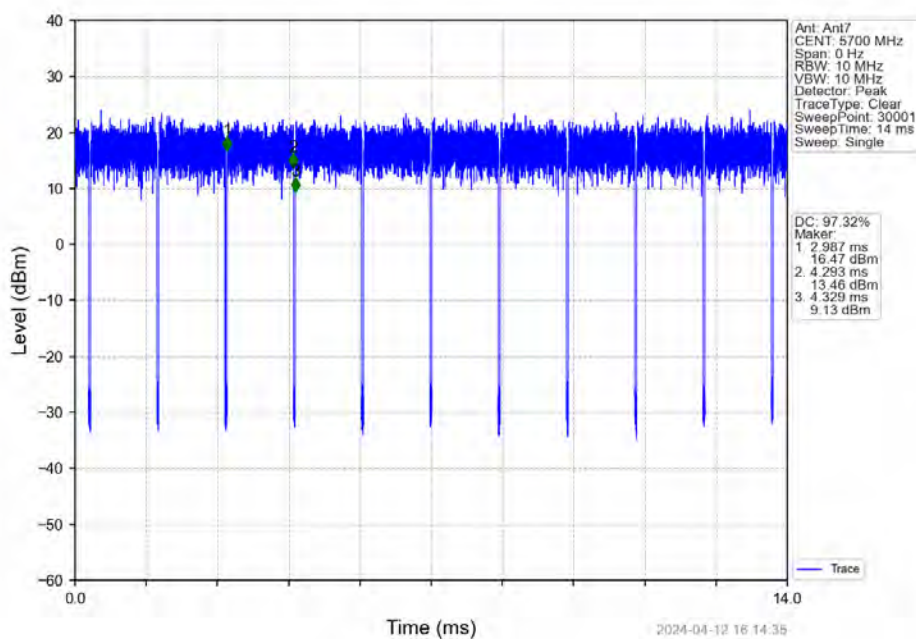
802.11ac(VHT20)_HCH_5700MHz_Ant7_NTNV
