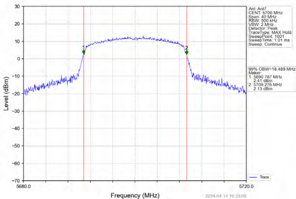
802.11ac(VHT20)_HCH_5700MHz_Ant7_NTNV
