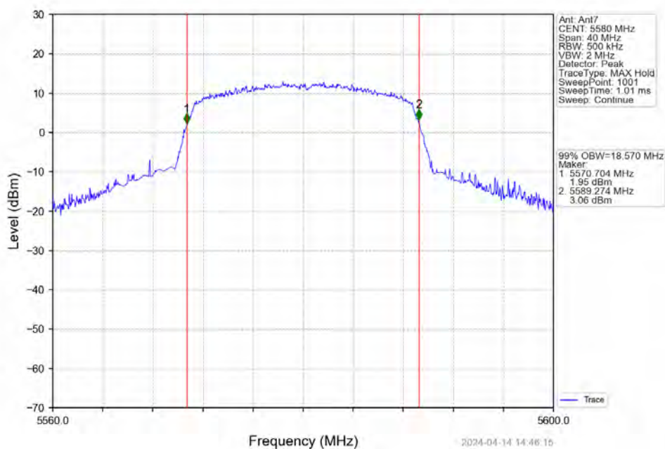
802.11n(HT20) MCH_5580MHz_Ant7_NTNV
