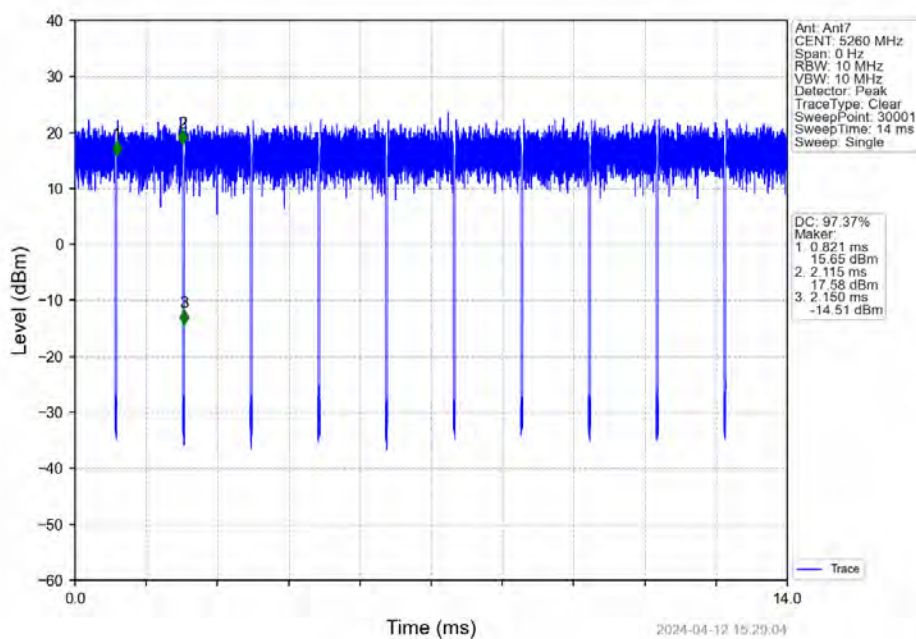
802.11n(HT20)_LCH_5260MHz_Ant7_NTNV
