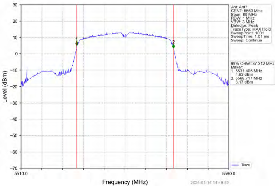
802.11n(HT40) MCH_5550MHz_Ant7_NTNV
