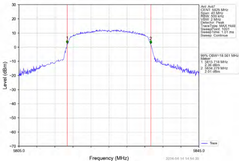
802.11n(HT20)_HCH_5825MHz_Ant7_NTNV
