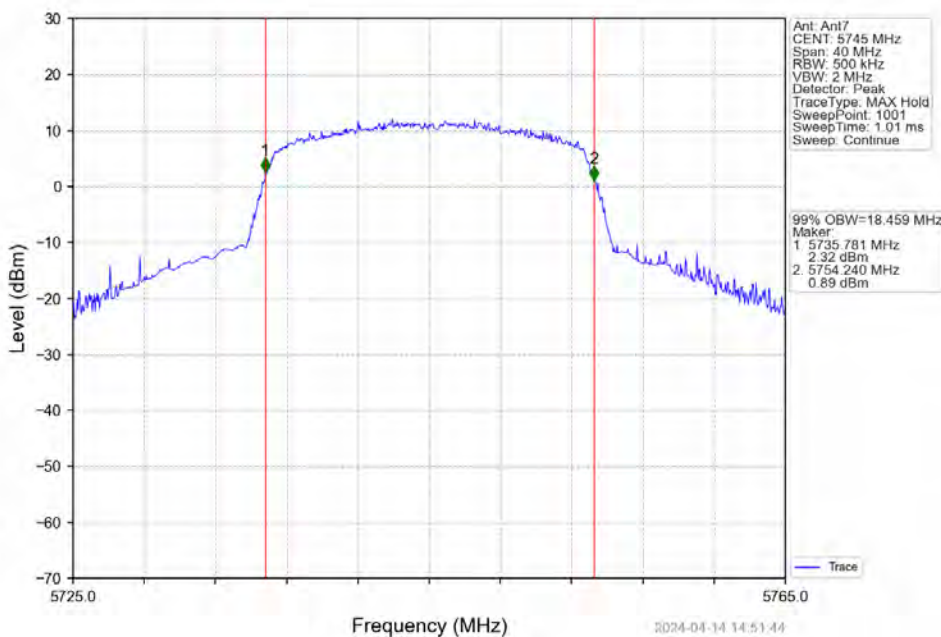
802.11n(HT20)_LCH_5745MHz_Ant7_NTNV
