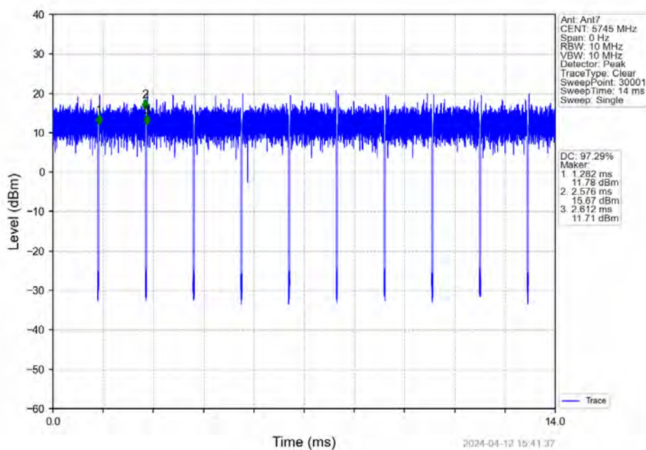
802.11n(HT20)_LCH_5745MHz_Ant7_NTNV
