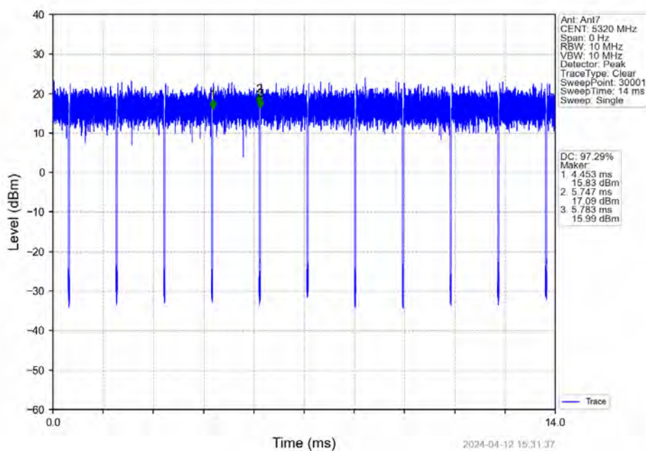
802.11n(HT20)_HCH_5320MHz_Ant7_NTNV
