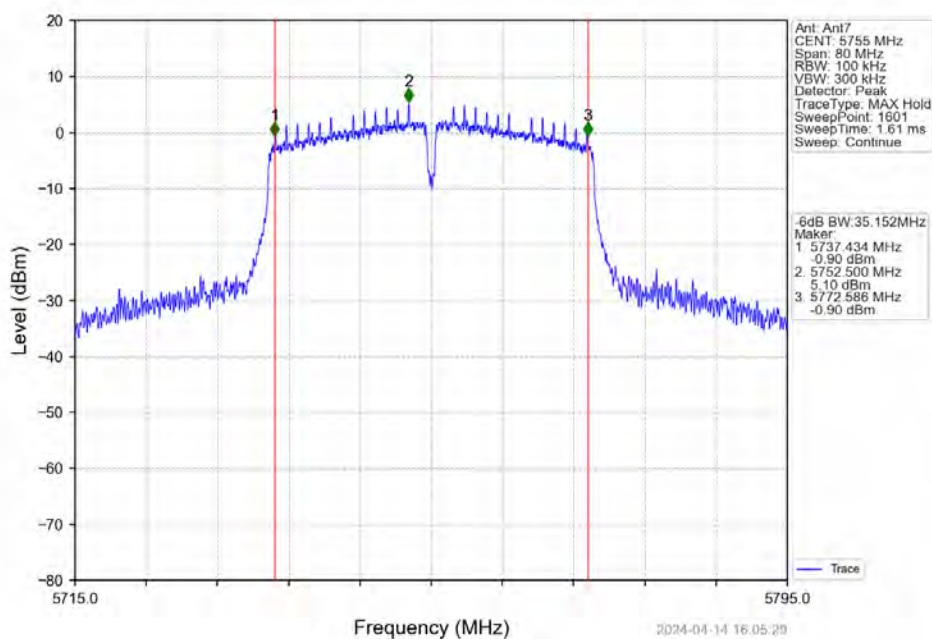
802.11ac(VHT40)_LCH_5755MHz_Ant7_NTNV
