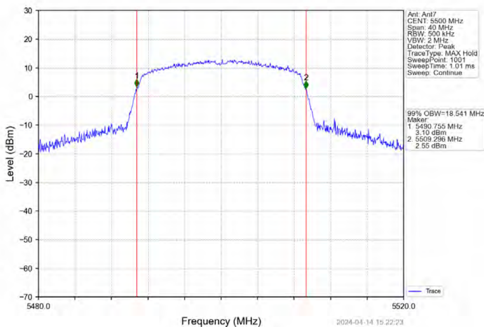
802.11ac(VHT20)_LCH_5500MHz_Ant7_NTNV
