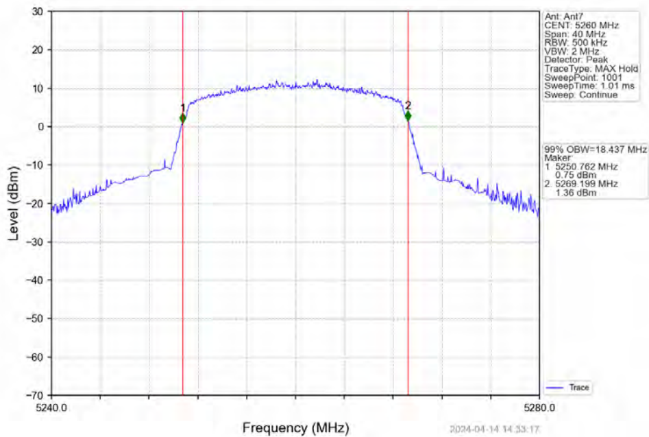
802.11n(HT20)_LCH_5260MHz_Ant7_NTNV
