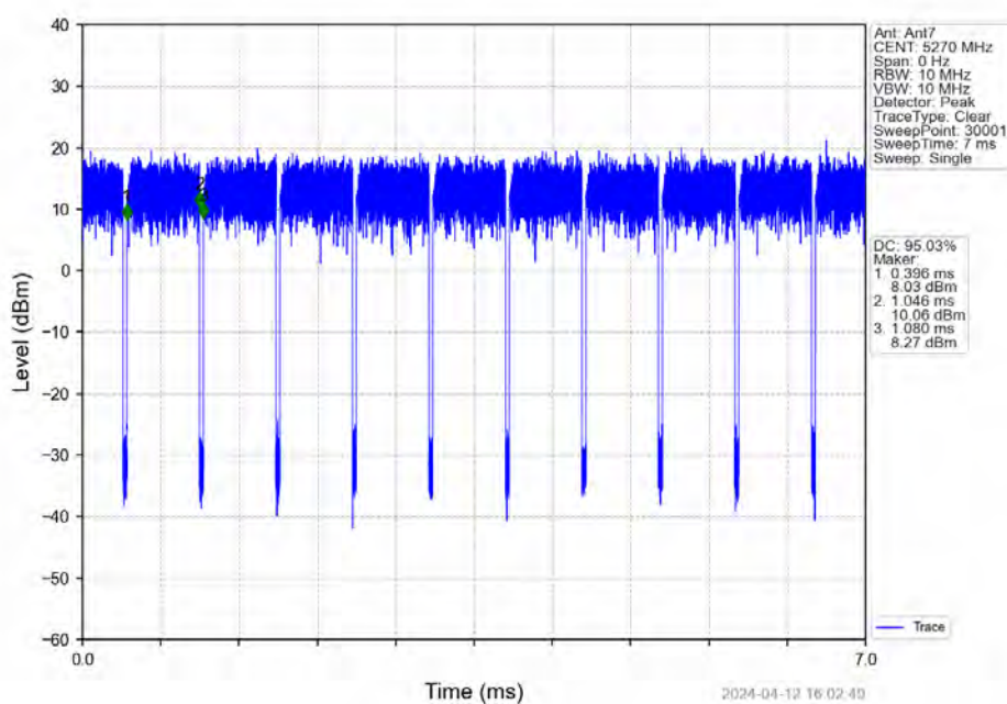
802.11ac(VHT40)_LCH_5270MHz_Ant7_NTNV
