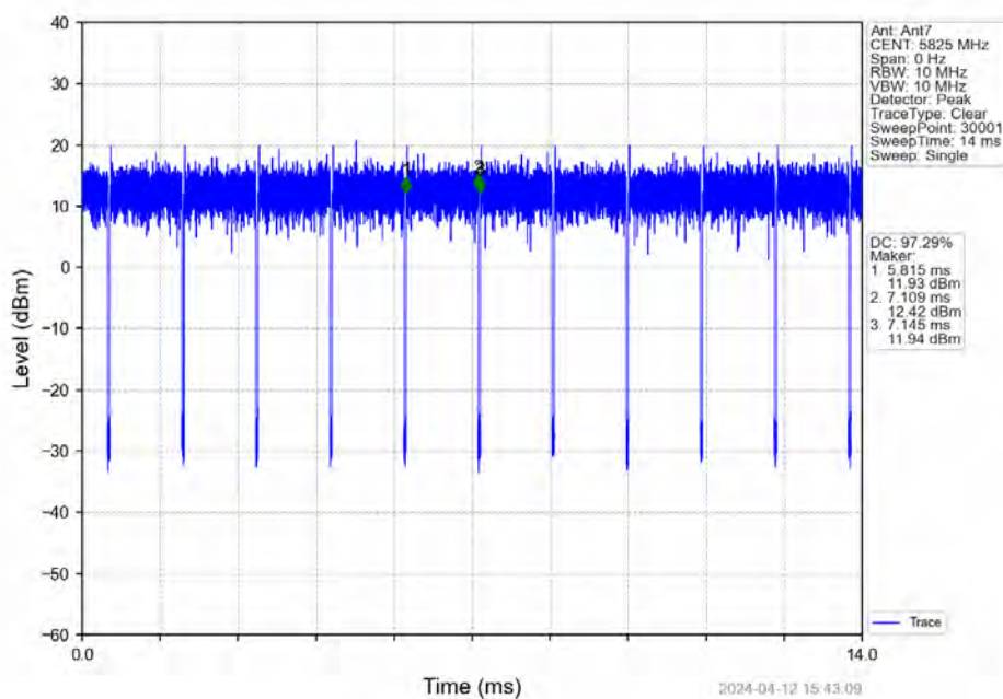
802.11n(HT20)_HCH_5825MHz_Ant7_NTNV
