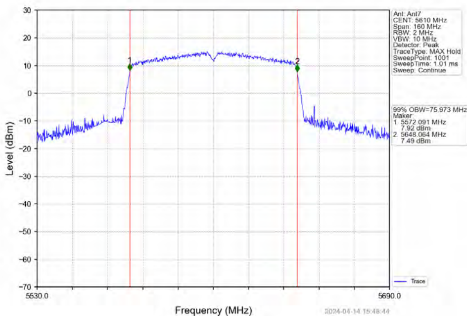
802.11ac(VHT80)_HCH_5610MHz_Ant7_NTNV
