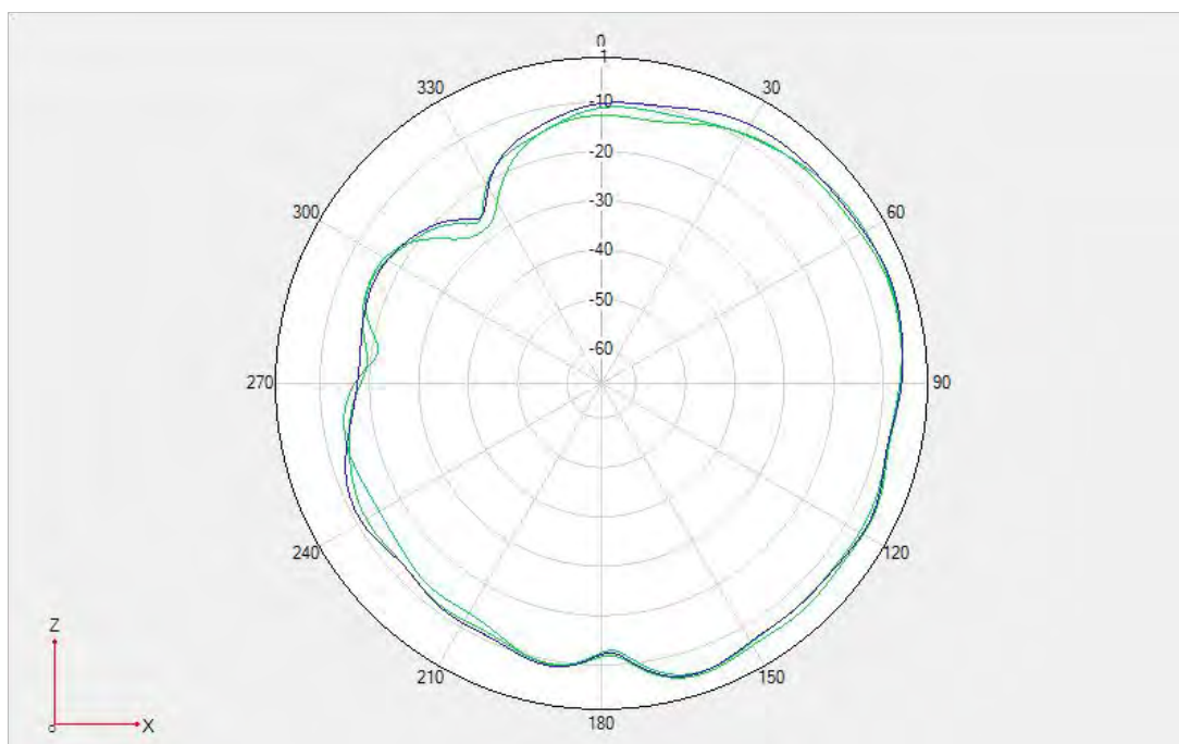
Unfold- NR n38DRX2 \Phi=0\text{deg}
