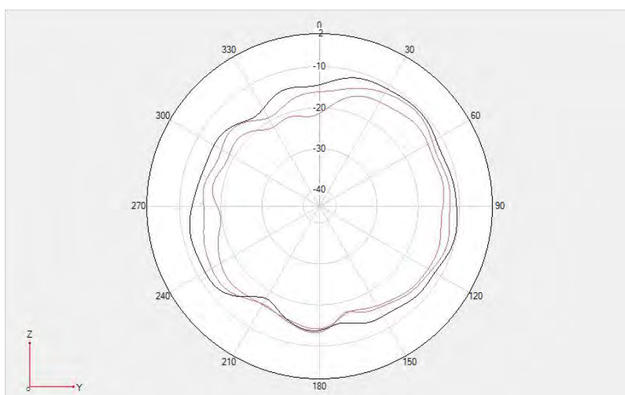
Fold- NR n3/N66 DRX \phi=0
