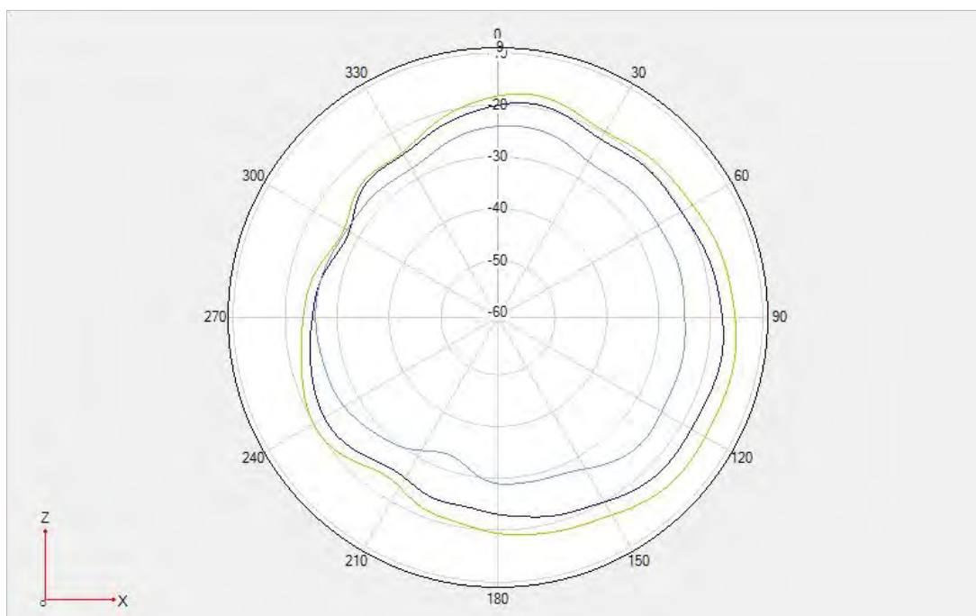
Fold- DPDT SWAP :GSM 850/WCDMA B5/LTE B5 \Phi = 0^\circ
