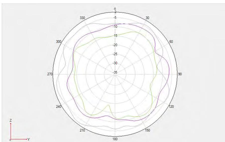
Fold- NR n77/78 DRX2 \phi=90
