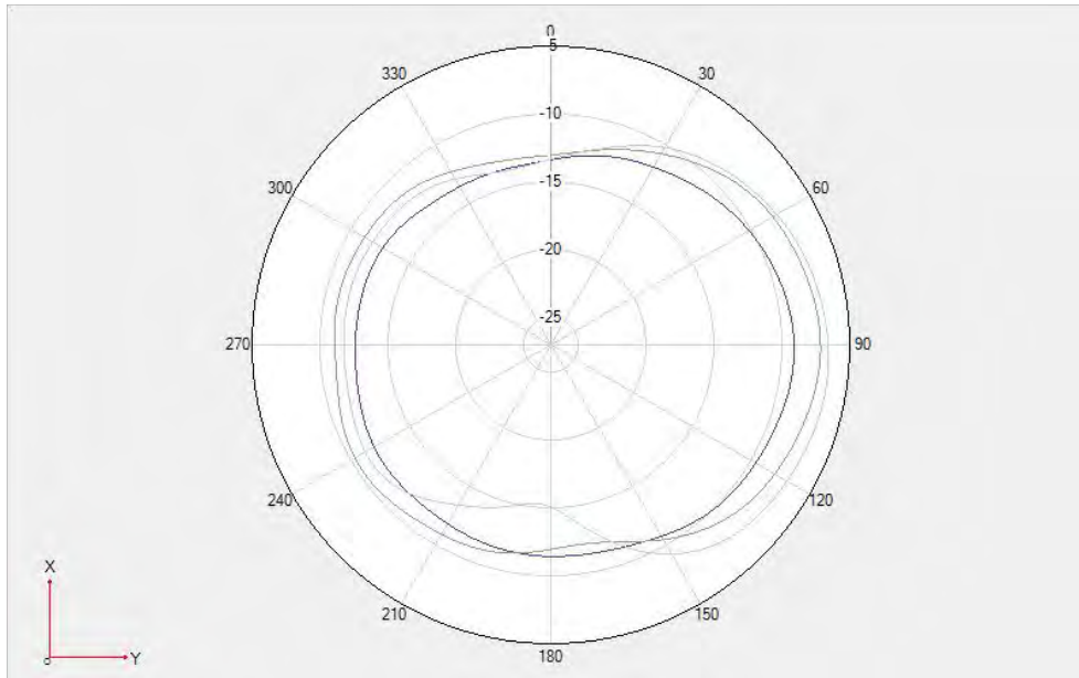
Fold-GSM 850/WCDMA B5/LTE B5/B20/N20 Theta=90deg
