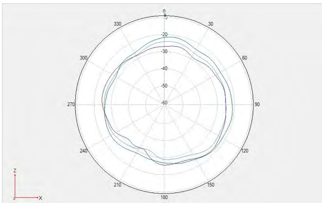
Fold- DPDT SWAPLITE B20/N20 Phi=0deg
