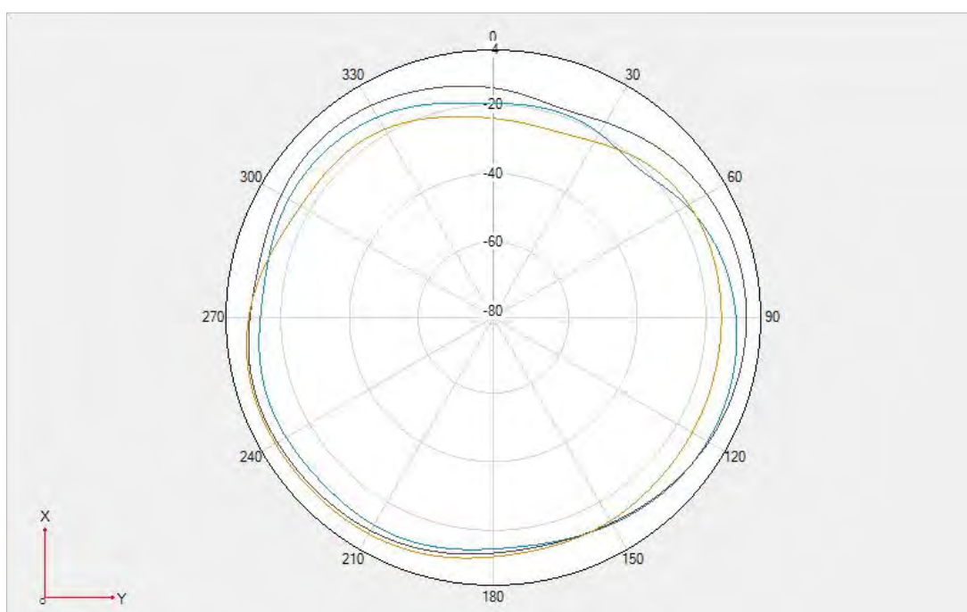
Fold- NR n40DRX2 \Theta=90^\circ
