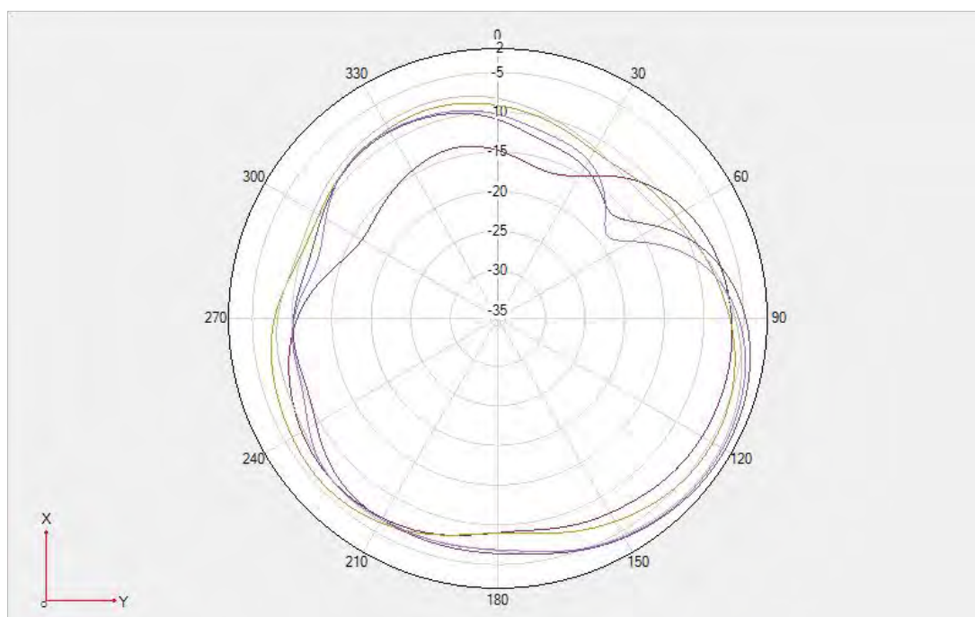
Fold- LTE B38/41 N38/41 Theta=90deg
