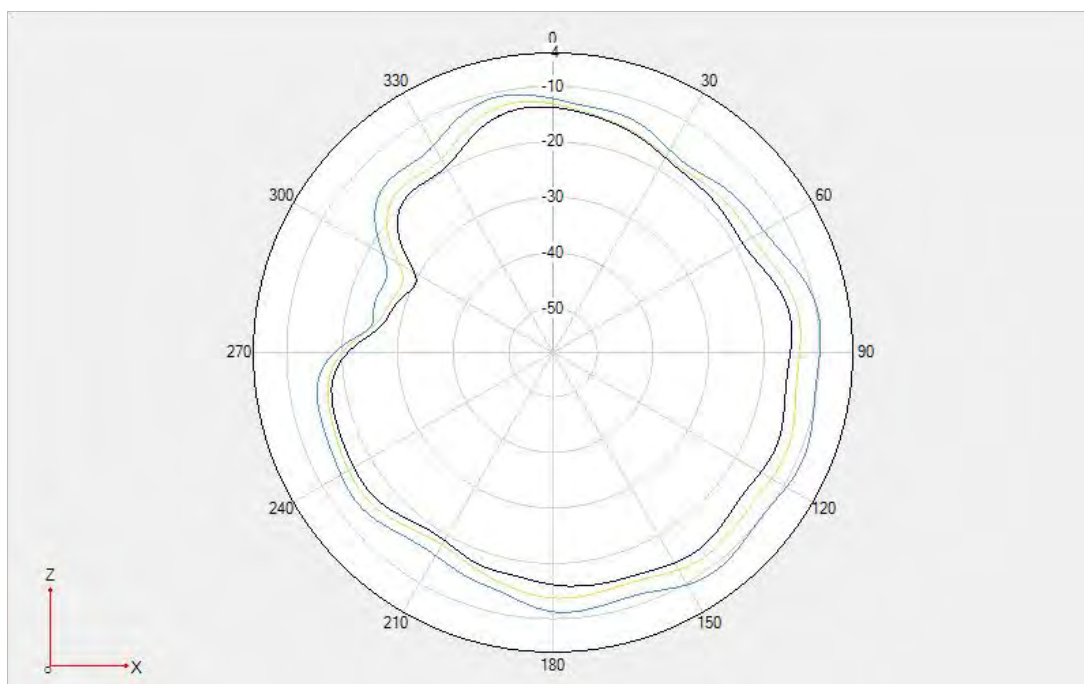
Unfold- DPDT SWAP :GSM 900/WCDMA B8/LTE B8 Phi=0deg
