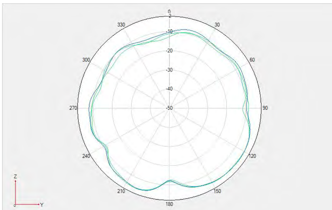
Unfold- NR n38DRX2 \Phi=90\text{deg}
