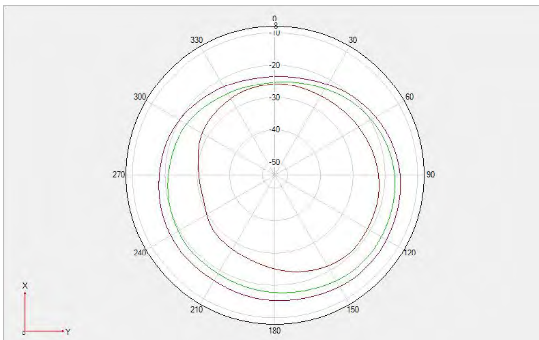
Fold- DPDT SWAP :GSM 850/WCDMA B5/LTE B5 Theta=90deg
