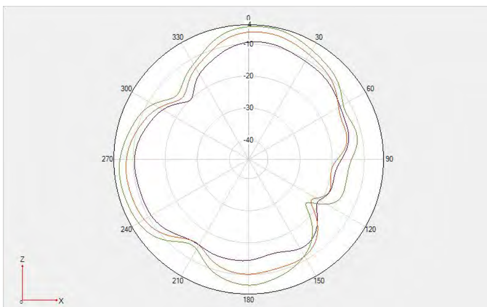
Unfold-GSM 850/WCDMA B5/LTE B5/B20/N20 \Phi=0^\circ
