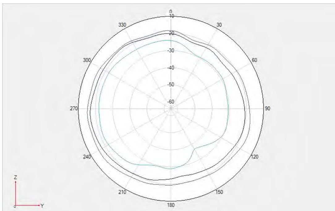
Fold- DPDT SWAP :GSM 850/WCDMA B5/LTE B5 \Phi = 90^\circ
