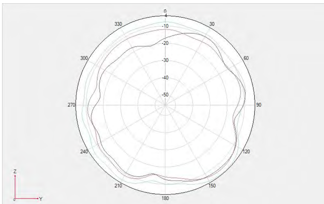
Fold- NR n40DRX2 \Phi=90^\circ
