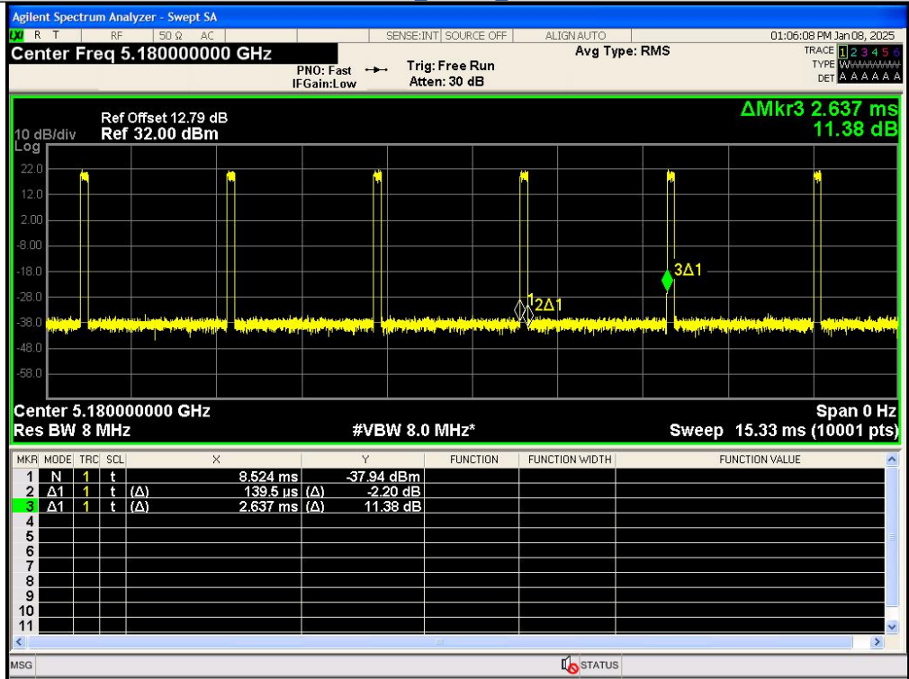
IEEE 802.11ac_20MHz_Channel 36
