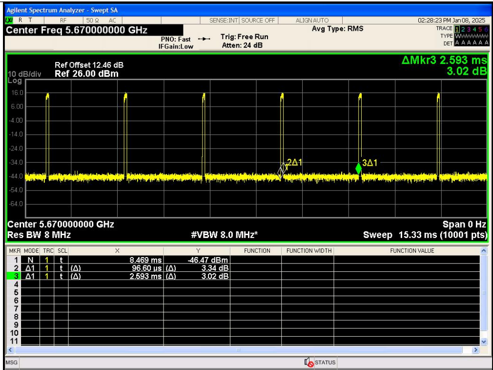
IEEE 802.11n_40MHz_Channel 134
