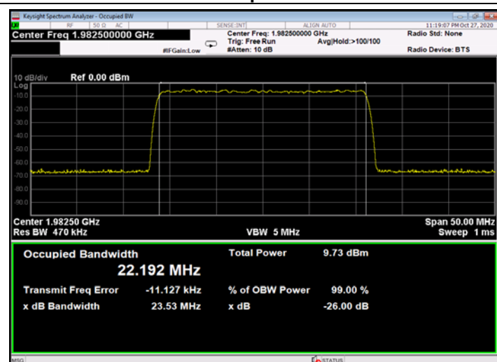
Figure 512: QPSK 25MHz B.W.; 1982.5MHz, 60kHz - Input
