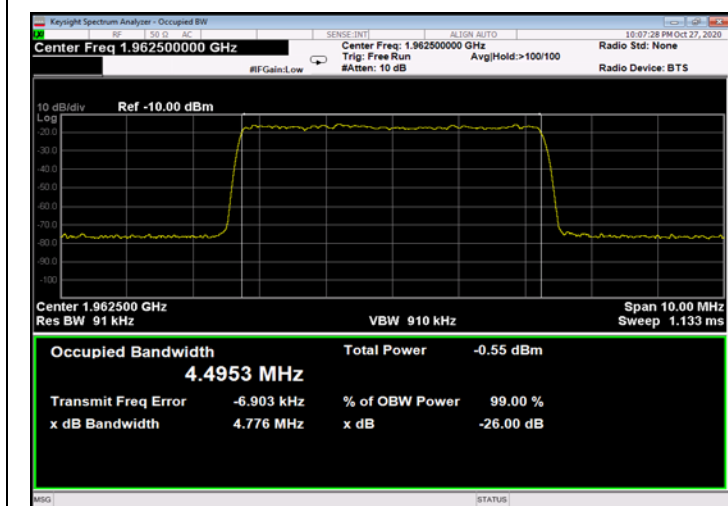
Figure 473: QPSK 5MHz B.W.; 1962.5MHz, 15kHz - Input
