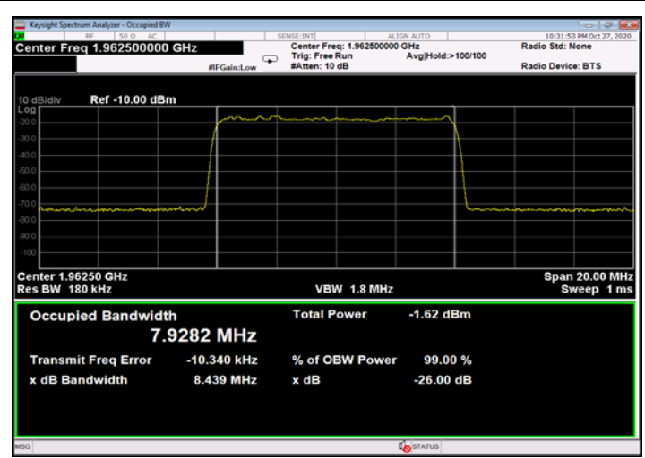
Figure 482: QPSK 10MHz B.W.; 1962.5MHz, 60kHz - Input
