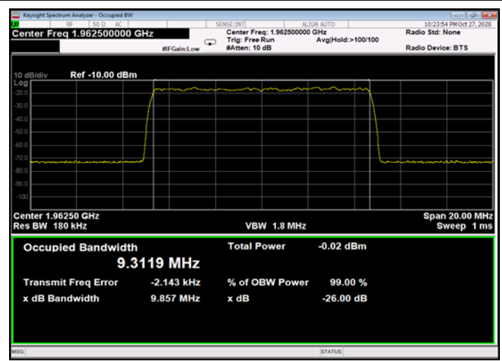
Figure 480: QPSK 10MHz B.W.; 1962.5MHz, 15kHz - Input
