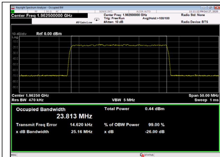
Figure 507: QPSK 25MHz B.W.; 1962.5MHz, 15kHz - Input
