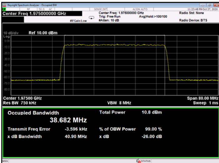
Figure 519: QPSK 40MHz B.W.; 1975.0MHz, 15kHz - Input
