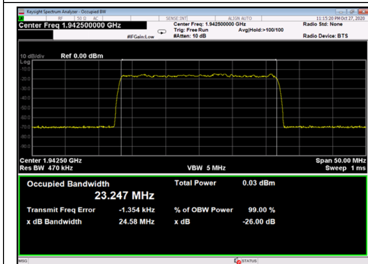
Figure 505: QPSK 25MHz B.W.; 1942.5MHz, 30kHz - Input
