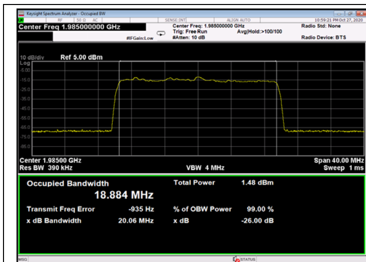
Figure 501: QPSK 20MHz B.W.; 1985.0MHz, 15kHz - Input
