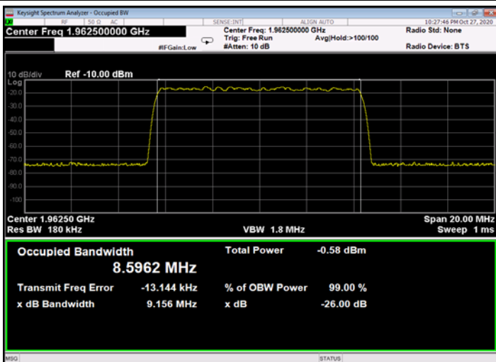
Figure 481: QPSK 10MHz B.W.; 1962.5MHz, 30kHz - Input
