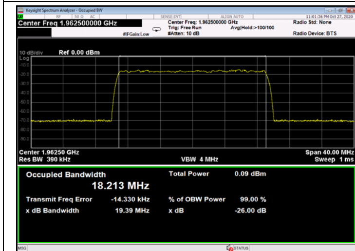
Figure 499: QPSK 20MHz B.W.; 1962.5MHz, 30kHz - Input
