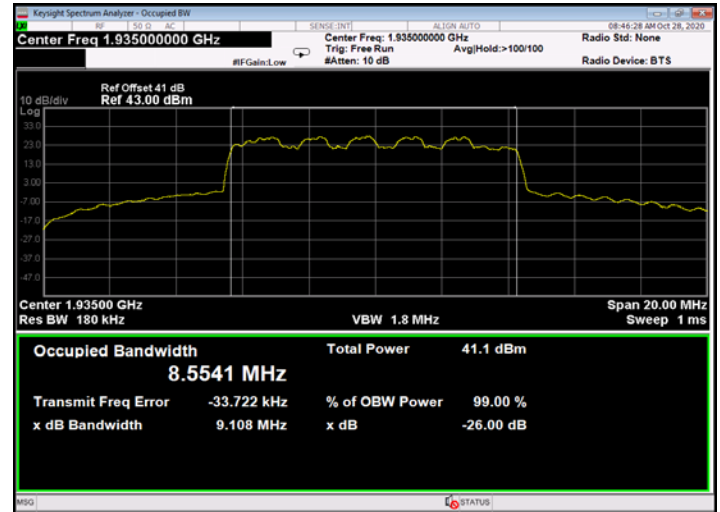
Figure 544: 16QAM 10MHz B.W.; 1935.0MHz, 30kHz - Output
