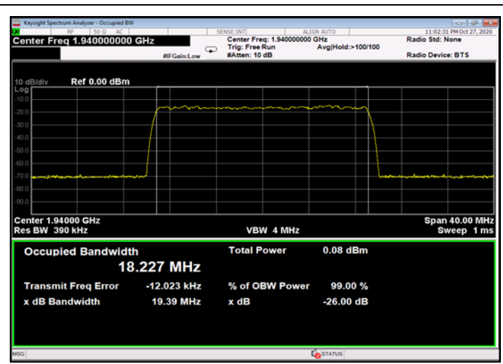
Figure 496: QPSK 20MHz B.W.; 1940.0MHz, 30kHz - Input
