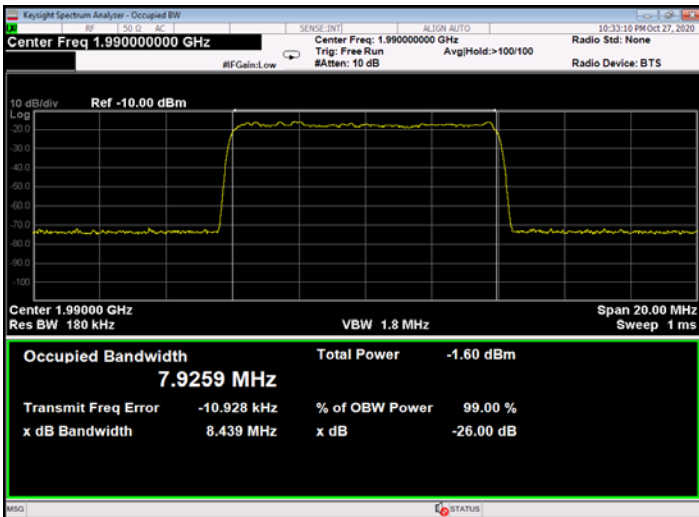
Figure 485: QPSK 10MHz B.W.; 1990.0MHz, 60kHz - Input
