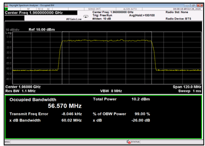
Figure 466: 256QAM 60MHz B.W.; 1960.0MHz, 60kHz - Input
