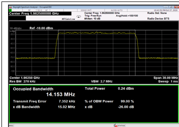
Figure 489: QPSK 15MHz B.W.; 1962.5MHz, 15kHz - Input
