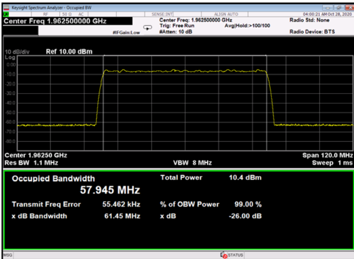
Figure 467: 256QAM 60MHz B.W.; 1962.5MHz, 30kHz - Input
