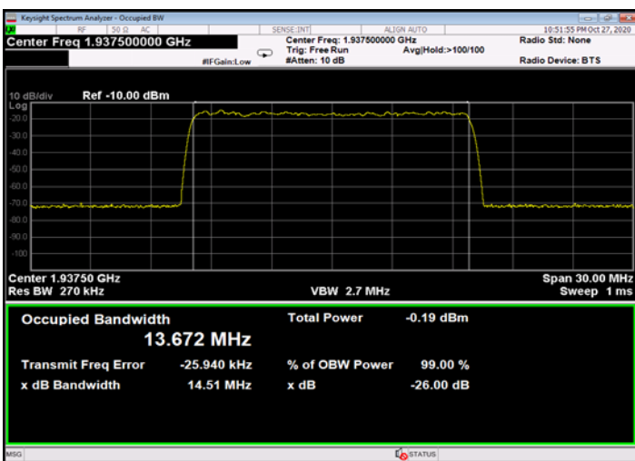
Figure 487: QPSK 15MHz B.W.; 1937.5MHz, 30kHz - Input
