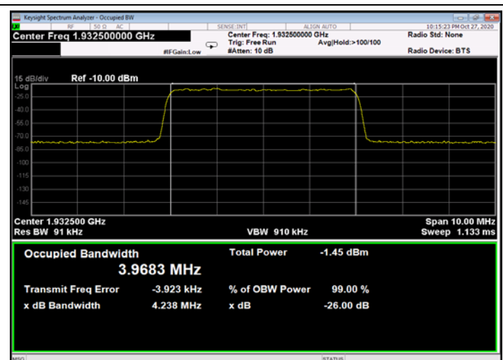
Figure 472: QPSK 5MHz B.W.; 1932.5MHz, 30kHz - Input
