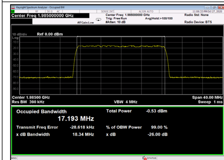
Figure 503: QPSK 20MHz B.W.; 1985.0MHz, 60kHz - Input
