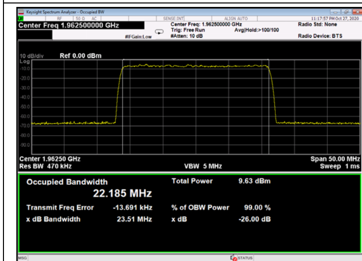
Figure 509: QPSK 25MHz B.W.; 1962.5MHz, 60kHz - Input
