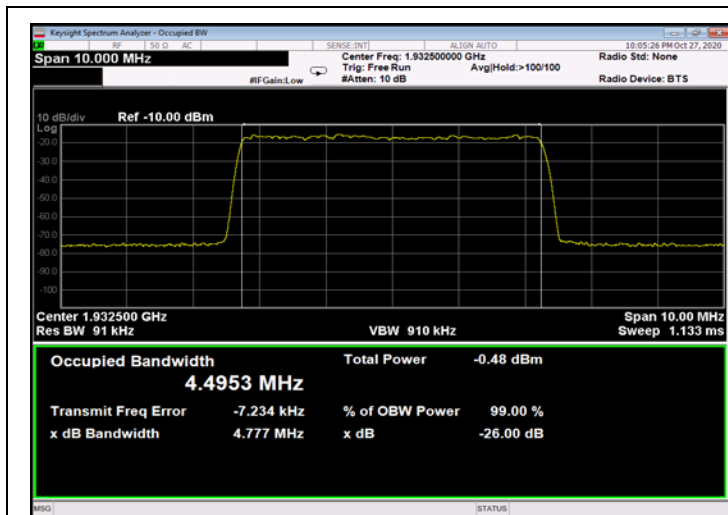
Figure 471: QPSK 5MHz B.W.; 1932.5MHz, 15kHz - Input
