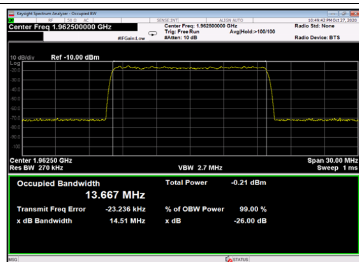
Figure 490: QPSK 15MHz B.W.; 1962.5MHz, 30kHz - Input
