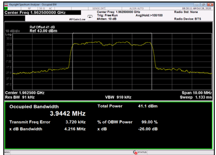
Figure 540: 16QAM 5MHz B.W.; 1962.5MHz, 30kHz - Output
