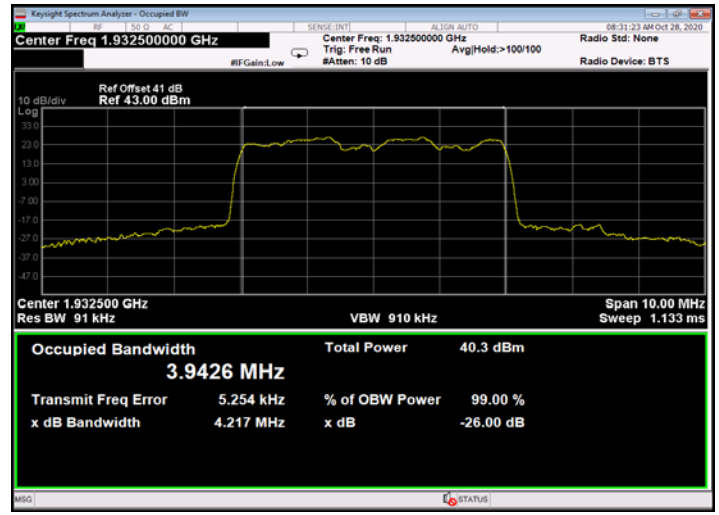
Figure 538: 16QAM 5MHz B.W.; 1932.5MHz, 30kHz - Output
