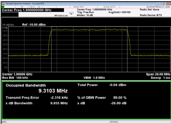
Figure 483: QPSK 10MHz B.W.; 1990.0MHz, 15kHz - Input
