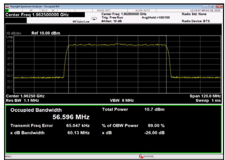
Figure 534: QPSK 60MHz B.W.; 1962.5MHz, 60kHz - Input
