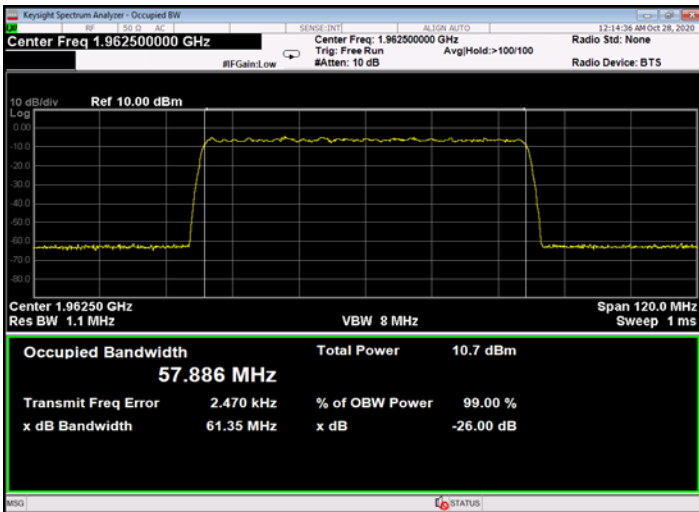
Figure 533: QPSK 60MHz B.W.; 1962.5MHz, 30kHz - Input
