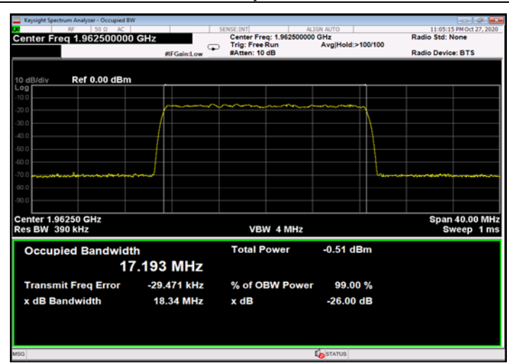
Figure 500: QPSK 20MHz B.W.; 1962.5MHz, 60kHz - Input
