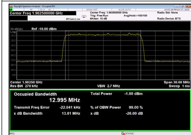
Figure 491: QPSK 15MHz B.W.; 1962.5MHz, 60kHz - Input
