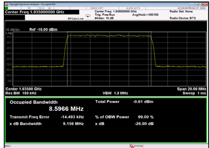
Figure 478: QPSK 10MHz B.W.; 1935.0MHz, 30kHz - Input
