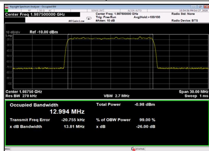
Figure 494: QPSK 15MHz B.W.; 1987.5MHz, 60kHz - Input
