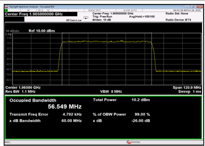
Figure 470: 256QAM 60MHz B.W.; 1965.0MHz, 60kHz - Input
