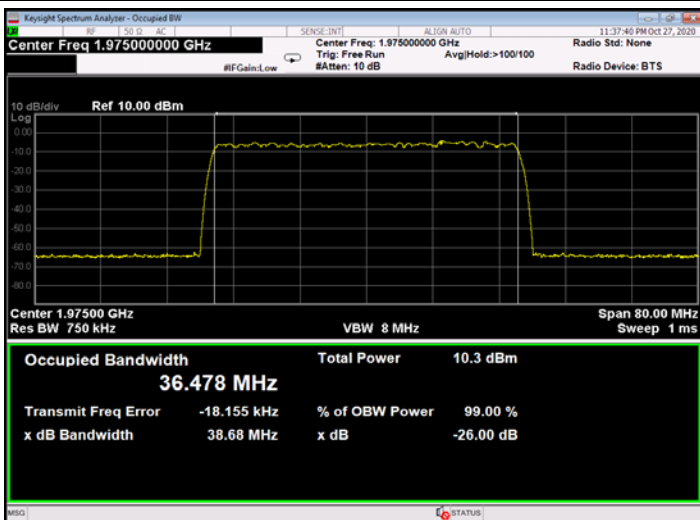
Figure 521: QPSK 40MHz B.W.; 1975.0MHz, 60kHz - Input
