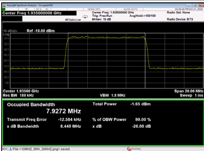
Figure 479: QPSK 10MHz B.W.; 1935.0MHz, 60kHz - Input
