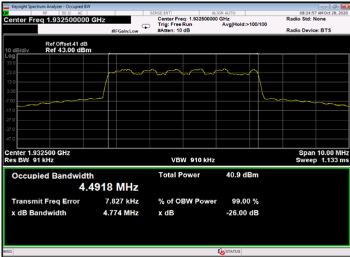
Figure 537: 16QAM 5MHz B.W.; 1932.5MHz, 15kHz - Output
