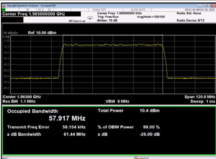
Figure 469: 256QAM 60MHz B.W.; 1965.0MHz, 30kHz - Input
