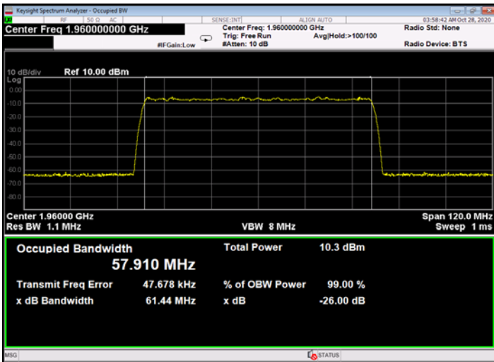
Figure 465: 256QAM 60MHz B.W.; 1960.0MHz, 30kHz - Input
