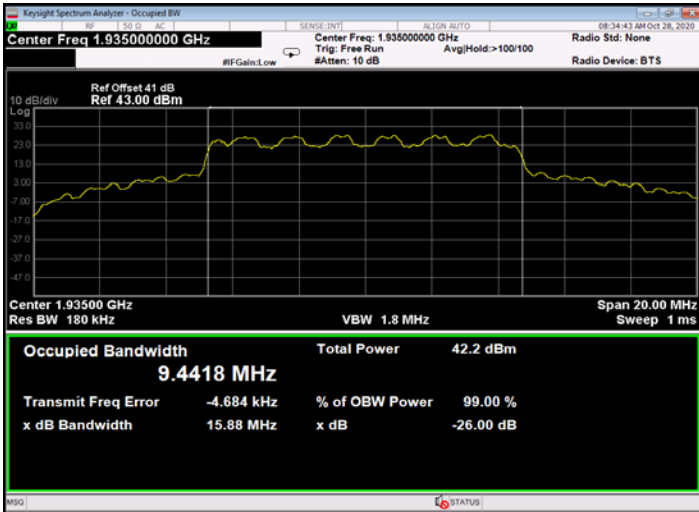
Figure 543: 16QAM 10MHz B.W.; 1935.00MHz, 15kHz - Output
