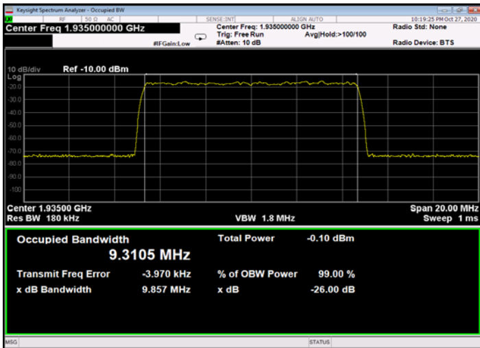
Figure 477: QPSK 10MHz B.W.; 1935.00MHz, 15kHz - Input
