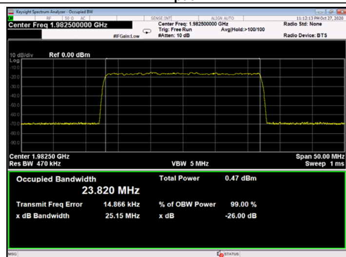
Figure 510: QPSK 25MHz B.W.; 1982.5MHz, 15kHz - Input
