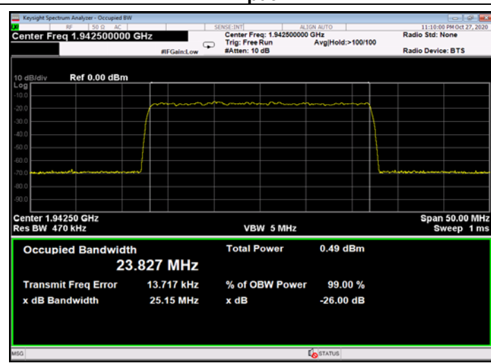
Figure 504: QPSK 25MHz B.W.; 1942.5MHz, 15kHz - Input
