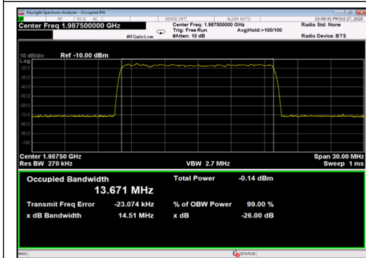
Figure 493: QPSK 15MHz B.W.; 1987.5MHz, 30kHz - Input
