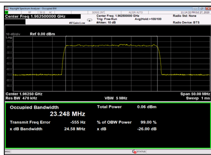
Figure 508: QPSK 25MHz B.W.; 1962.5MHz, 30kHz - Input
