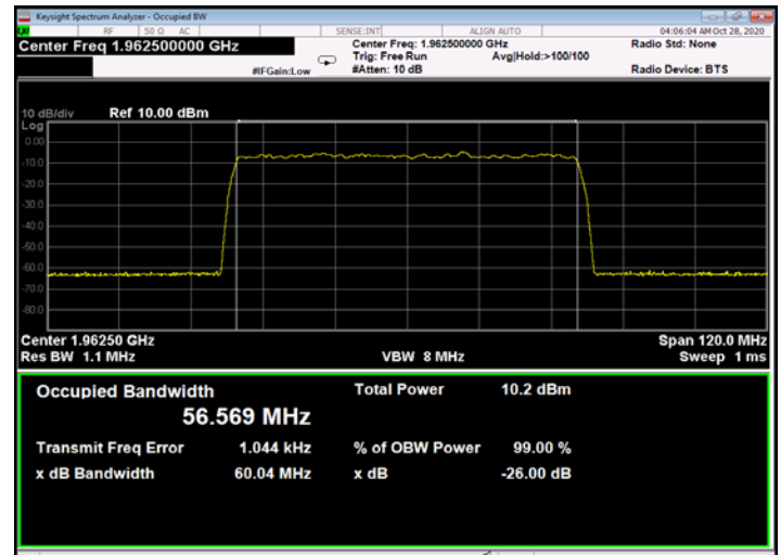
Figure 468: 256QAM 60MHz B.W.; 1962.5MHz, 60kHz - Input
