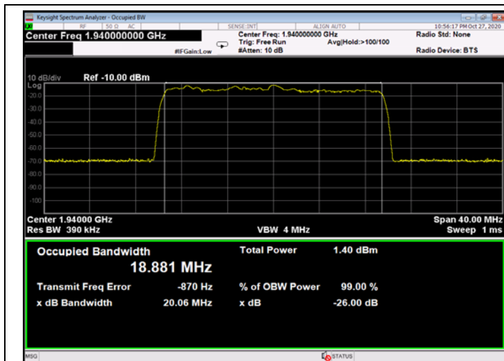
Figure 495: QPSK 20MHz B.W.; 1940.0MHz, 15kHz - Input
