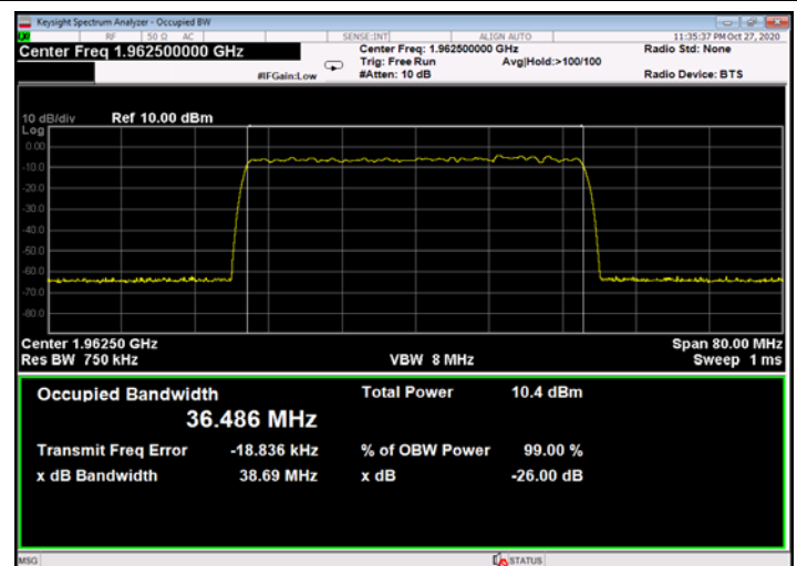
Figure 518: QPSK 40MHz B.W.; 1962.5MHz, 60kHz - Input
