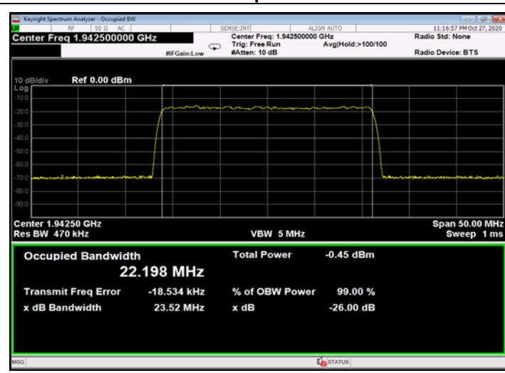
Figure 506: QPSK 25MHz B.W.; 1942.5MHz, 60kHz - Input
