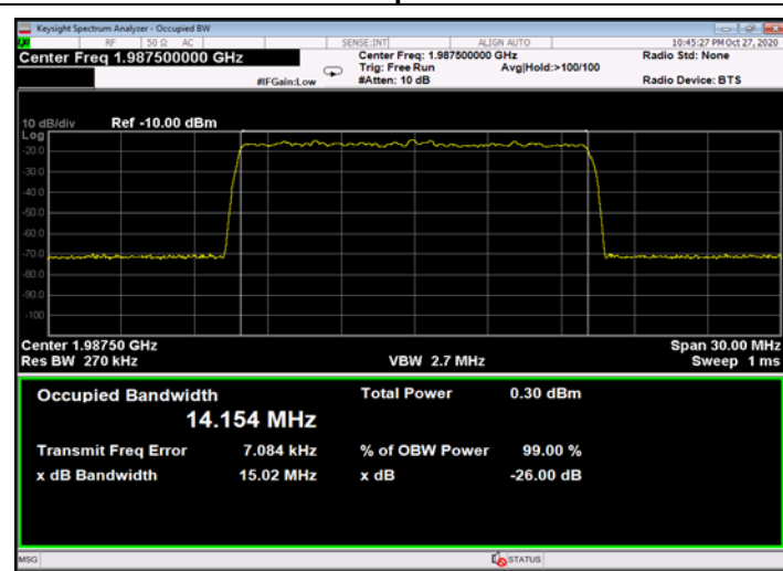
Figure 492: QPSK 15MHz B.W.; 1987.5MHz, 15kHz - Input
