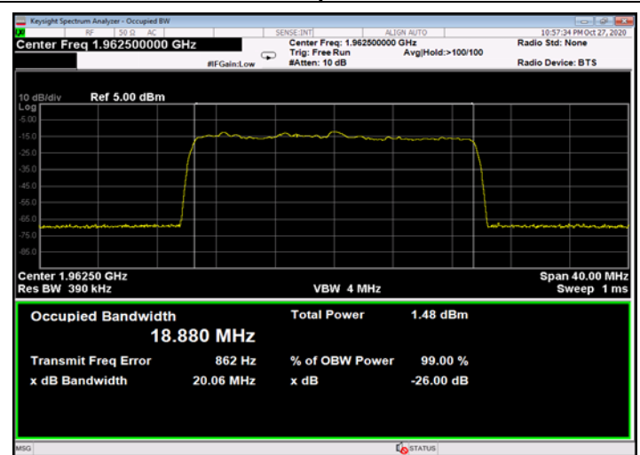
Figure 498: QPSK 20MHz B.W.; 1962.5MHz, 15kHz - Input
