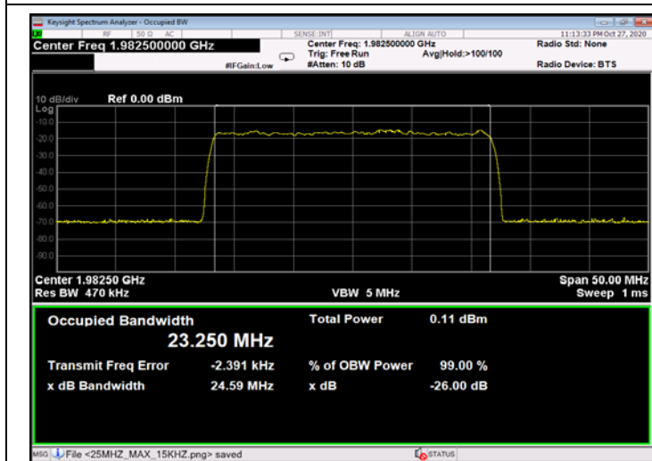
Figure 511: QPSK 25MHz B.W.; 1982.5MHz, 30kHz - Input
