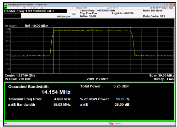
Figure 486: QPSK 15MHz B.W.; 1937.5MHz, 15kHz - Input
