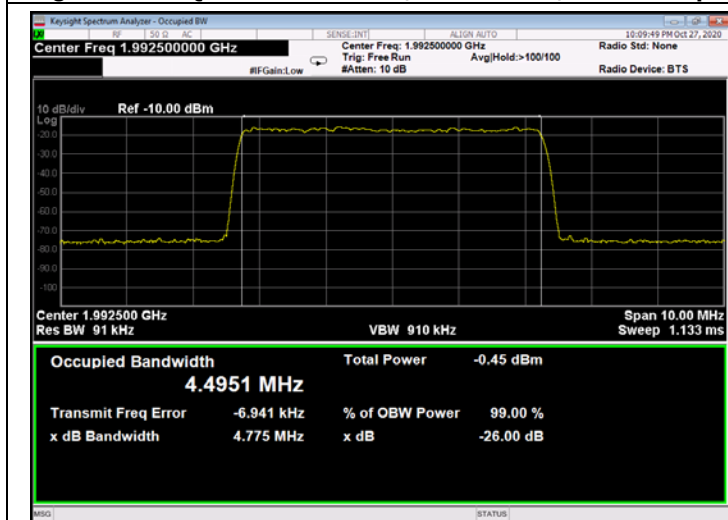
Figure 475: QPSK 5MHz B.W.; 1992.5MHz, 15kHz - Input
