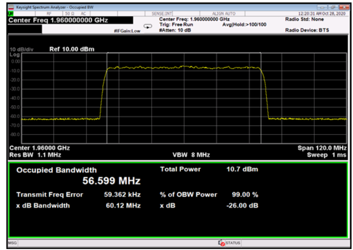
Figure 532: QPSK 60MHz B.W.; 1960.0MHz, 60kHz - Input
