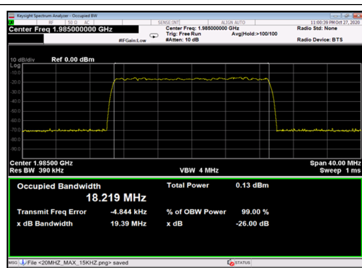
Figure 502: QPSK 20MHz B.W.; 1985.0MHz, 30kHz - Input
