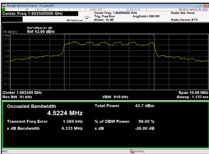
Figure 541: 16QAM 5MHz B.W.; 1992.5MHz, 15kHz - Output
