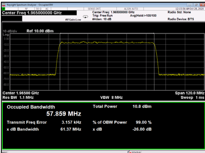
Figure 535: QPSK 60MHz B.W.; 1965.0MHz, 30kHz - Input
