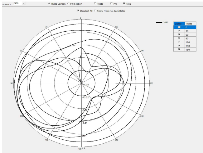
2400MHz
