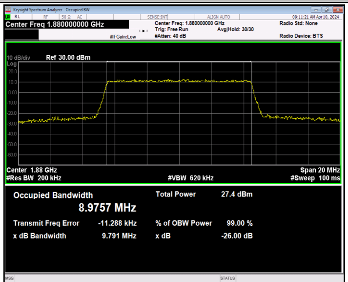
Band2-10MHz-16QAM-18900-50RB#0-PASS
