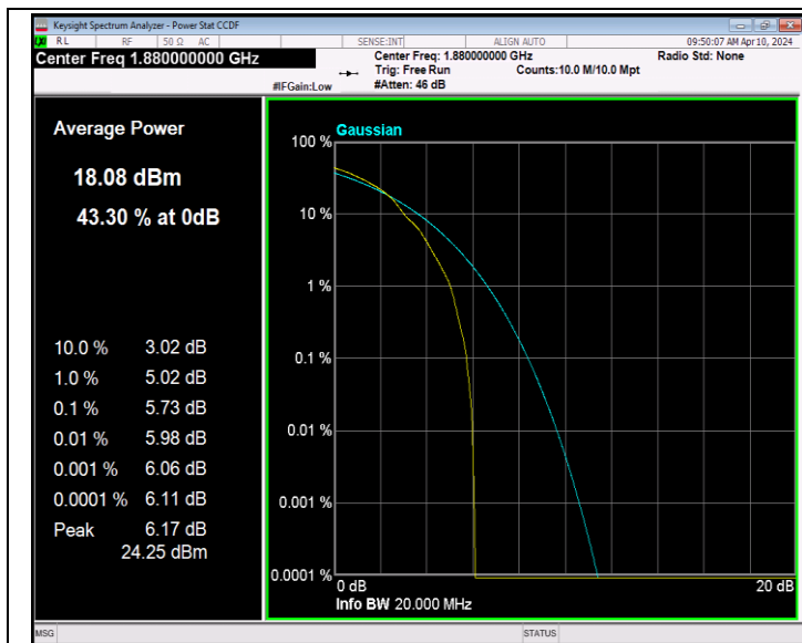
Band2-20MHz-64QAM-18900-1RB#0-PASS
