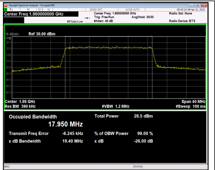
Band2-20MHz-QPSK-18700-100RB#0-PASS
