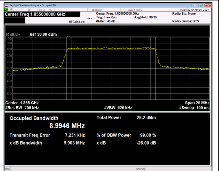
Band2-10MHz-QPSK-18650-50RB#0-PASS
