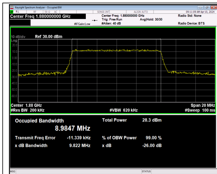
Band2-10MHz-QPSK-18900-50RB#0-PASS
