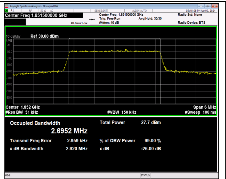
Band2-3MHz-QPSK-18615-15RB#0-PASS
