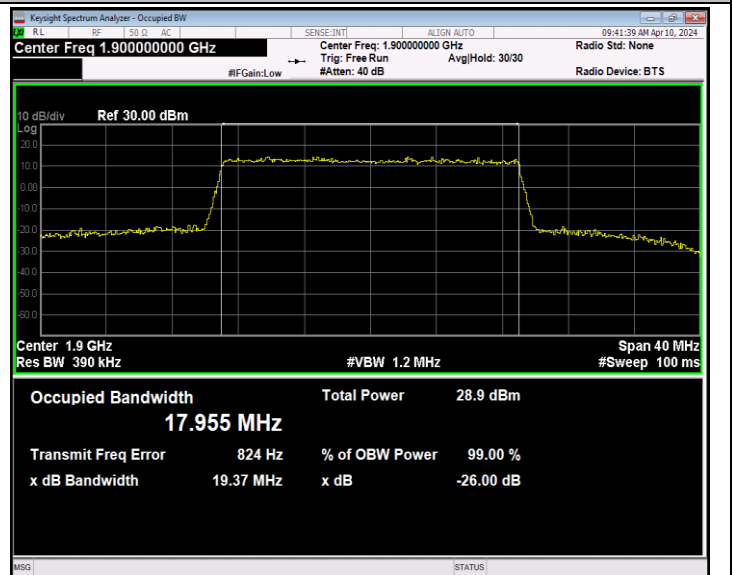
Band2-20MHz-QPSK-19100-100RB#0-PASS
