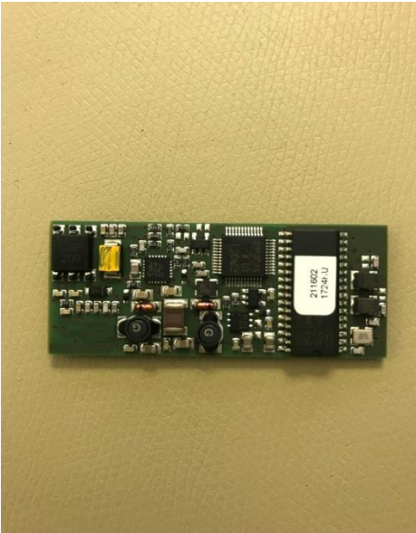
PCBA Top
