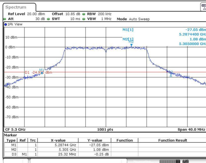
11A_Ant1_5300
