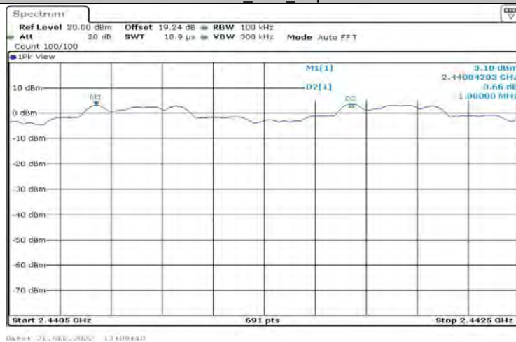
3DH1_Ant1_Hop
