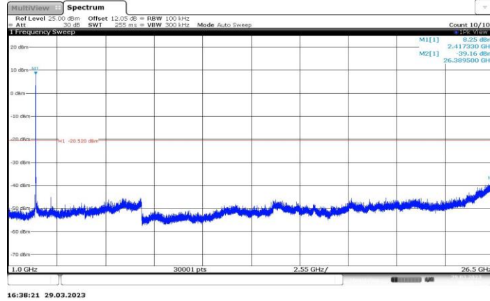
11B_Ant1_2417_1000~26500
