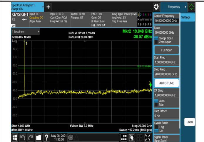
Band2-20MHz-16QAM-18700-1RB#0-Range2:1000~20
