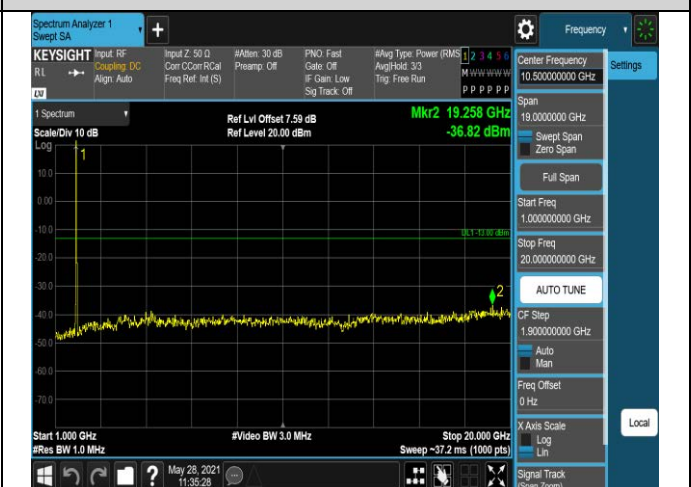
Band2-20MHz-QPSK-18900-1RB#0-Range2:1000~200
