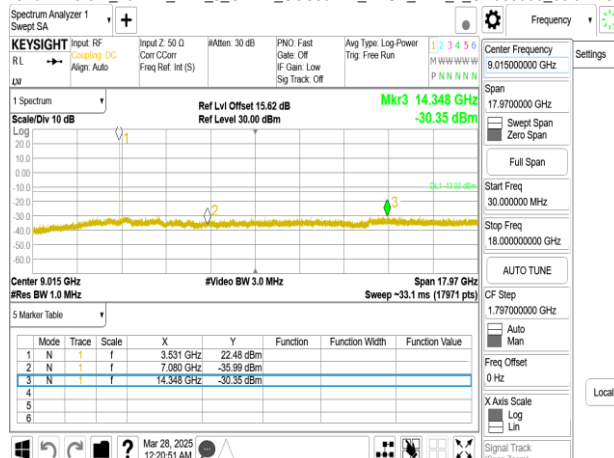
Band77-Part27_20MHz_DFT_s_OFDM_SCS30kHz_BPSK_RB1_1_CH636000upper 18G
