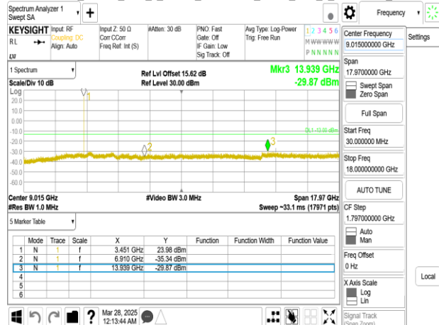
Band77-Part27_10MHz_DFT_s_OFDM_SCS30kHz_BPSK_RB1_1_CH630334upper 18G
