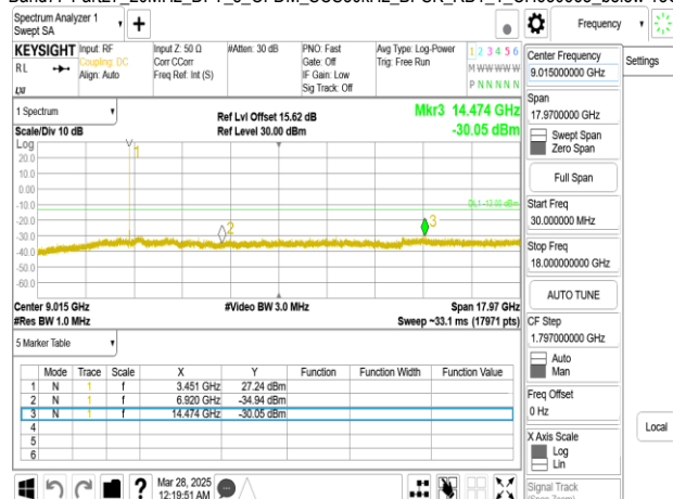
Band77-Part27_20MHz_DFT_s_OFDM_SCS30kHz_BPSK_RB1_1_CH630668upper 18G
