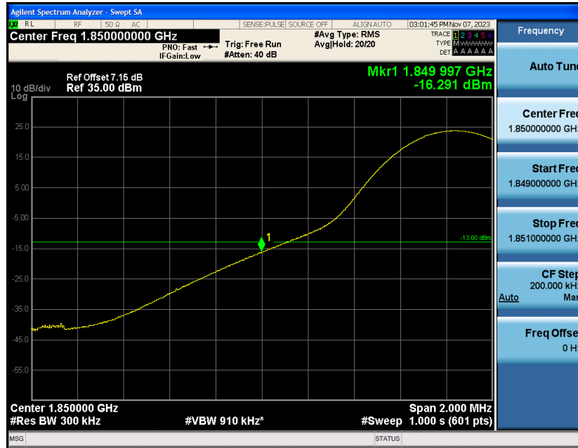
Band2-15MHz-QPSK-18675-1RB#74
