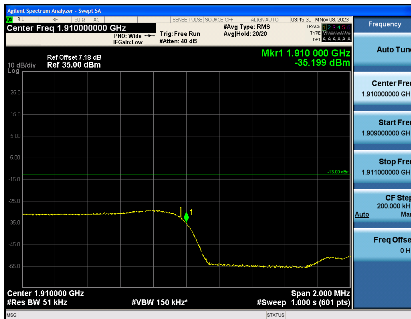
Band2-3MHz-QPSK-19185-1RB#14
