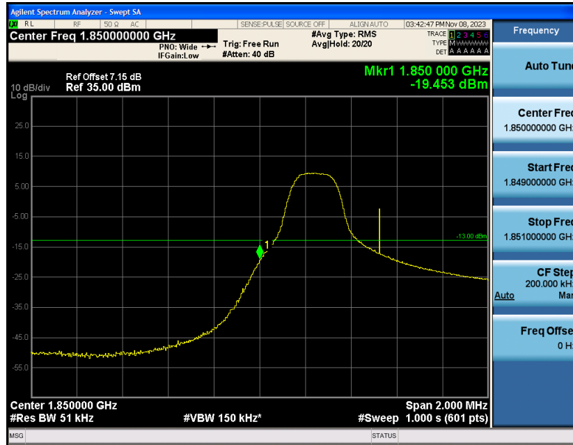
Band2-3MHz-QPSK-18615-1RB#14
