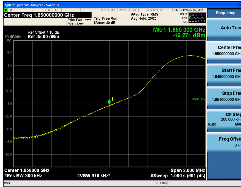
Band2-15MHz-16QAM-18675-1RB#74
