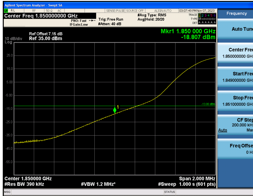
Band2-20MHz-QPSK-18700-1RB#99
