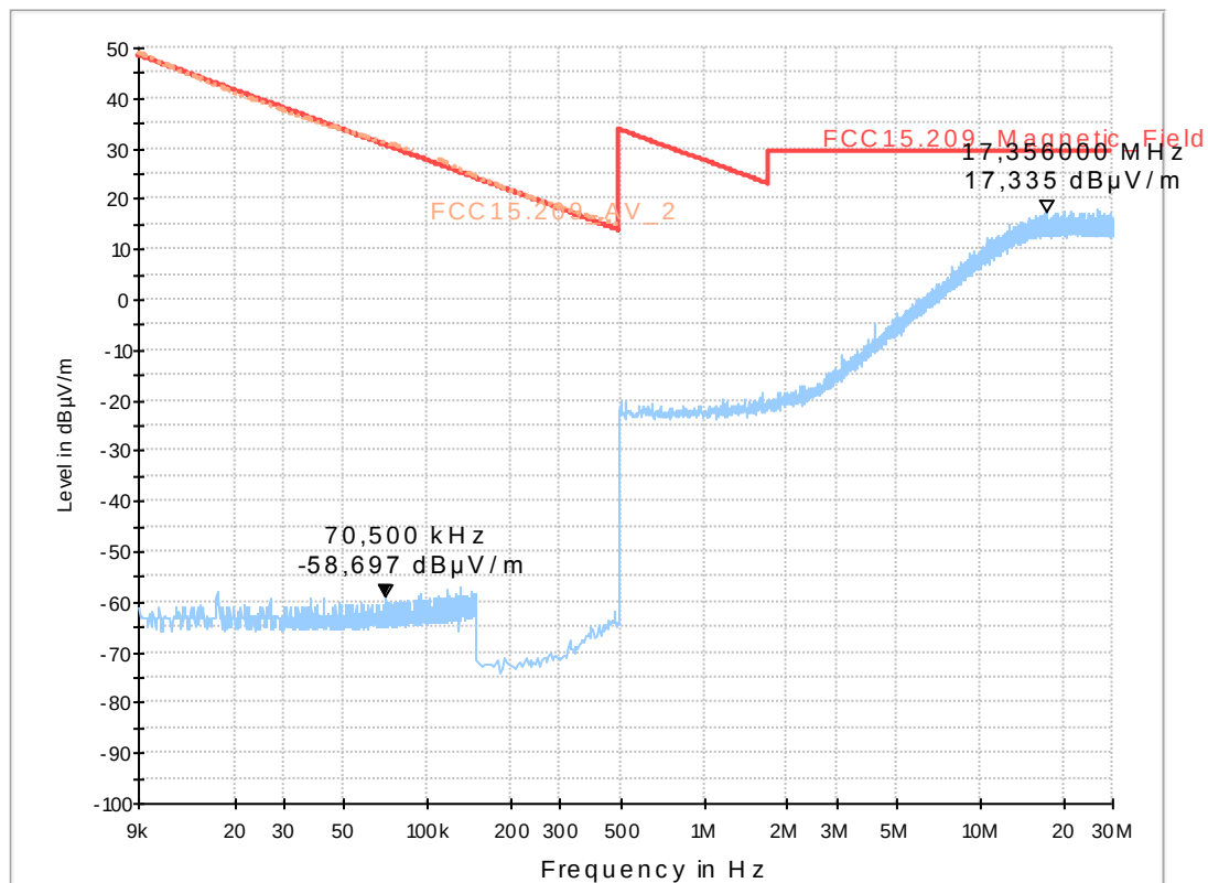
FCC15.209_magn hor+vert
