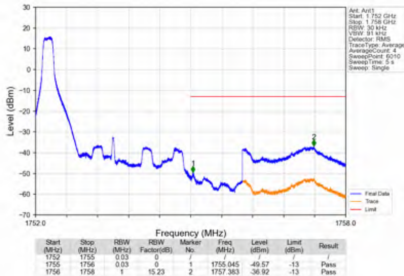
Band4_3MHz_QPSK_HCH_1753.5MHz_RB_1_14_NTNV
