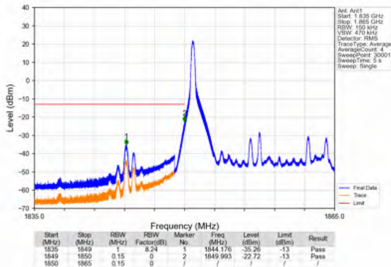
Band2_15MHz_QPSK_LCH_1857.5MHz_RB_1_0_NTNV
