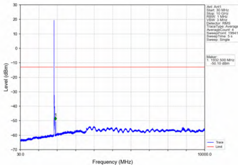
Band2 20MHz 256QAM LCH 1860MHz RB 1 0 NTNV
