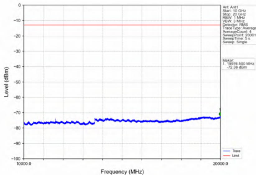
Band2_20MHz_256QAM_MCH_1880MHz_RB_1_0_NTNV
