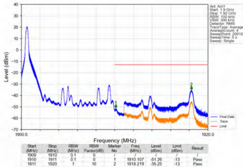
Band2_10MHz_QPSK_HCH_1905MHz_RB_1_49_NTNV
