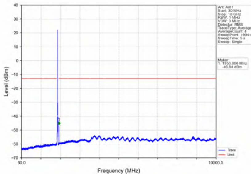
Band2_20MHz_64QAM_MCH_1880MHz_RB_1_0_NTNV
