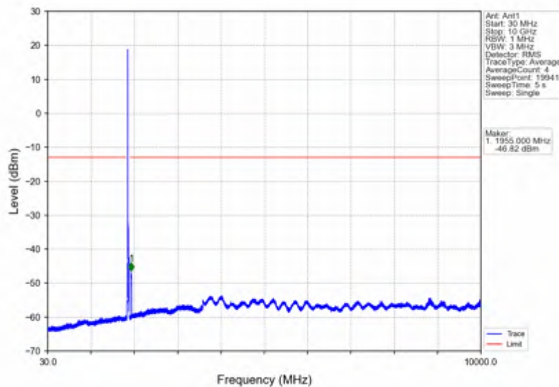
Band2_20MHz_256QAM_MCH_1880MHz_RB_1_0_NTNV
