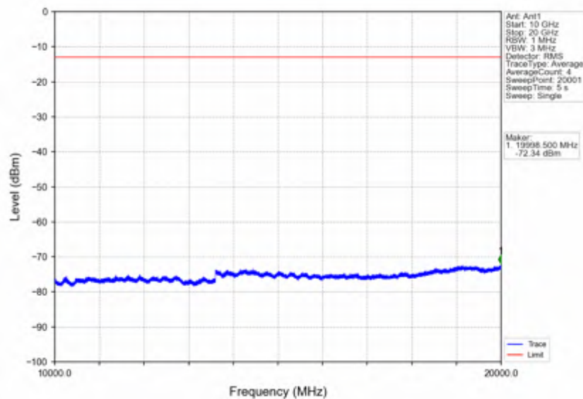
Band2 10MHz 64QAM LCH 1855MHz RB 50 0 NTNv
