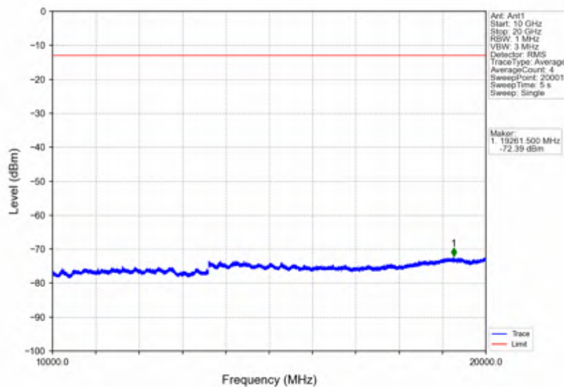
Band2_10MHz_16QAM_MCH_1880MHz_RB_1_0_NTNV
