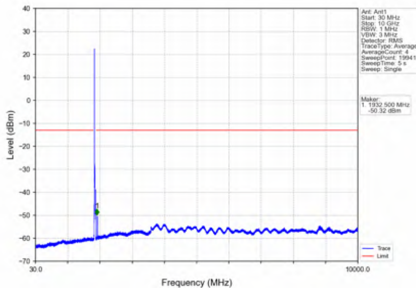
Band2_20MHz_16QAM_LCH_1860MHz_RB_1_0_NTNV
