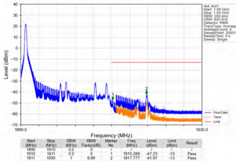
Band2_20MHz_16QAM_HCH_1900MHz_RB_1_99_NTNV
