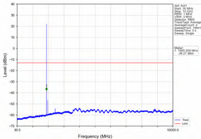
Band2_1.4MHz_QPSK_HCH_1909.3MHz_RB_1_0_NTNV
