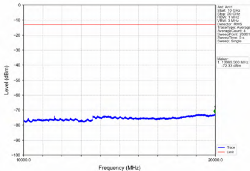
Band2 15MHz 16QAM LCH 1857.5MHz RB 75 0 NTNV
