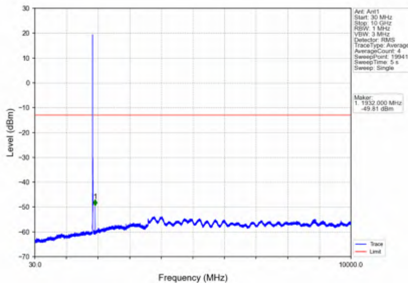
Band2 10MHz 256QAM LCH 1855MHz RB 1 0 NTNV
