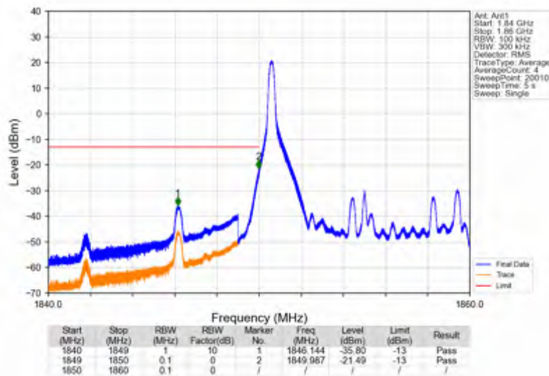
Band2_10MHz_16QAM_LCH_1855MHz_RB_50_0_NTNV
