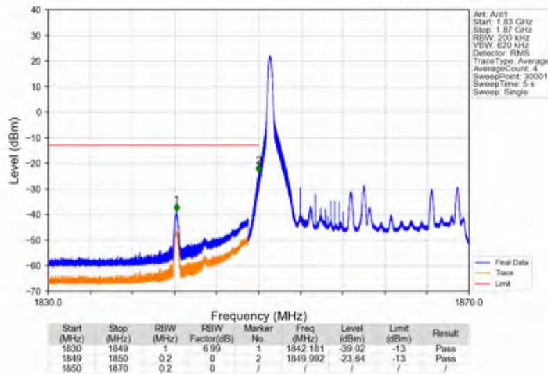
Band2 20MHz 64QAM LCH 1860MHz RB 1 0 NTNv
