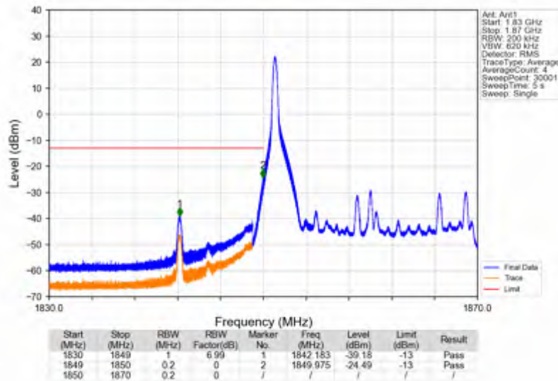
Band2 20MHz 64QAM LCH 1860MHz RB 100 0 NTNv
