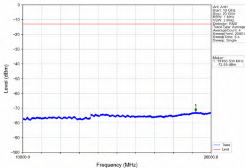
Band2_3MHz_QPSK_MCH_1880MHz_RB_1_0_NTNV
