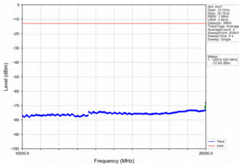
Band2_3MHz_256QAM_MCH_1880MHz_RB_1_0_NTNV
