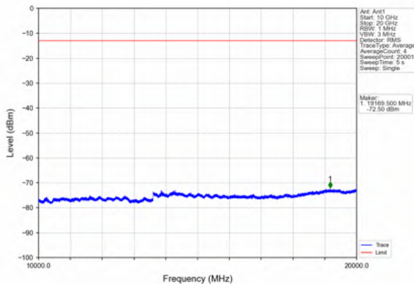
Band2_10MHz_QPSK_MCH_1880MHz_RB_1_0_NTNV
