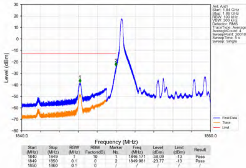
Band2 10MHz 256QAM LCH 1855MHz RB 1 0 NTNV
