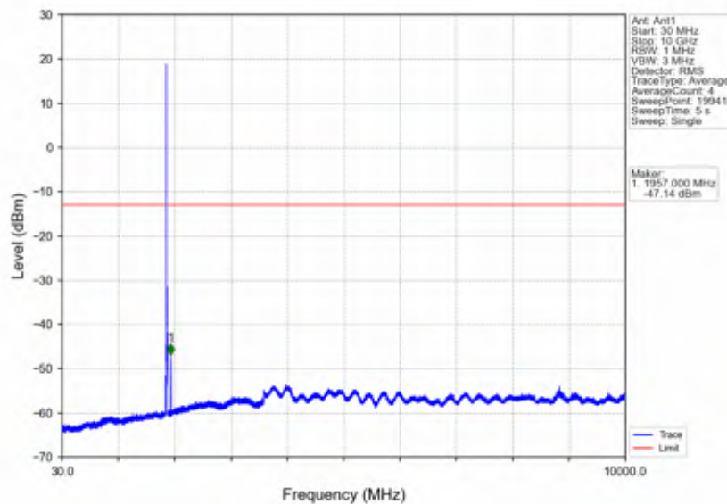
Band2_10MHz_256QAM_MCH_1880MHz_RB_1_0_NTNV
