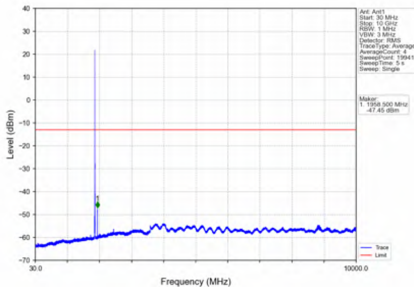
Band2_5MHz_QPSK_MCH_1880MHz_RB_1_0_NTNV
