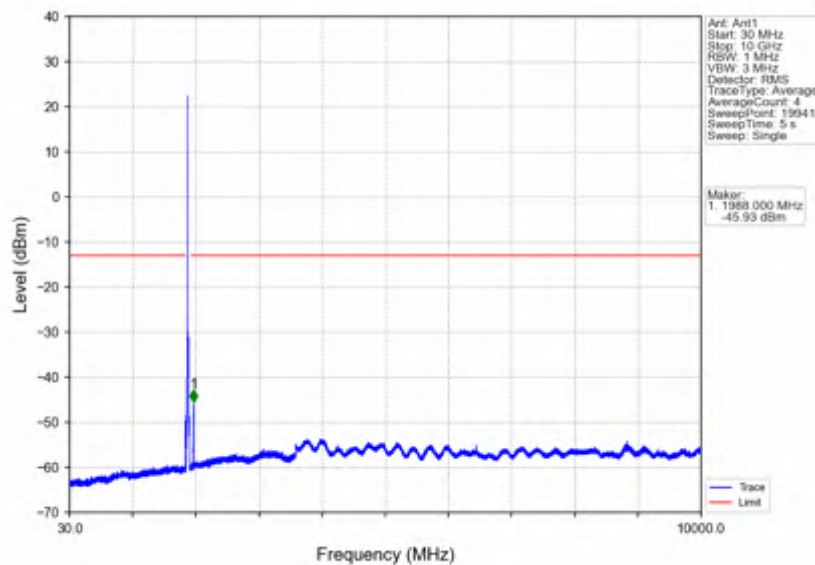
Band2_20MHz_16QAM_HCH_1900MHz_RB_1_0_NTNV
