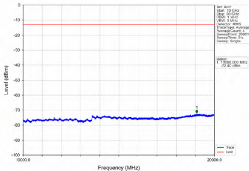
Band2_1.4MHz_QPSK_MCH_1880MHz_RB_1_0_NTNV
