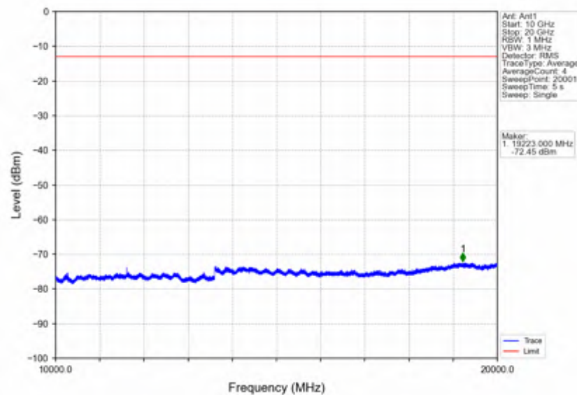
Band4 1.4MHz QPSK LCH 1710.7MHz RB 6 0 NTV
