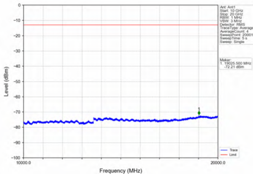
Band2_20MHz_QPSK_HCH_1900MHz_RB_1_0_NTNV
