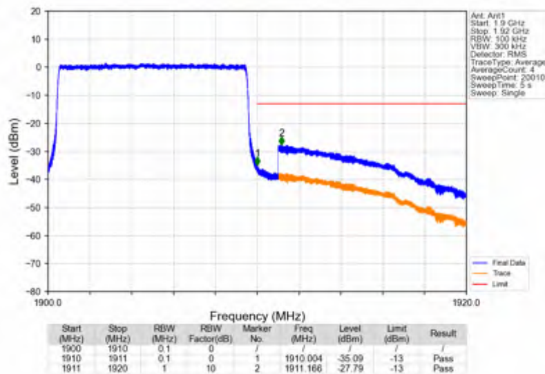
Band2_10MHz_256QAM_HCH_1905MHz_RB_50_0_NTNV
