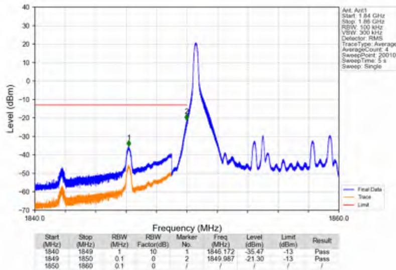
Band2_10MHz_64QAM_LCH_1855MHz_RB_1_0_NTNV
