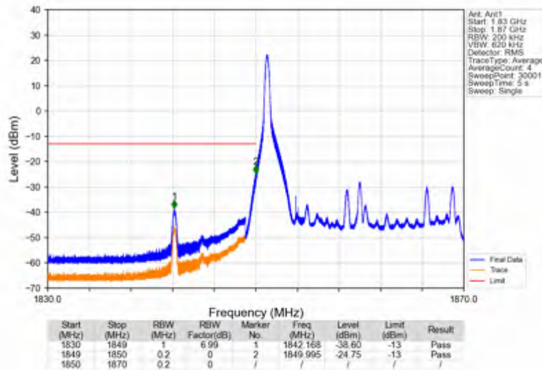
Band2_20MHz_QPSK_LCH_1860MHz_RB_100_0_NTNV
