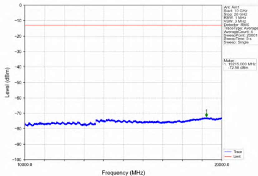
Band2 5MHz QPSK LCH 1852.5MHz RB 25 0 NTNV
