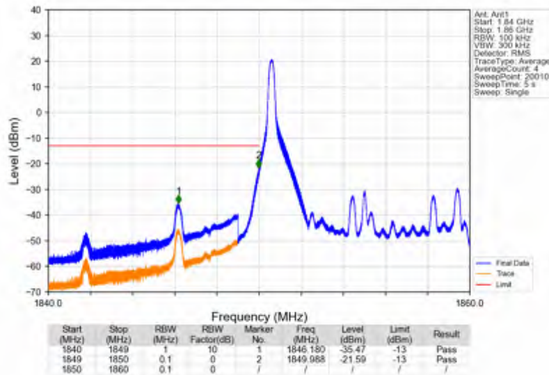
Band2 10MHz 64QAM LCH 1855MHz RB 50 0 NTNv
