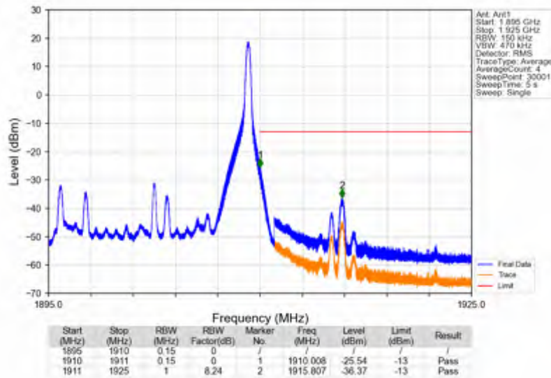
Band2_15MHz_256QAM_HCH_1902.5MHz_RB_1_74_NTNV
