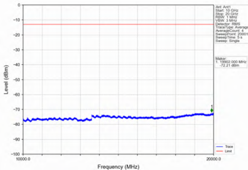
Band2_20MHz_16QAM_MCH_1880MHz_RB_1_0_NTNV
