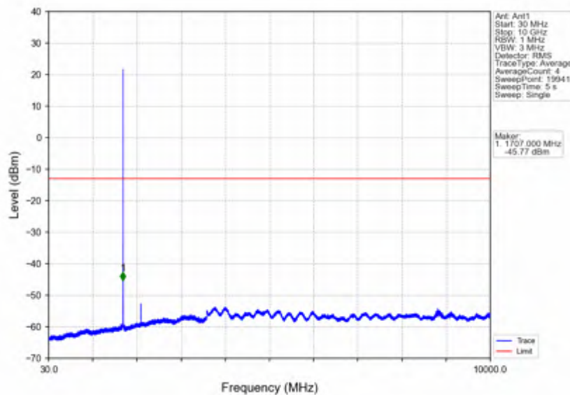
Band4 1.4MHz 64QAM LCH 1710.7MHz RB 1 0 NTNV
