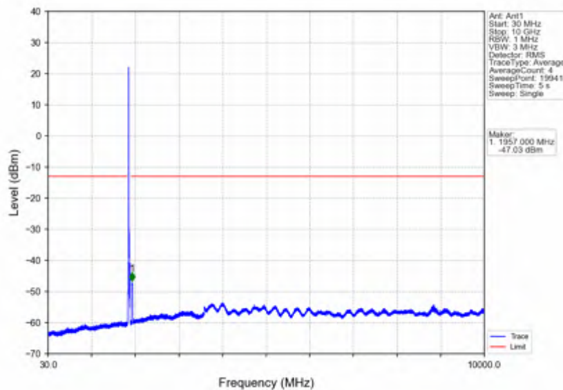
Band2_20MHz_16QAM_MCH_1880MHz_RB_1_0_NTNV
