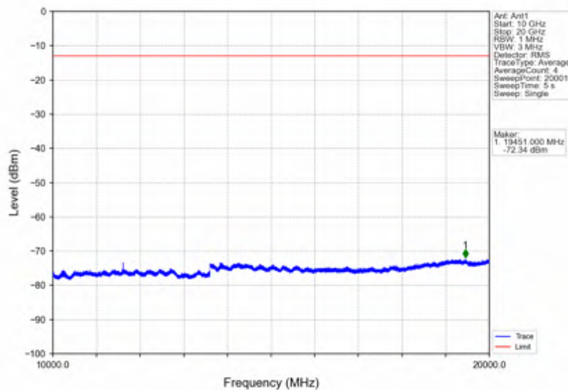
Band2_20MHz_16QAM_HCH_1900MHz_RB_1_0_NTNV
