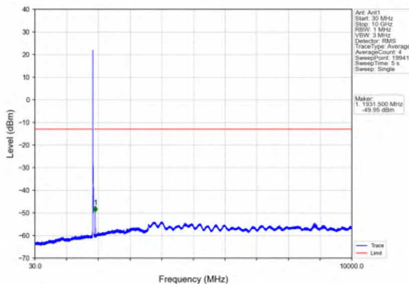
Band2_15MHz_QPSK_LCH_1857.5MHz_RB_1_0_NTNV
