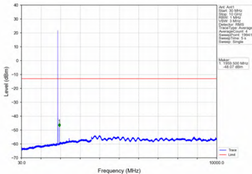
Band2_3MHz_QPSK_MCH_1880MHz_RB_1_0_NTNV
