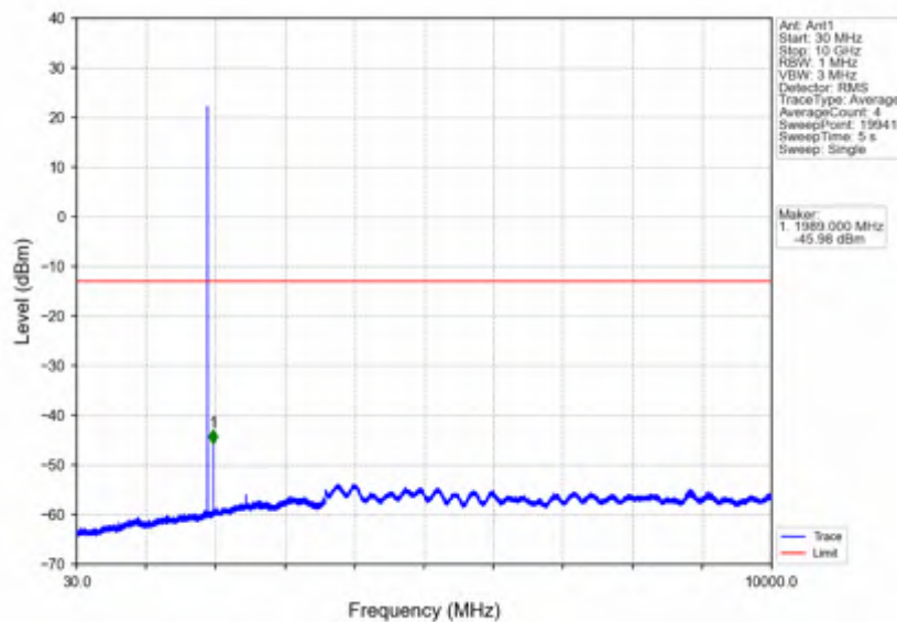
Band2_3MHz_QPSK_HCH_1908.5MHz_RB_1_0_NTNV
