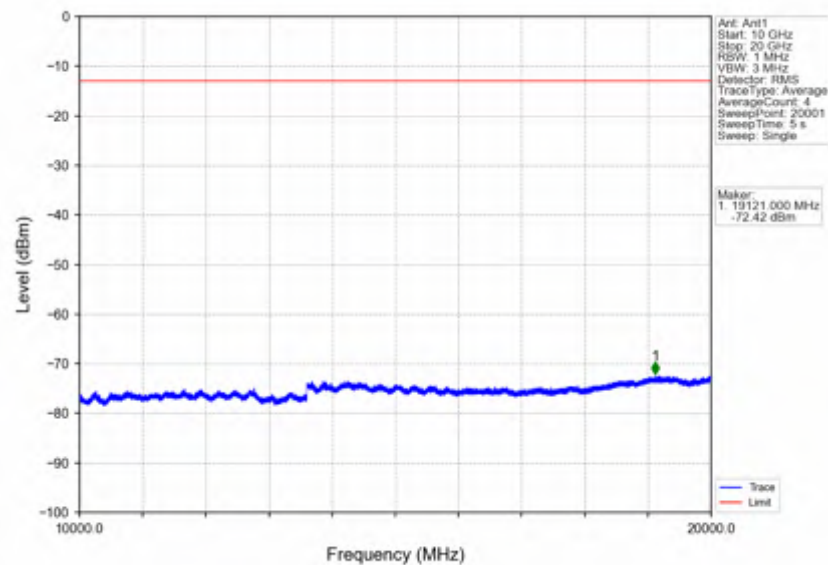
Band2_20MHz_QPSK_LCH_1860MHz_RB_100_0_NTNV
