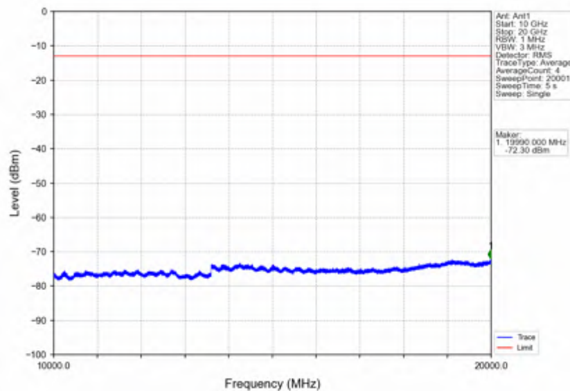
Band2 20MHz QPSK MCH 1880MHz RB 1 0 NTNV
