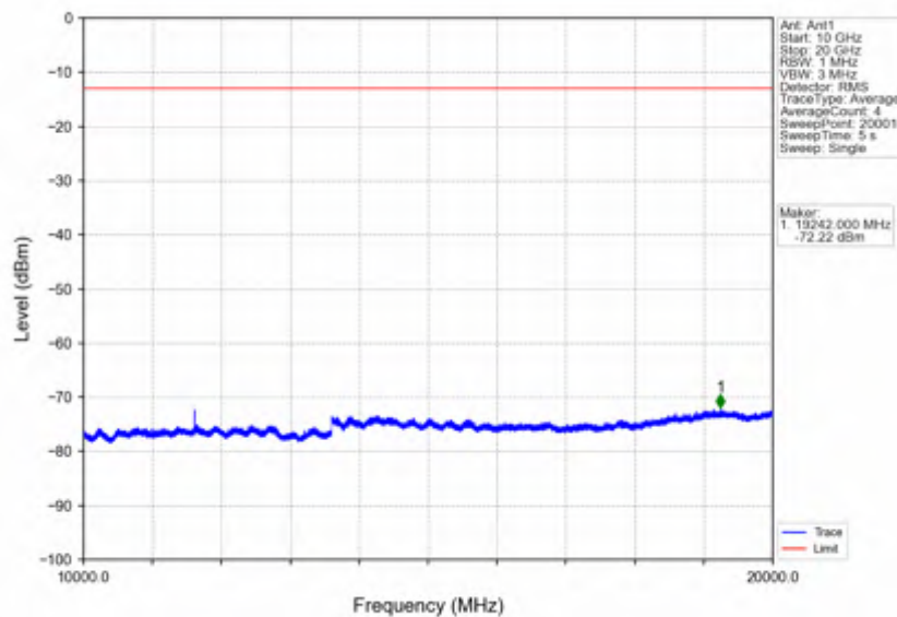
Band2_20MHz_256QAM_HCH_1900MHz_RB_1_0_NTNV
