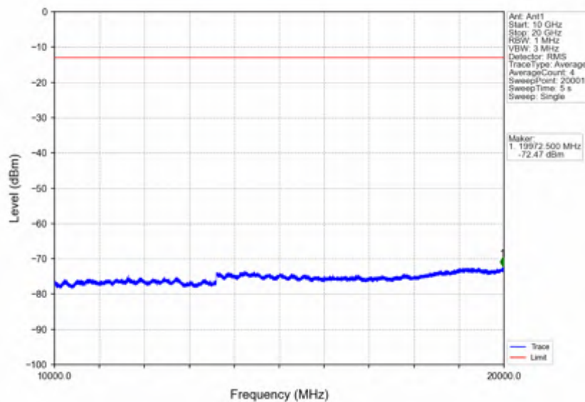
Band2_10MHz_QPSK_HCH_1905MHz_RB_1_0_NTNV
