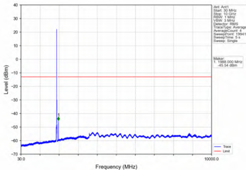
Band2_15MHz_QPSK_HCH_1902.5MHz_RB_1_0_NTNV
