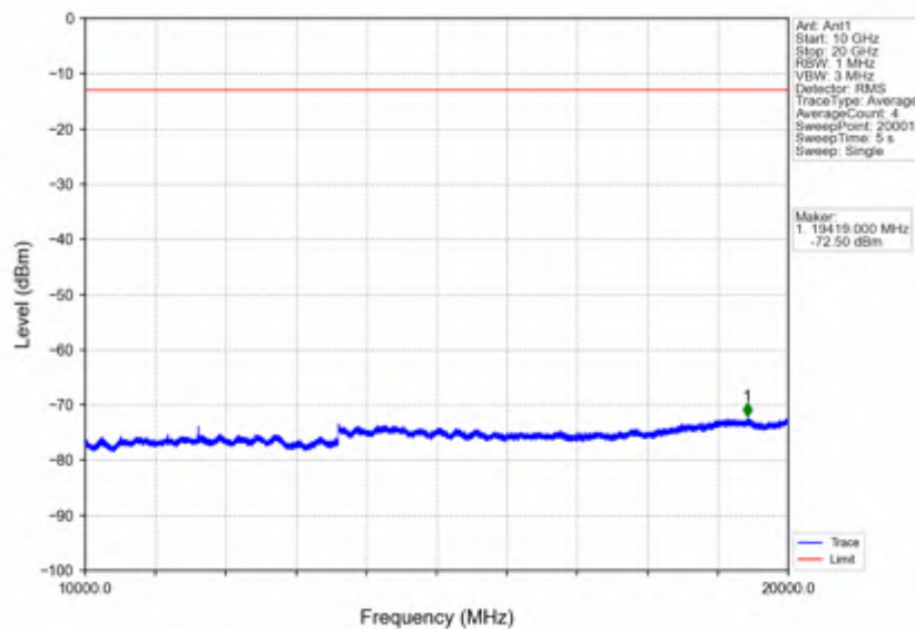
Band2_1.4MHz_QPSK_HCH_1909.3MHz_RB_1_0_NTNV
