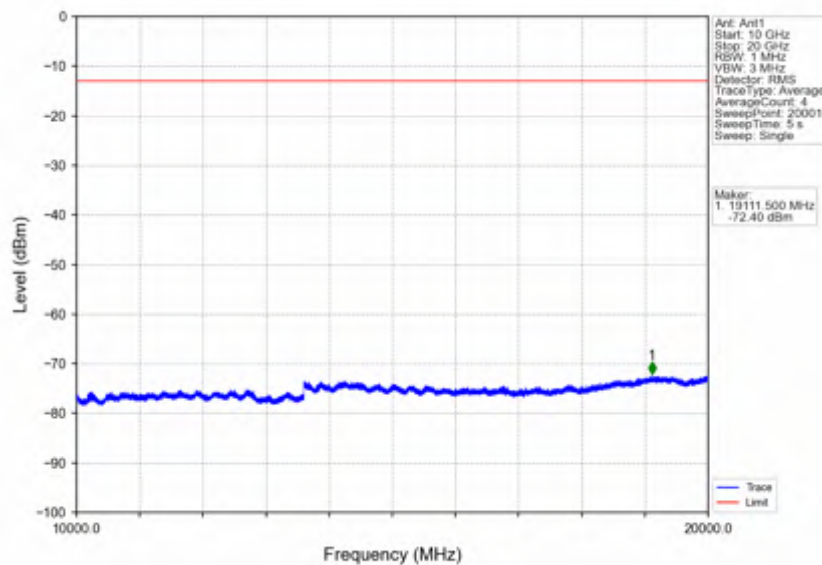
Band2_10MHz_16QAM_HCH_1905MHz_RB_1_0_NTNV
