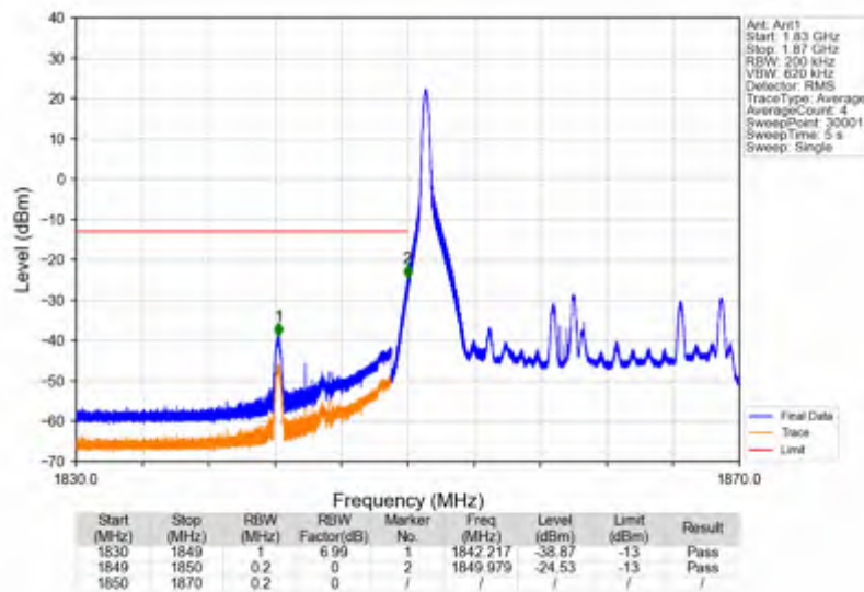
Band2_20MHz_16QAM_LCH_1860MHz_RB_100_0_NTNV
