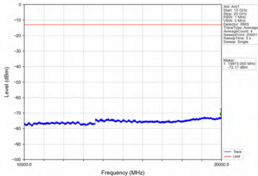
Band4 1.4MHz 16QAM LCH 1710.7MHz RB 6 0 NTN
