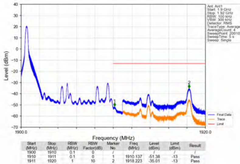
Band2_10MHz_16QAM_HCH_1905MHz_RB_50_0_NTNV
