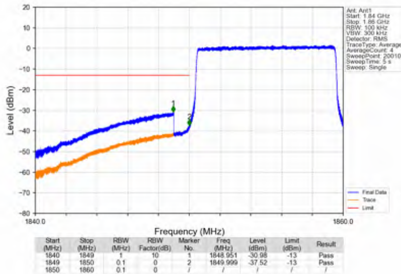
Band2_10MHz_256QAM_LCH_1855MHz_RB_50_0_NTNV
