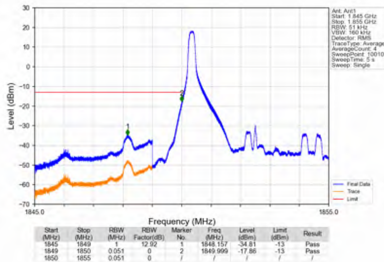
Band2 5MHz QPSK LCH 1852.5MHz RB 25 0 NTNV
