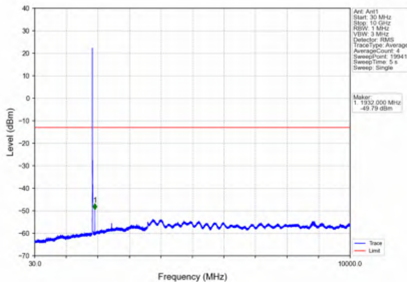
Band2_10MHz_16QAM_LCH_1855MHz_RB_1_0_NTNV
