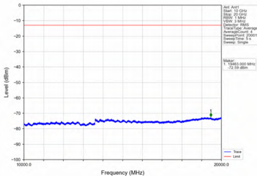
Band2_3MHz_QPSK_HCH_1908.5MHz_RB_1_0_NTNV
