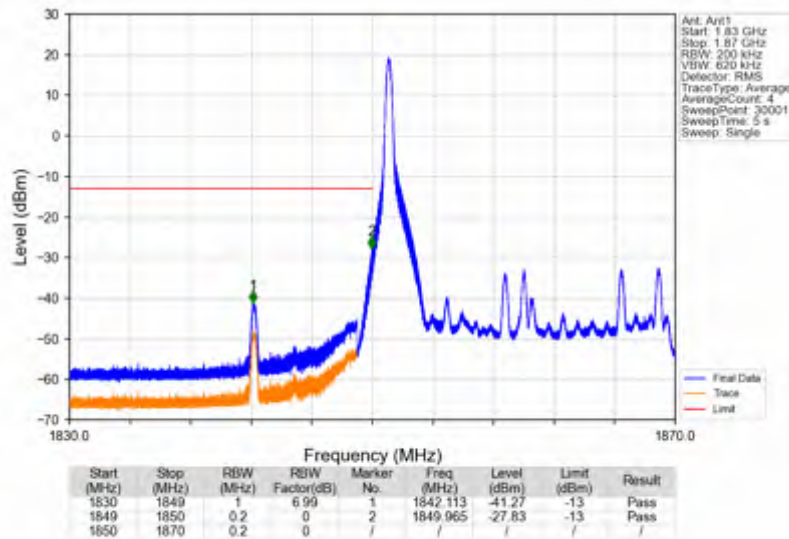
Band2 20MHz 256QAM LCH 1860MHz RB 1 0 NTNV
