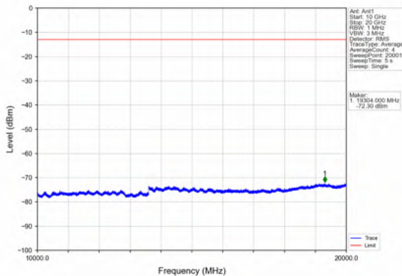
Band2_15MHz_QPSK_HCH_1902.5MHz_RB_1_0_NTNV
