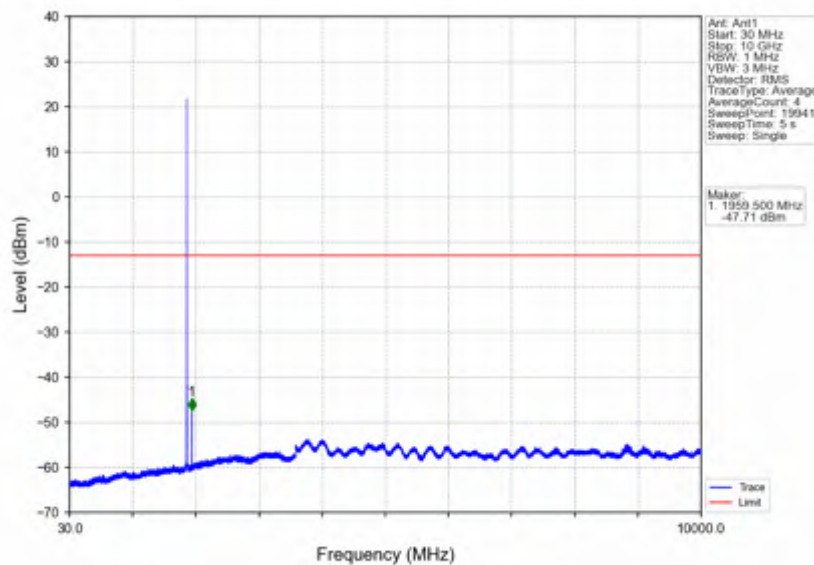
Band2_3MHz_16QAM_MCH_1880MHz_RB_1_0_NTNV
