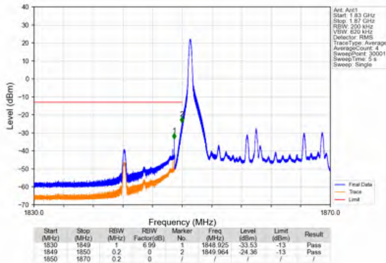
Band2_20MHz_16QAM_LCH_1860MHz_RB_1_0_NTNV
