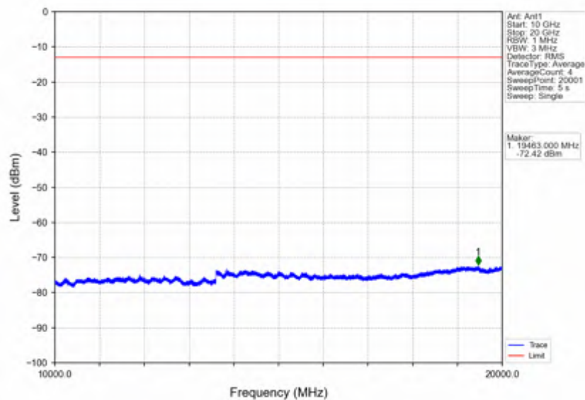
Band2_20MHz_16QAM_LCH_1860MHz_RB_100_0_NTNV
