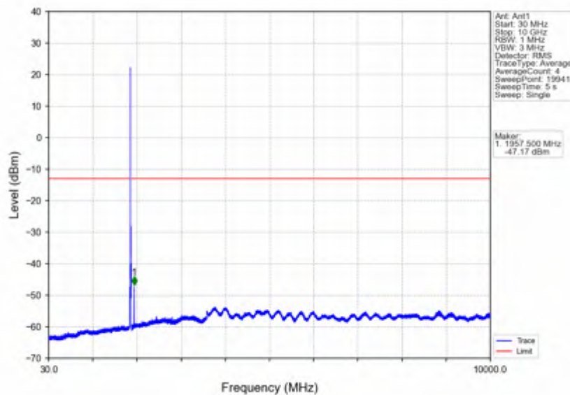
Band2_10MHz_QPSK_MCH_1880MHz_RB_1_0_NTNV
