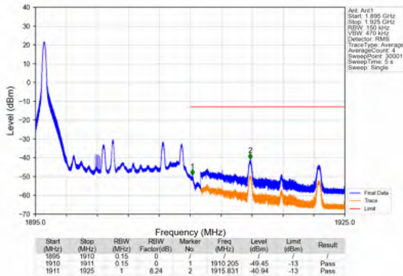
Band2_15MHz_QPSK_HCH_1902.5MHz_RB_1_74_NTNV
