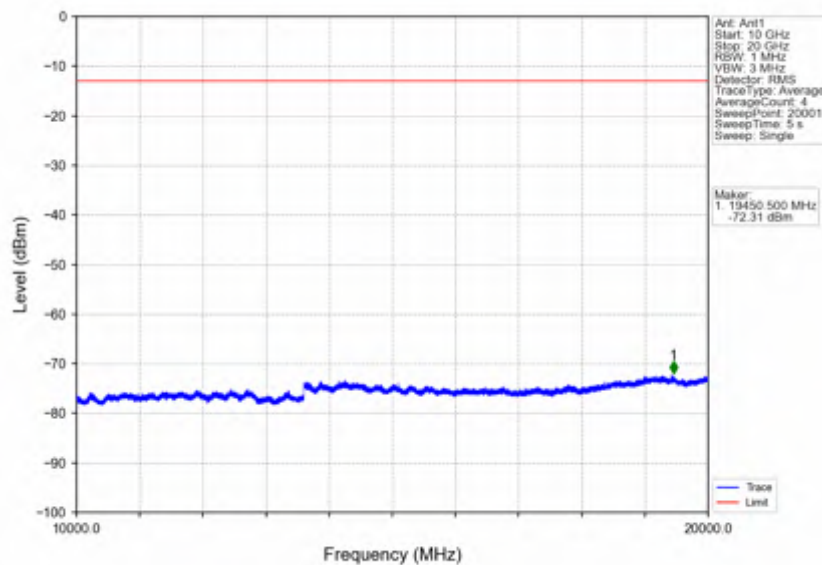
Band2_3MHz_256QAM_HCH_1908.5MHz_RB_1_0_NTNV
