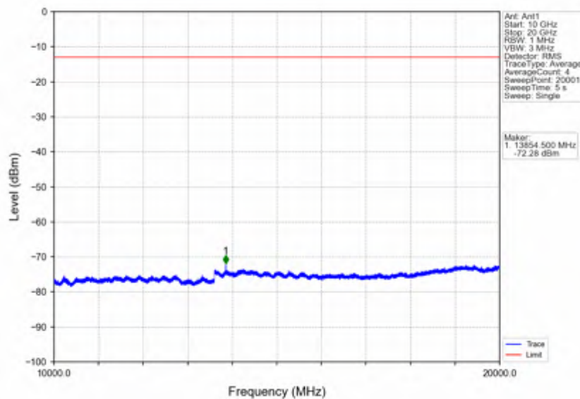
Band2_15MHz_QPSK_MCH_1880MHz_RB_1_0_NTNV
