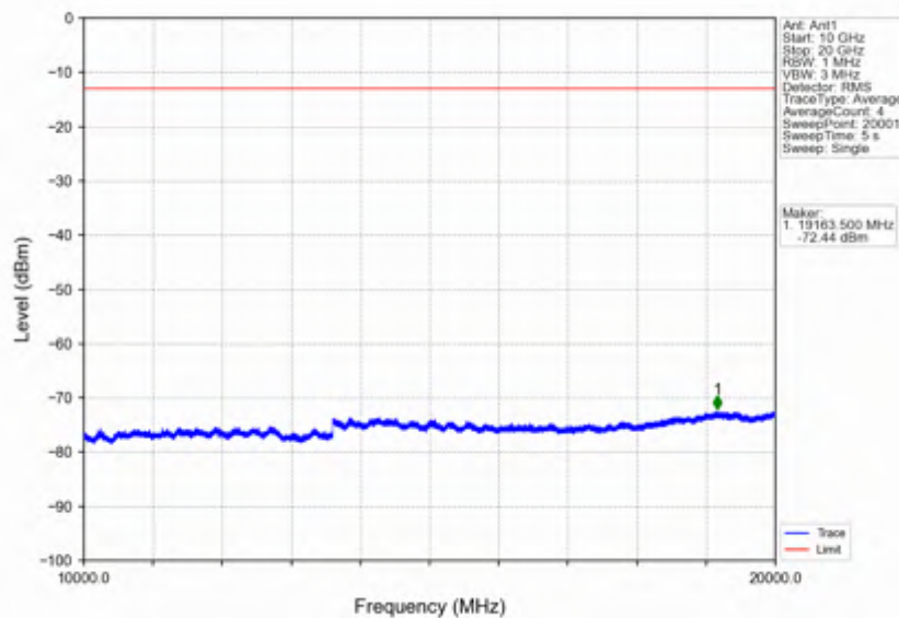
Band2_3MHz_16QAM_MCH_1880MHz_RB_1_0_NTNV
