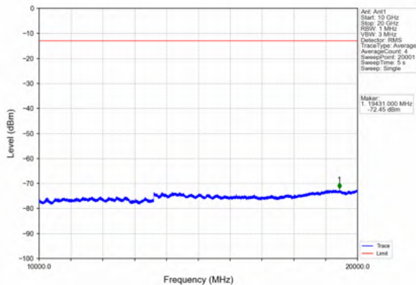
Band2 20MHz 64QAM LCH 1860MHz RB 100 0 NTNv
