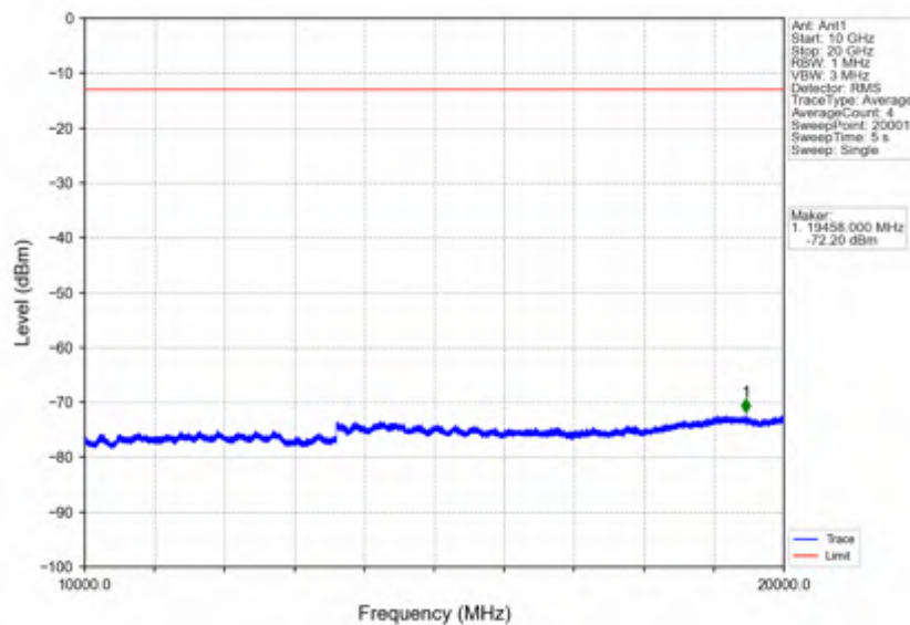
Band2_20MHz_64QAM_MCH_1880MHz_RB_1_0_NTNV
