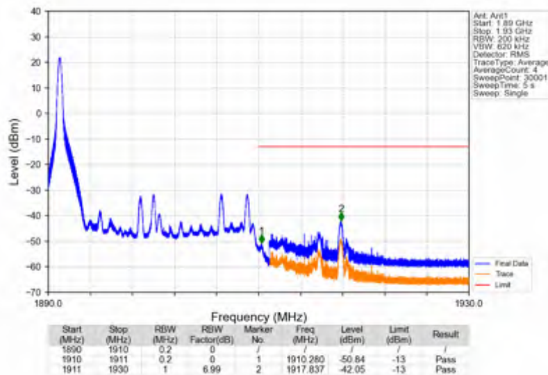
Band2_20MHz_QPSK_HCH_1900MHz_RB_100_0_NTNV
