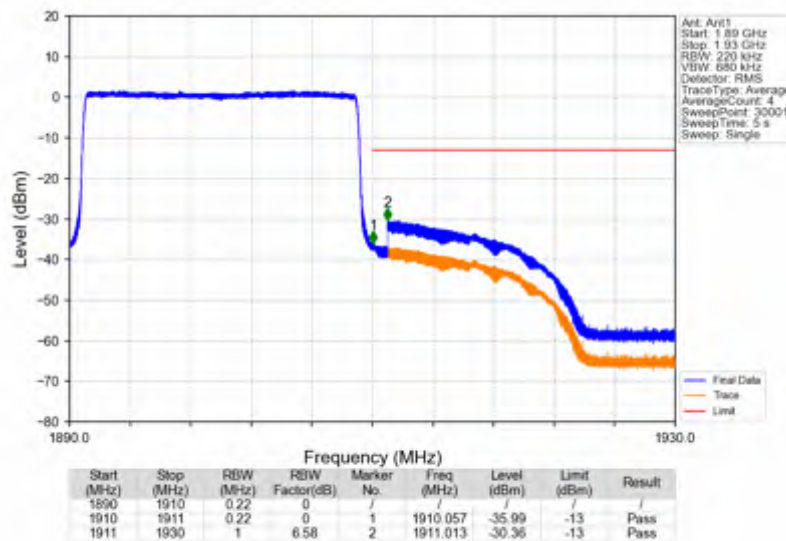
Band2_20MHz_256QAM_HCH_1900MHz_RB_100_0_NTNV
