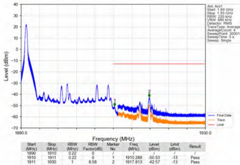
Band2_20MHz_64QAM_HCH_1900MHz_RB_1_99_NTNV
