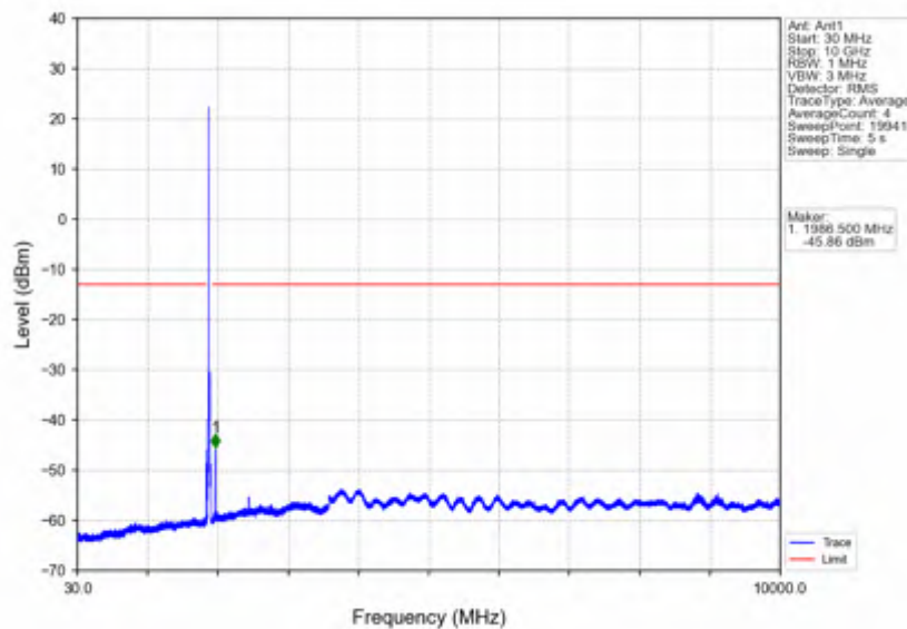
Band2_20MHz_QPSK_HCH_1900MHz_RB_1_0_NTNV
