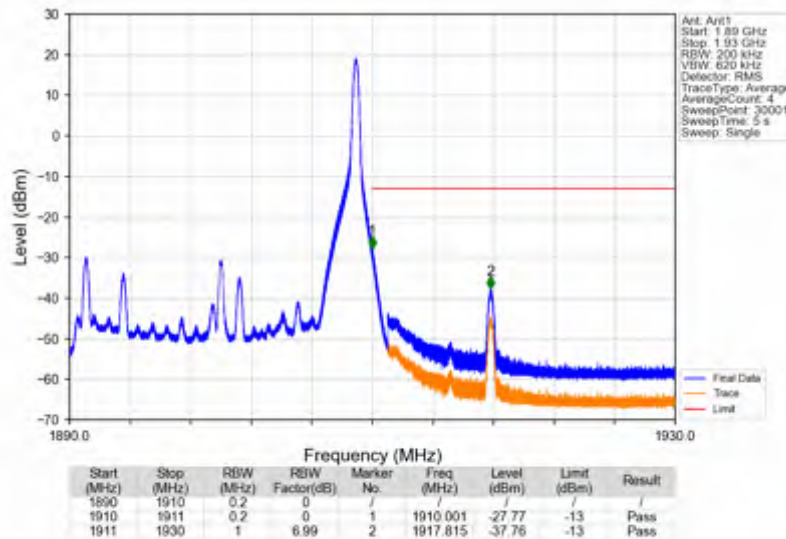
Band2_20MHz_256QAM_HCH_1900MHz_RB_1_99_NTNV
