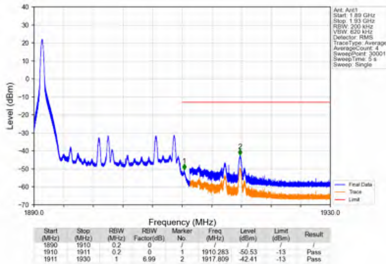
Band2_20MHz_QPSK_HCH_1900MHz_RB_1_99_NTNV
