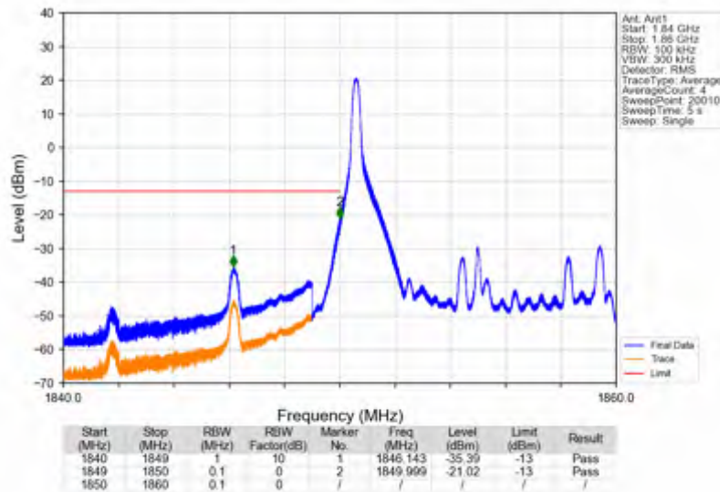
Band2_10MHz_QPSK_LCH_1855MHz_RB_50_0_NTNV
