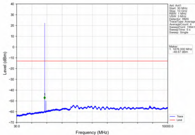
Band2_1.4MHz_QPSK_MCH_1880MHz_RB_1_0_NTNV
