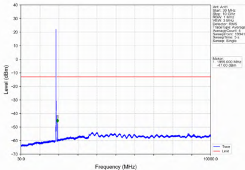
Band2_15MHz_QPSK_MCH_1880MHz_RB_1_0_NTNV
