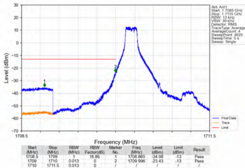
Band4 1.4MHz 16QAM LCH 1710.7MHz RB 6 0 NTN
