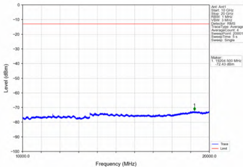
Band2_5MHz_QPSK_MCH_1880MHz_RB_1_0_NTNV
