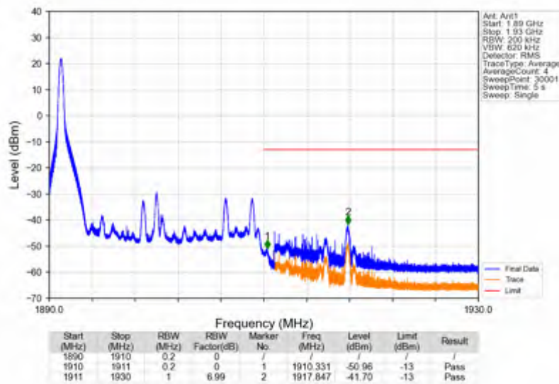
Band2_20MHz_16QAM_HCH_1900MHz_RB_100_0_NTNV
