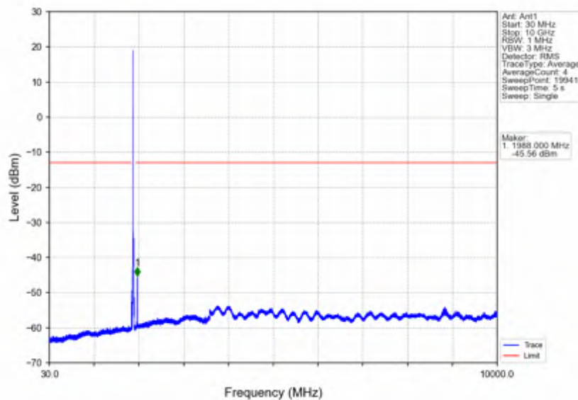
Band2_20MHz_256QAM_HCH_1900MHz_RB_1_0_NTNV
