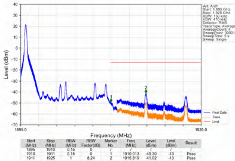
Band2_15MHz_16QAM_HCH_1902.5MHz_RB_1_74_NTNV
