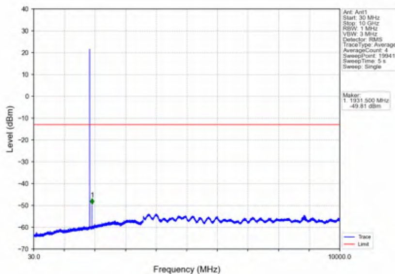
Band2_3MHz_QPSK_LCH_1851.5MHz_RB_1_0_NTNV
