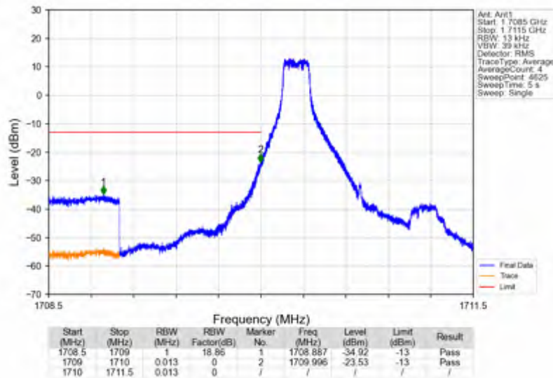
Band4 1.4MHz 64QAM LCH 1710.7MHz RB 1 0 NTNv
