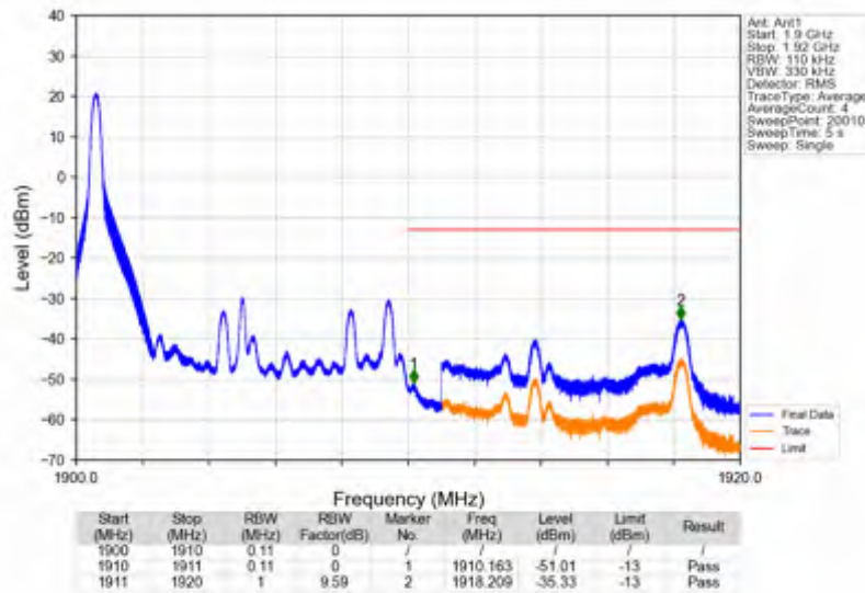
Band2_10MHz_16QAM_HCH_1905MHz_RB_1_49_NTNV
