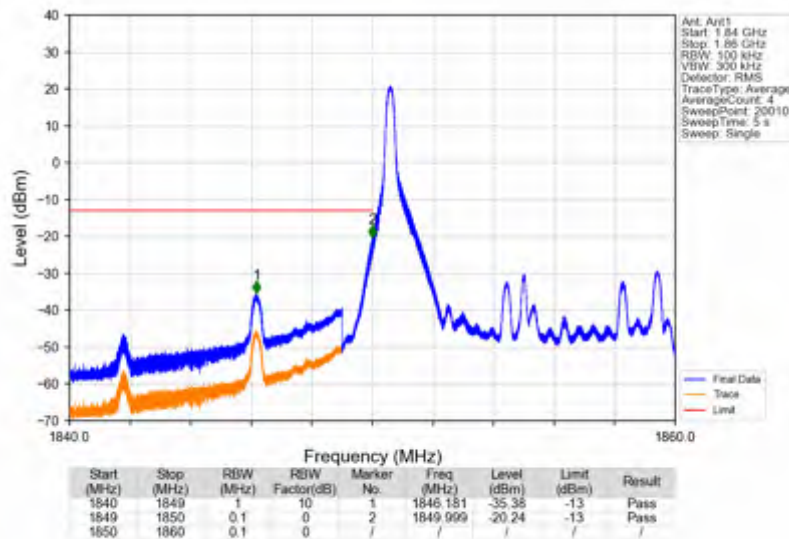
Band2_10MHz_QPSK_LCH_1855MHz_RB_1_0_NTNV
