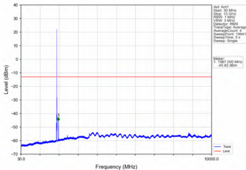
Band2_10MHz_16QAM_HCH_1905MHz_RB_1_0_NTNV
