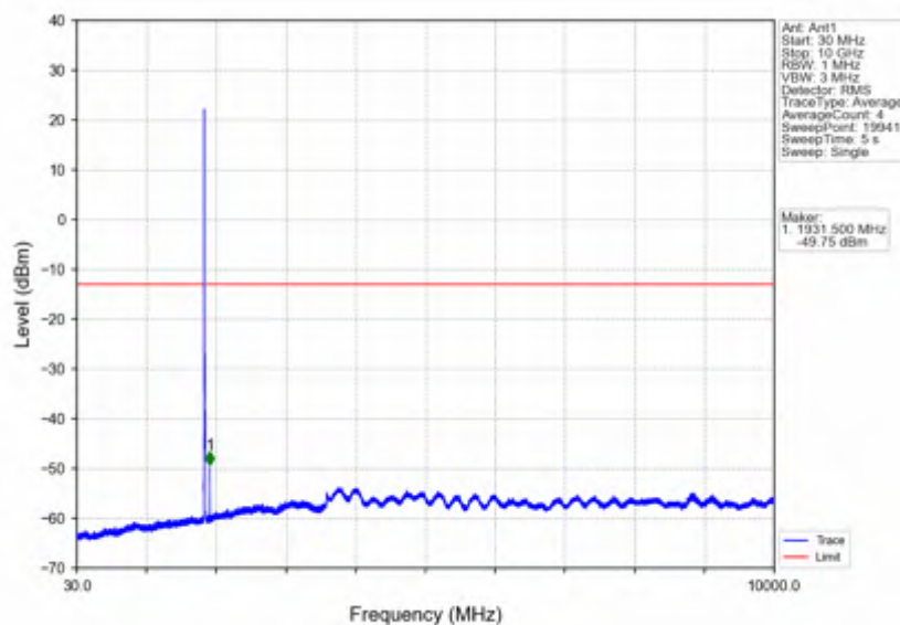
Band2_10MHz_QPSK_LCH_1855MHz_RB_1_0_NTNV
