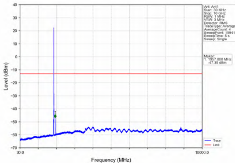
Band2_10MHz_16QAM_MCH_1880MHz_RB_1_0_NTNV
