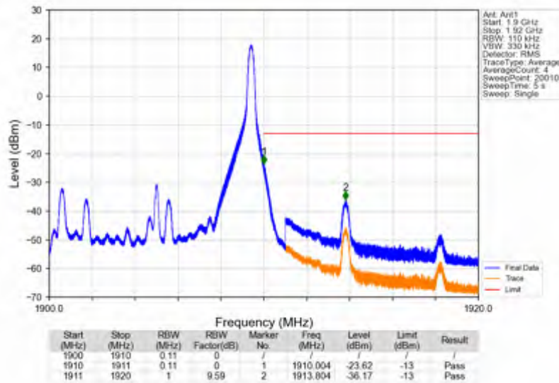
Band2_10MHz_256QAM_HCH_1905MHz_RB_1_49_NTNV
