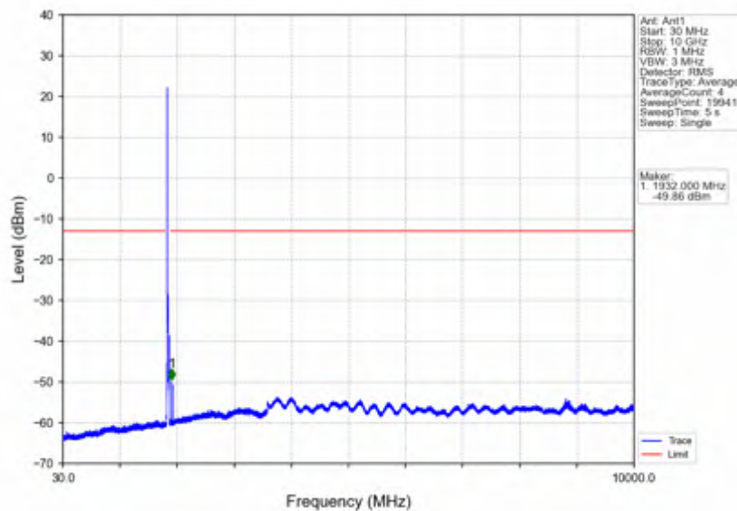
Band2 20MHz 64QAM LCH 1860MHz RB 1 0 NTNV
