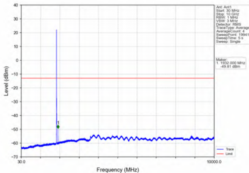
Band2_10MHz_64QAM_LCH_1855MHz_RB_1_0_NTNV
