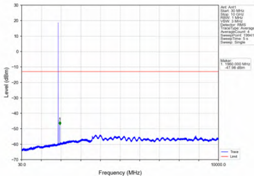
Band2_3MHz_256QAM_MCH_1880MHz_RB_1_0_NTNV
