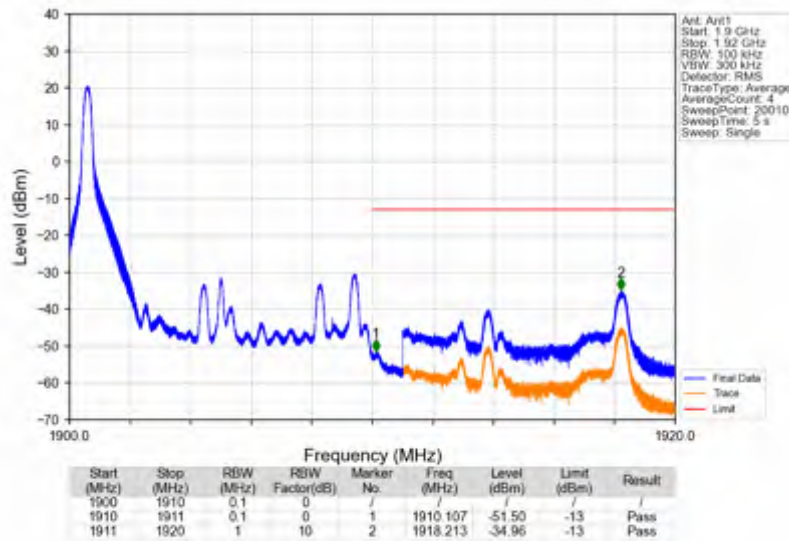
Band2_10MHz_QPSK_HCH_1905MHz_RB_50_0_NTNV
