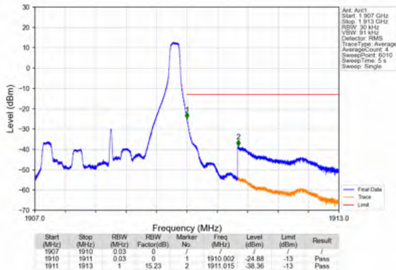
Band2_3MHz_256QAM_HCH_1908.5MHz_RB_1_14_NTNV
