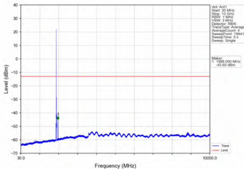
Band2_10MHz_QPSK_HCH_1905MHz_RB_1_0_NTNV
