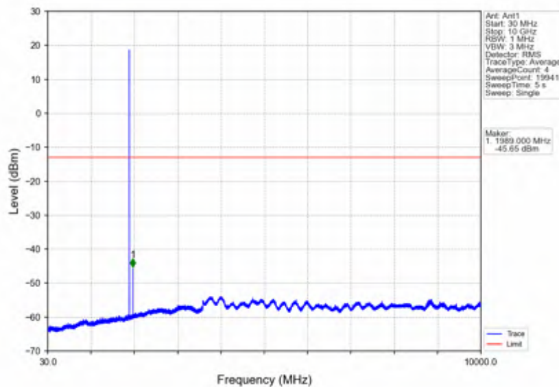
Band2_3MHz_256QAM_HCH_1908.5MHz_RB_1_0_NTNV
