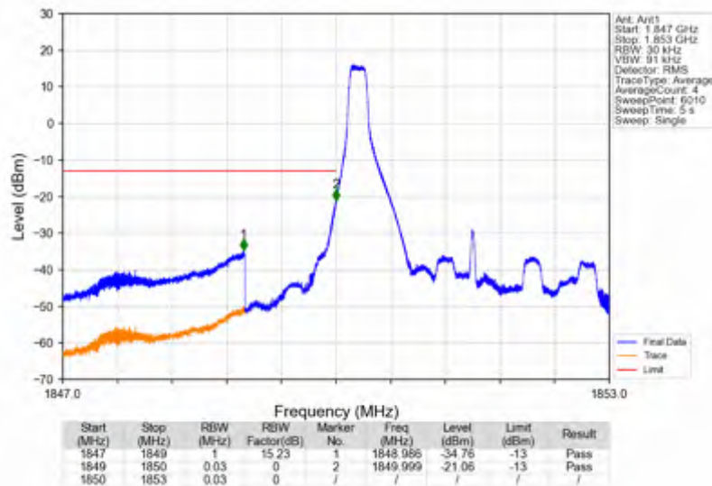
Band2_3MHz_QPSK_LCH_1851.5MHz_RB_1_0_NTNV
