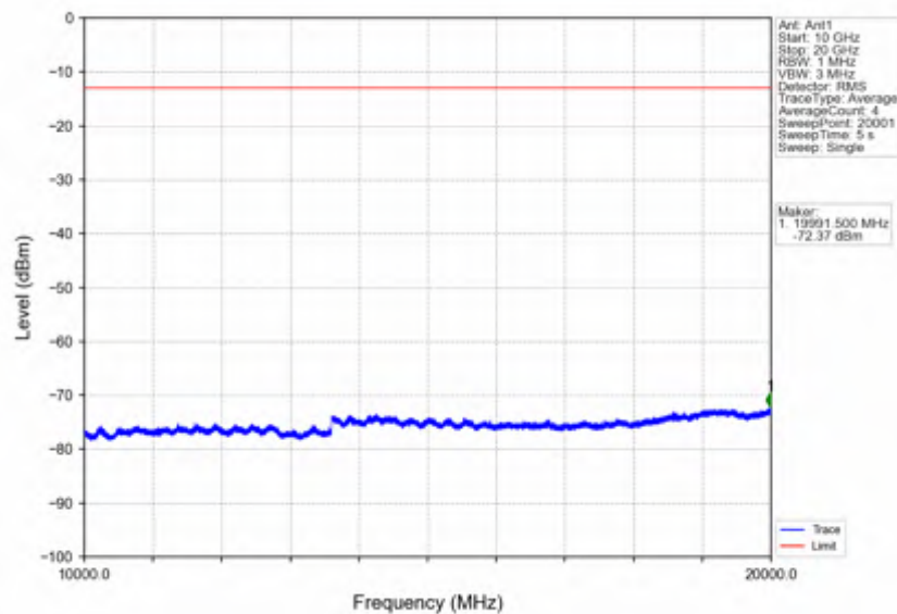
Band2_10MHz_256QAM_LCH_1855MHz_RB_50_0_NTNV
