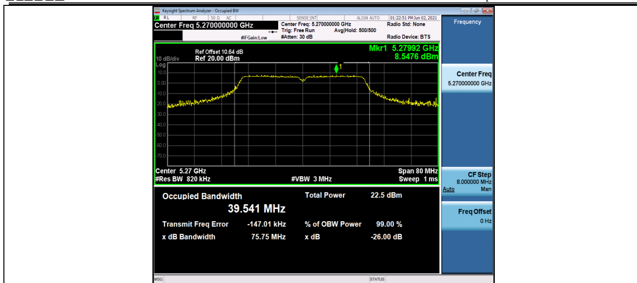
11N40SISO_Ant1_5270
