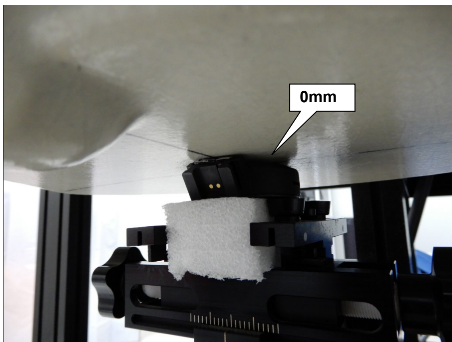
EUT Back_0mm
