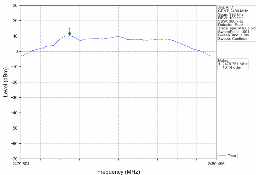
S2_HCH_2480MHz_Ant1_NTNV
