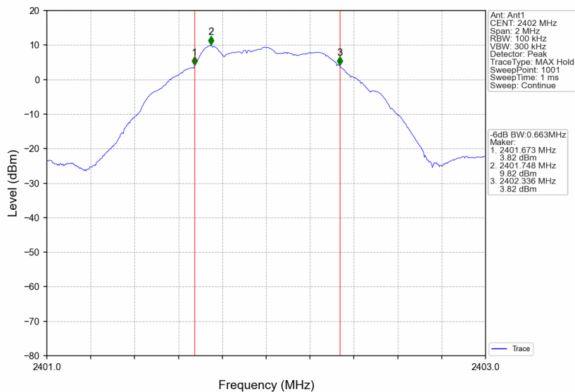
S2_LCH_2402MHz_Ant1_NTNV
