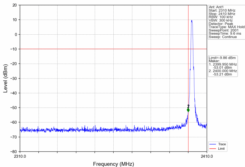
S2_LCH_2402MHz_Ant1_NTNV
