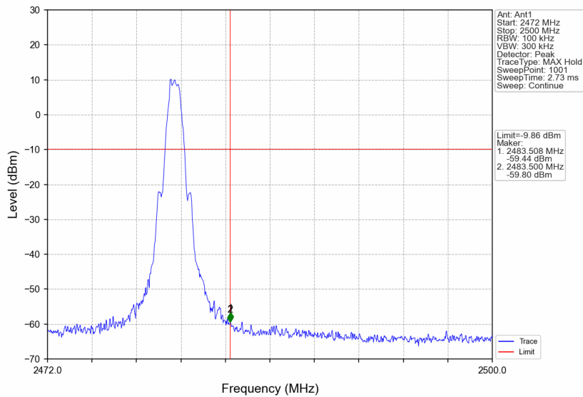
S2_HCH_2480MHz_Ant1_NTNV
