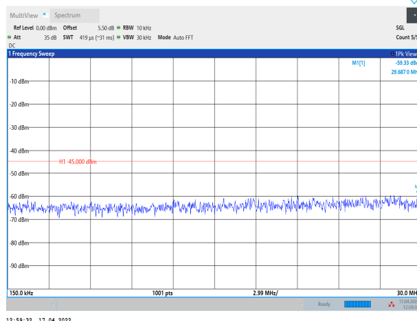
Band38-20MHz-QPSK-37850-1RB#0-Range2:0.15~30MHz
