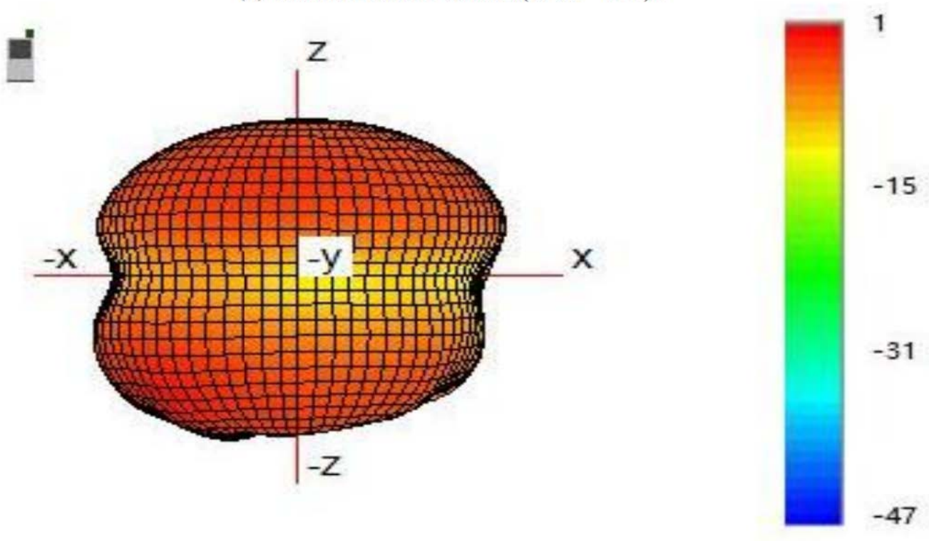
(4) 2420MHz 的 3D 方向图(单位： dBi):
