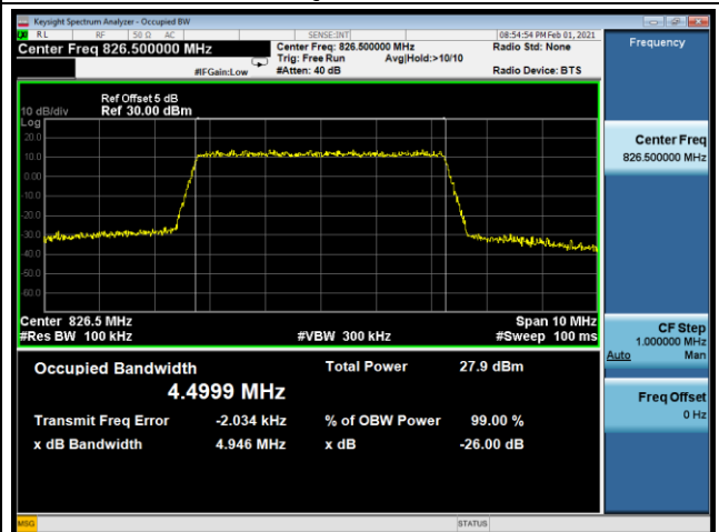
16QAM-27015
