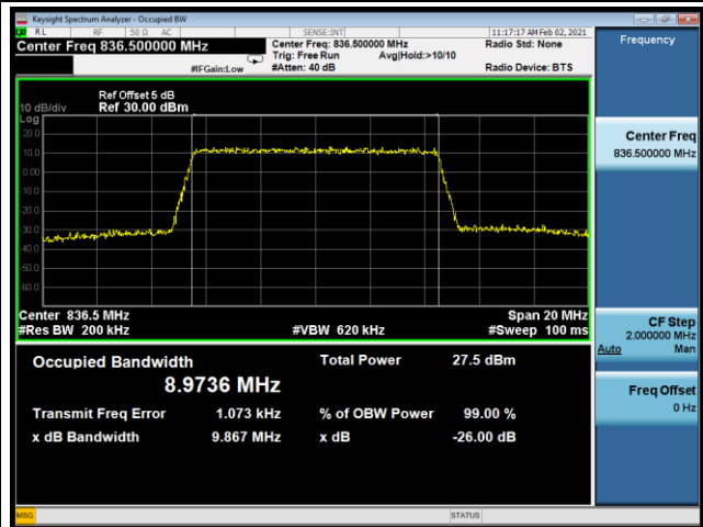
64QAM-26915
