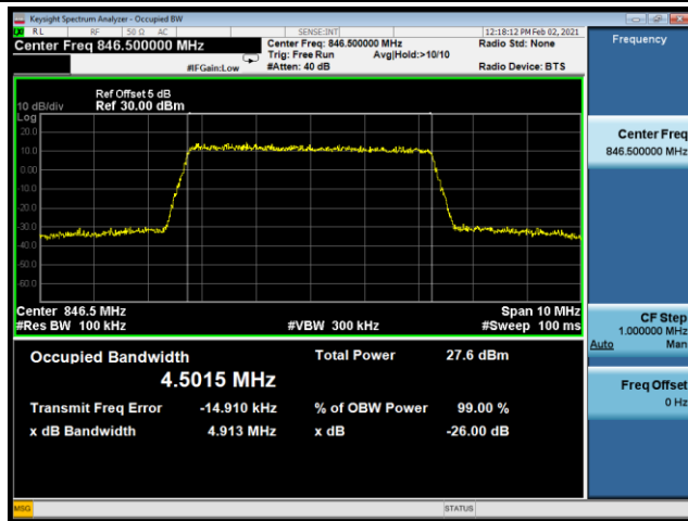
64QAM-20625
