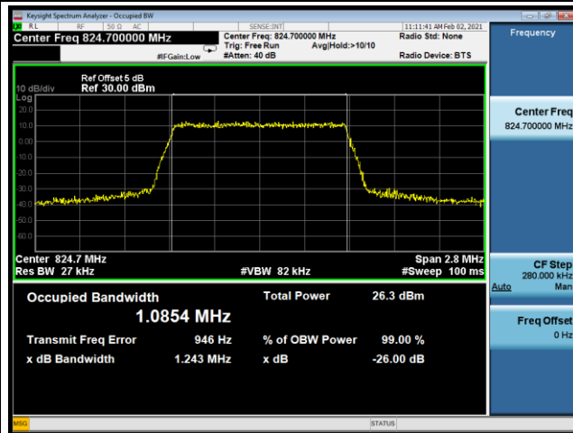
64QAM-27033
