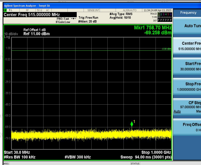
2.4G_Ant1_2436_30~1000
