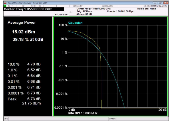
B66_N2(10M)_DFT-s-OFDM_PI_2-BPSK_Edge 1RB_Left_Low_CH
