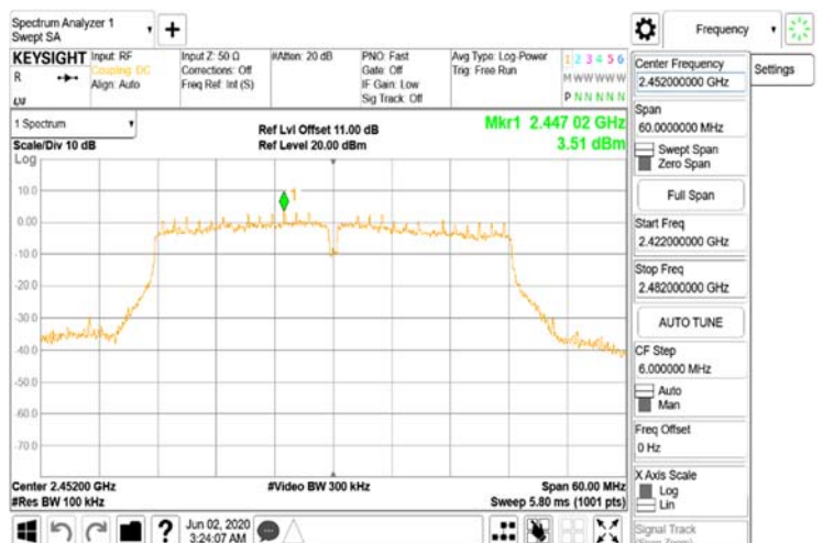
FCC_15_247_WLAN\Reference Level_802.11n_40MHz_Chain0_2452MHz
