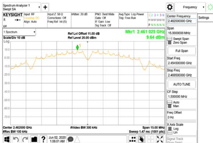
FCC_15_247_WLAN\Reference Level_802.11b_20MHz_Chain0_2462MHz
