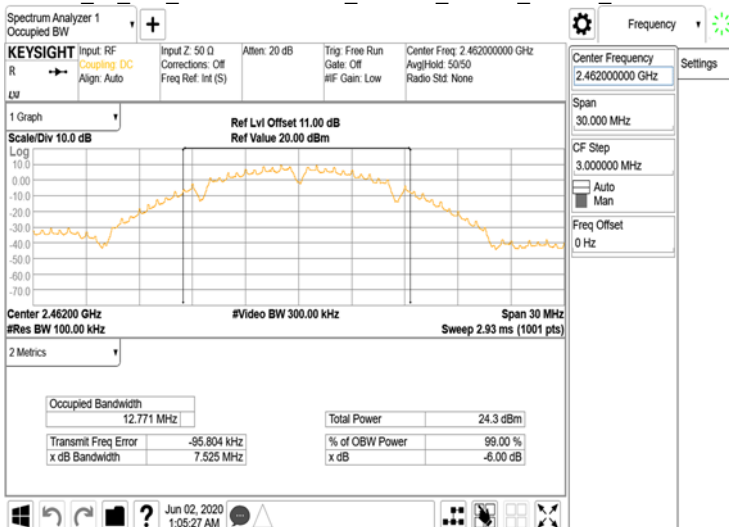
FCC_15_247_WLAN\OBW 6dB_802.11b_20MHz_Chain0_2462MHz
