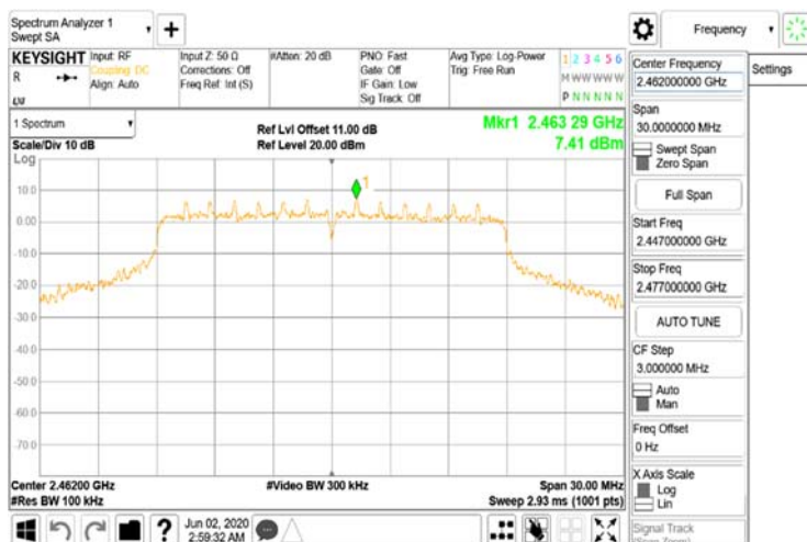
FCC_15_247_WLAN\Reference Level_802.11n_20MHz_Chain0_2462MHz
