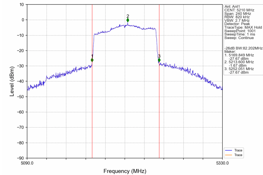
802.11ac(VHT80) _MCH_5210MHz_Ant1_NTNV
