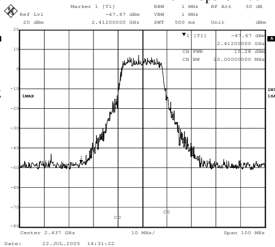
54Mbps-CH 06
