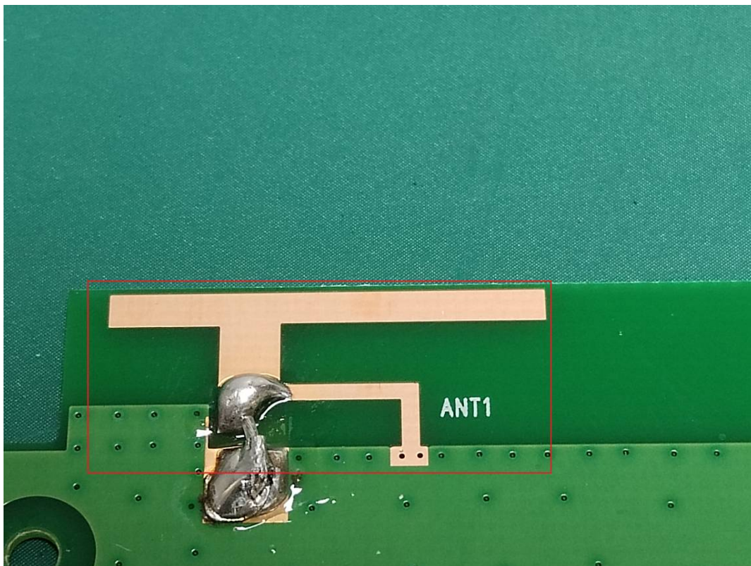
Wi-Fi ANT1
