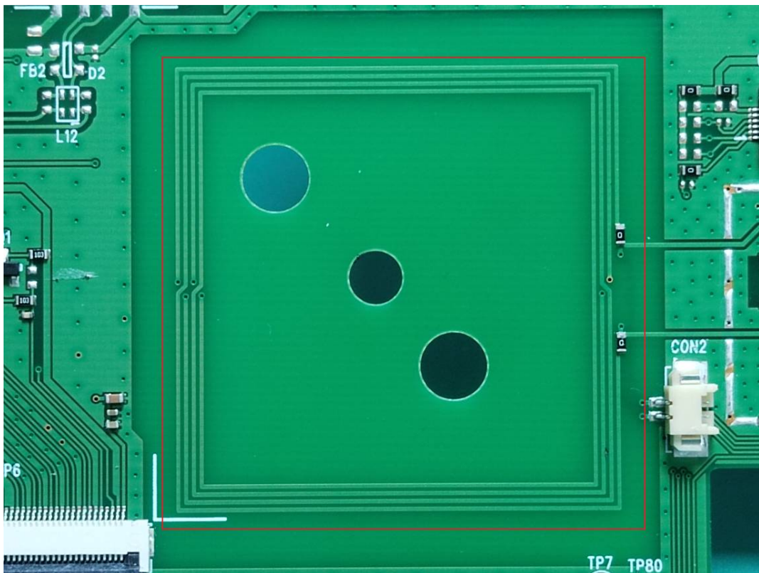
NFC ANT
