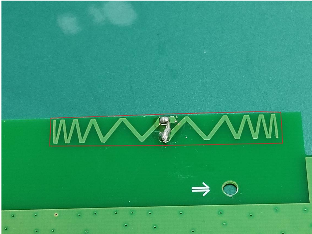
NFC ANT
