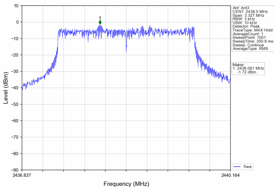
3M_MCH_2438.5MHz_Ant3_NTNV
