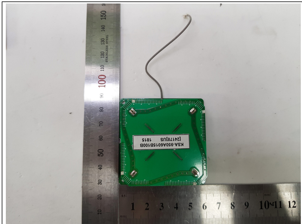
<RFID Antenna>
