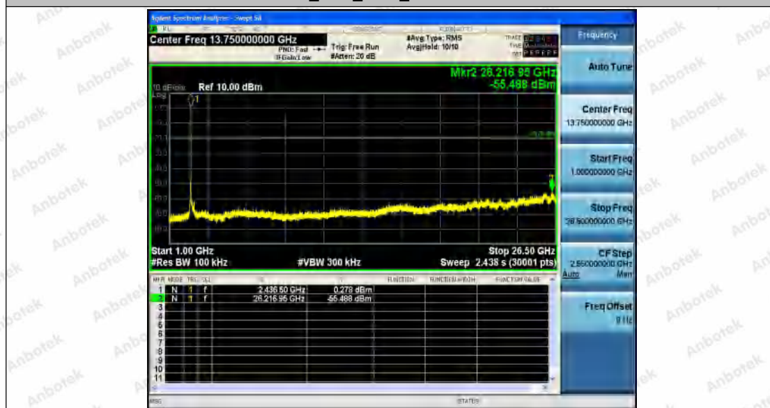
11B_Ant2_2437_0~Reference
