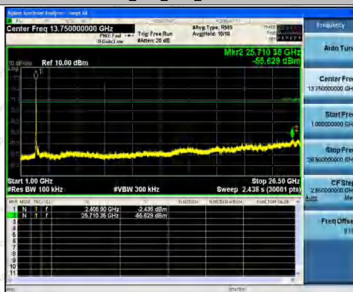
11N20_Ant2_2412_0~Reference
