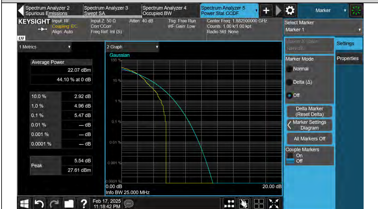
Band25-20MHz-16QAM-26365-27RB#0
