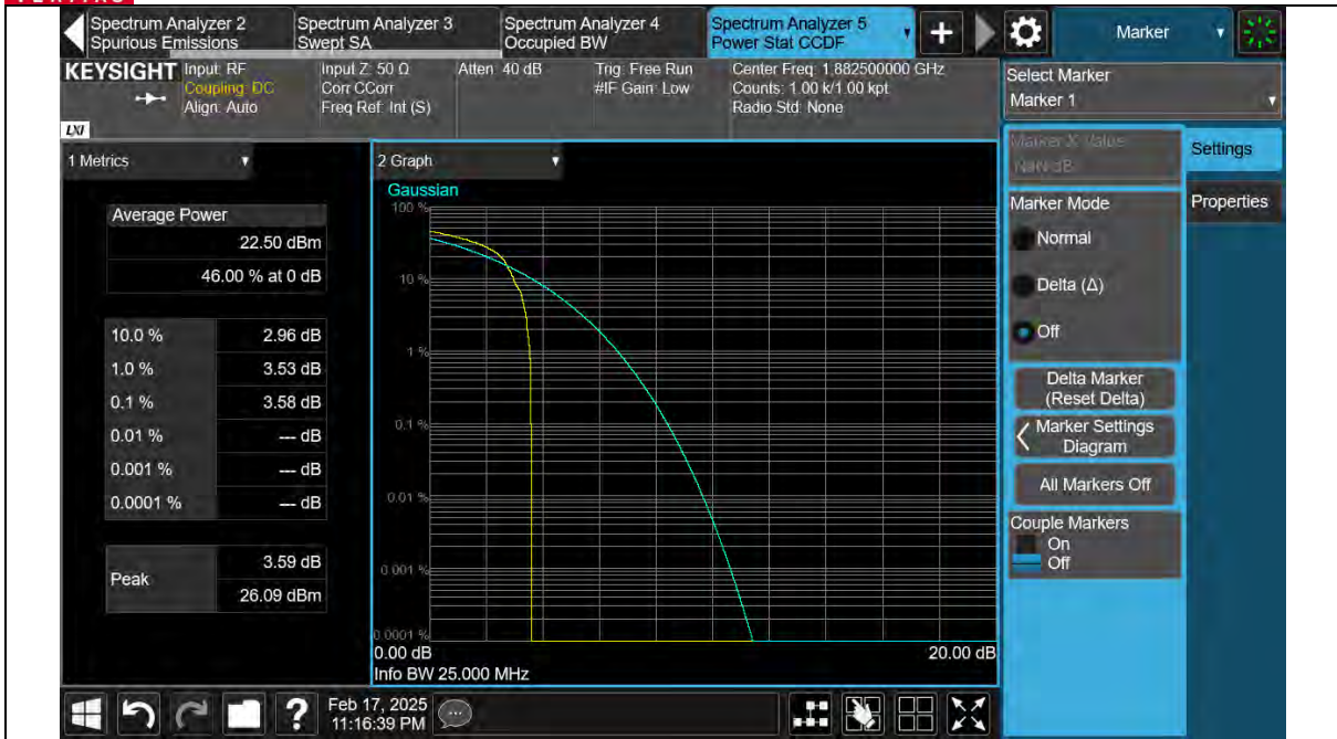
Band25-20MHz-QPSK-26365-1RB#0
