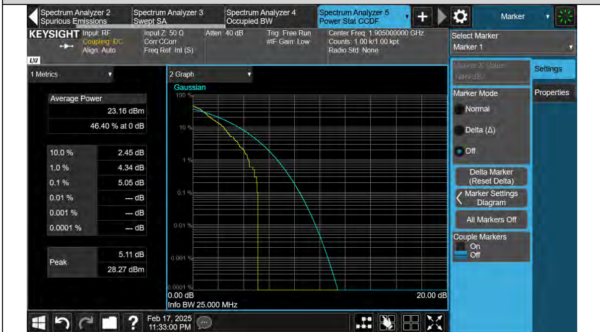
Band25-20MHz-QPSK-26590-100RB#0
