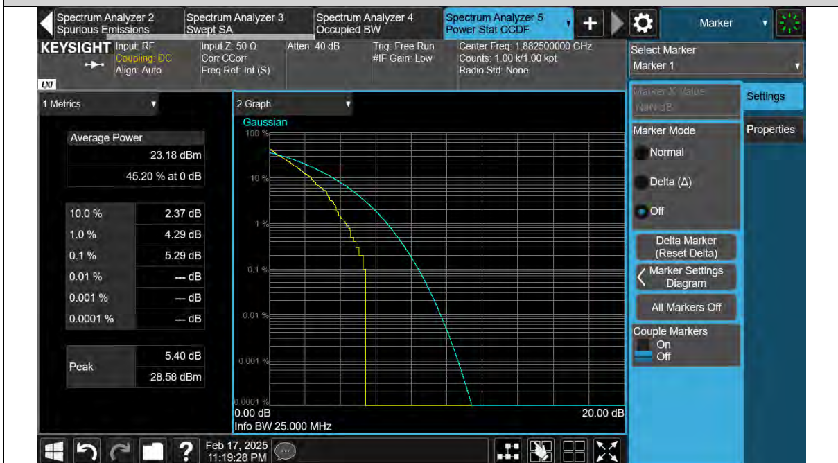
Band25-20MHz-QPSK-26365-100RB#0
