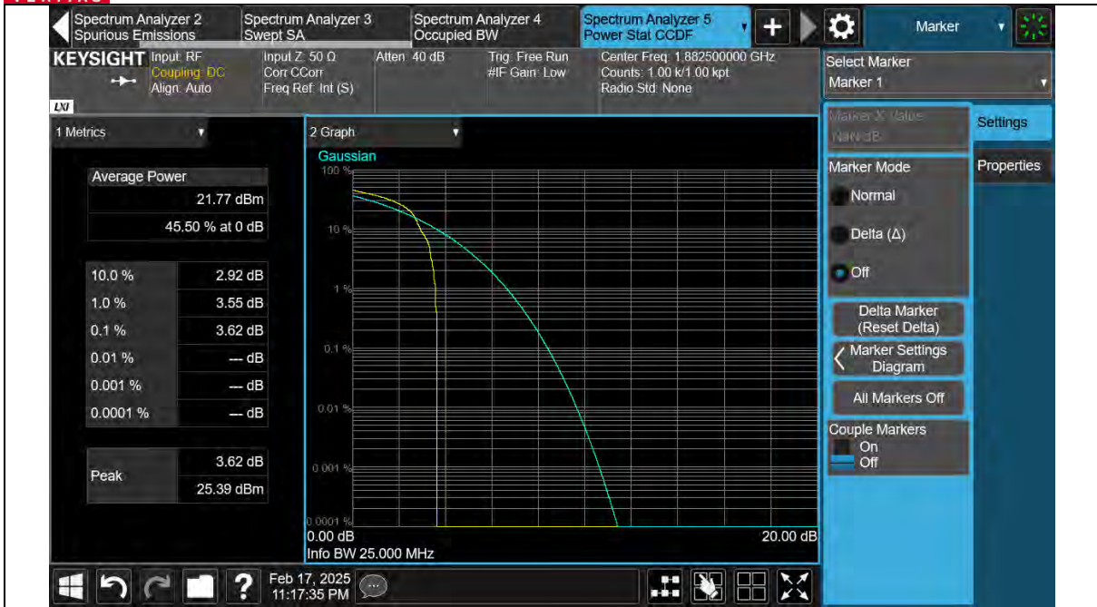
Band25-20MHz-16QAM-26365-1RB#0
