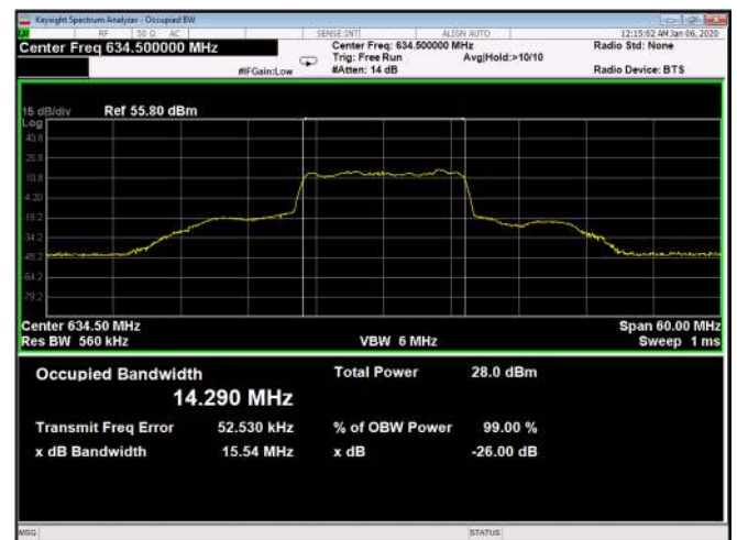
Figure 608: QPSK 15MHz B.W; 634.5MHz, 15kHz Output
