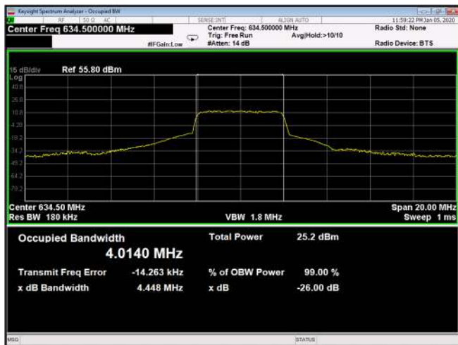
Figure 593: QPSK 5MHz B.W; 634.5MHz, 30kHz Output
