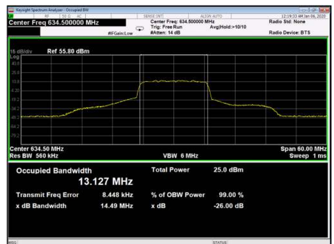
Figure 610: QPSK 15MHz B.W; 634.5MHz, 60kHz Output
