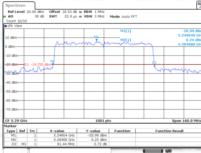
11AX80-CDD_Ant2_5290
