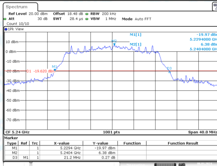
11AC20-CDD_Ant1_5240
