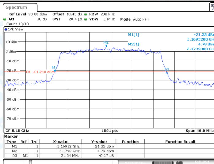
11AX20-CDD_Ant1_5180
