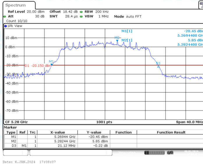
11AC20-CDD_Ant2_5280
