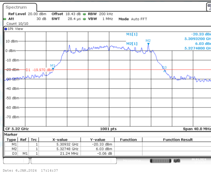
11AC20-CDD_Ant2_5320
