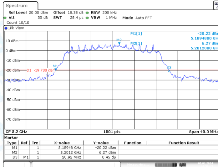
11AC20-CDD_Ant2_5200
