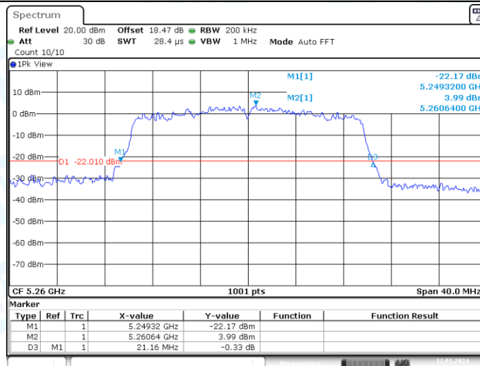
11AX20-CDD_Ant1_5260
