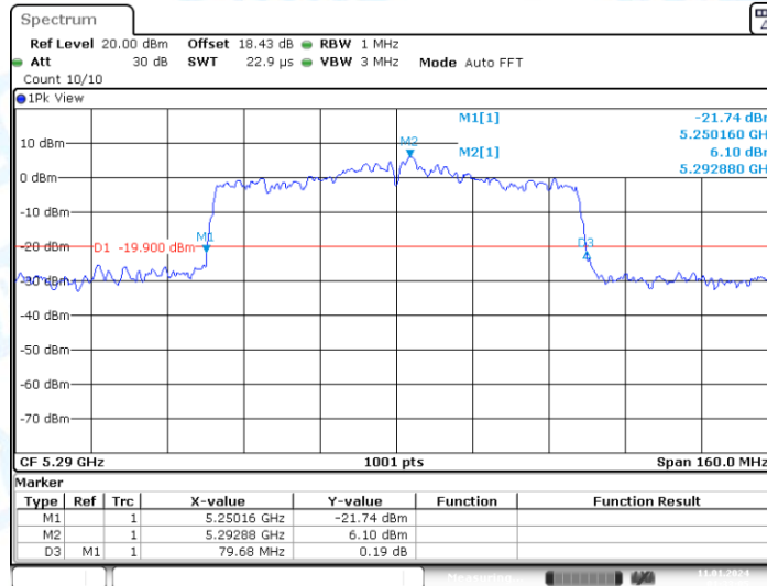
11AC80-CDD_Ant2_5290
