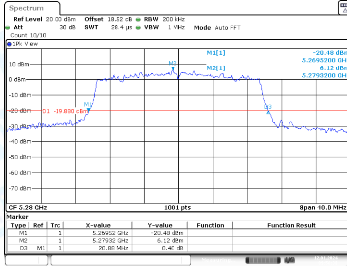
11AX20-CDD_Ant2_5280
