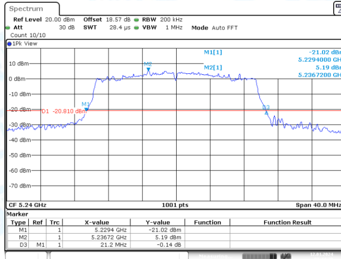
11AX20-CDD_Ant2_5240
