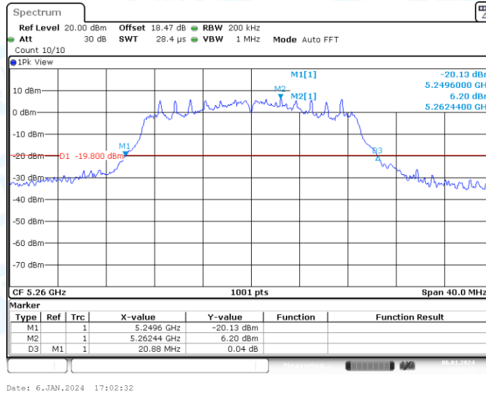
11AC20-CDD_Ant2_5260
