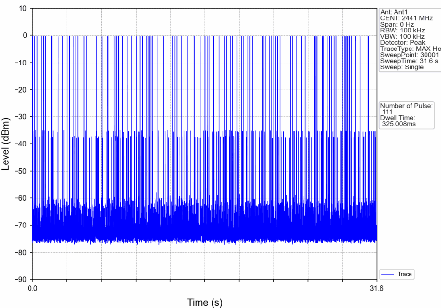
GFSK_DH5_HOPP_Ant1_NTNV
