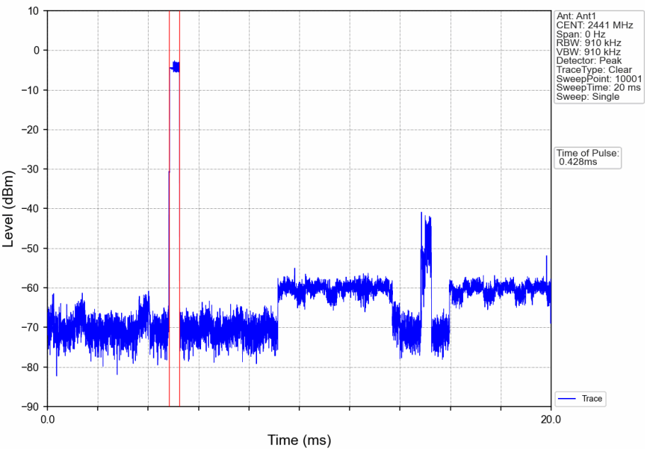
Pi/4DQPSK_2DH1_HOPP_Ant1_NTNV
