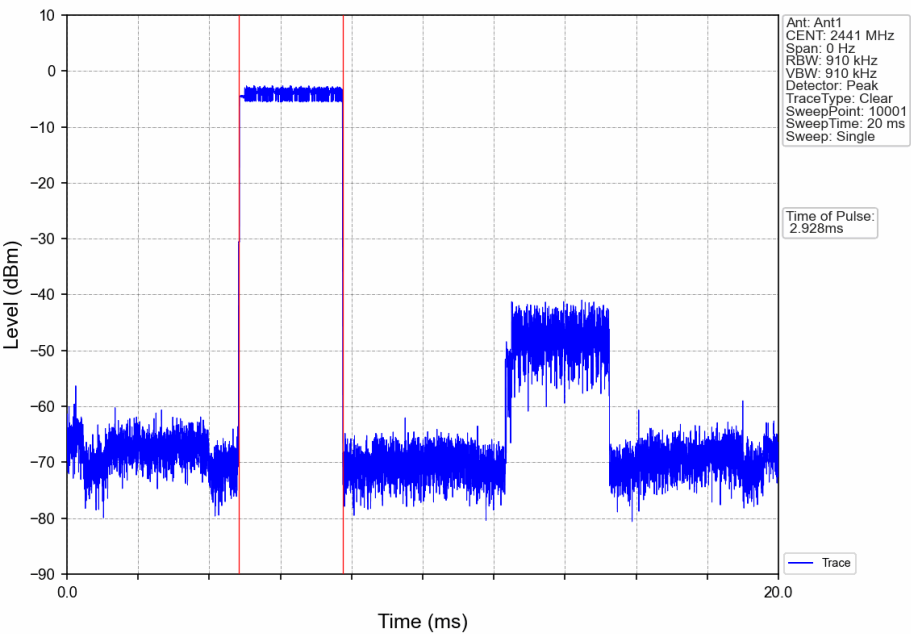
Pi/4DQPSK_2DH5_HOPP_Ant1_NTNV
