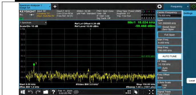
Band4-20MHz-QPSK-20175-1RB#0-0.009~0.15-PASS
