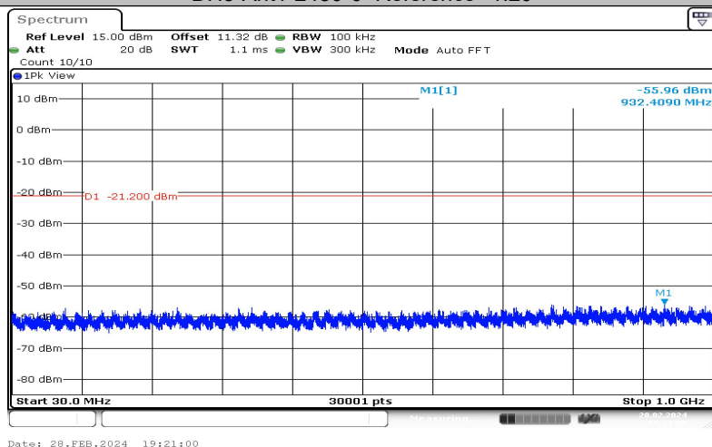
DH5-Ant1-2480-30~1000--1.20
