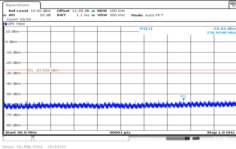
2DH5-Ant1-2402-30~1000--7.01
