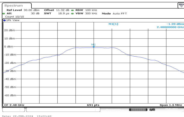
DH5-Ant1-2480-0~Reference--1.20
