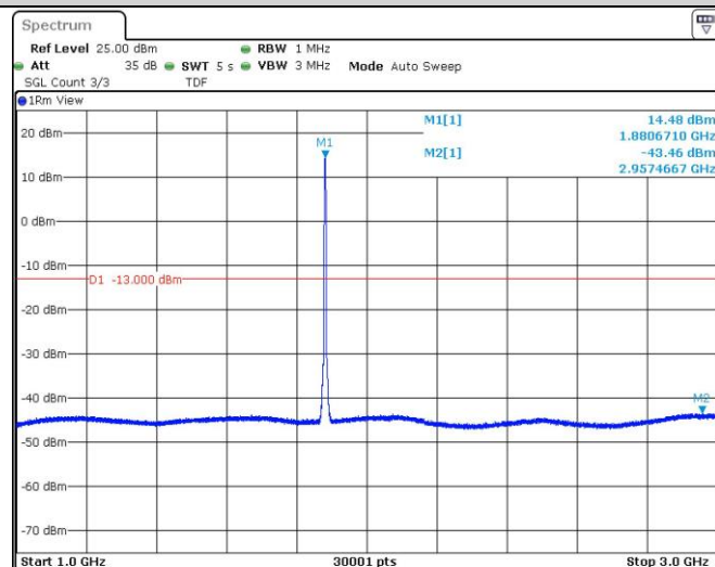
Band2-9400-4-1000~3000MHz
