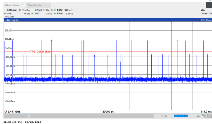
3DH5_Ant1_Hop
