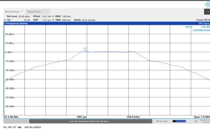
DH5_Ant1_2480_0-Reference
