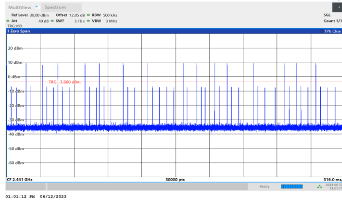
3DH3_Ant1_Hop
