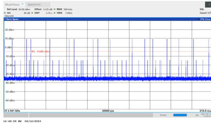
DH3_Ant1_Hop
