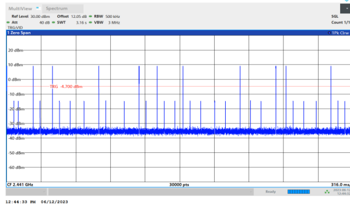
DH5_Ant1_Hop
