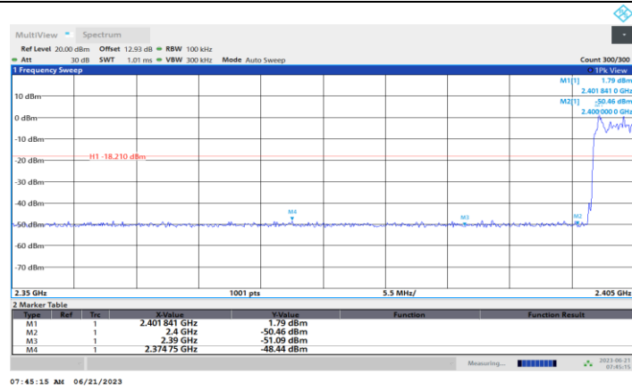
3DH5_Ant1_Low_Hop_2402
