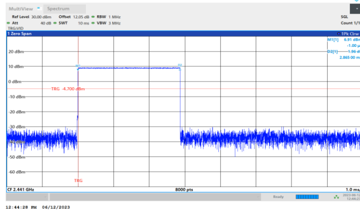
DH5_Ant1_Hop
