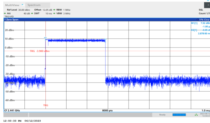
3DH5_Ant1_Hop
