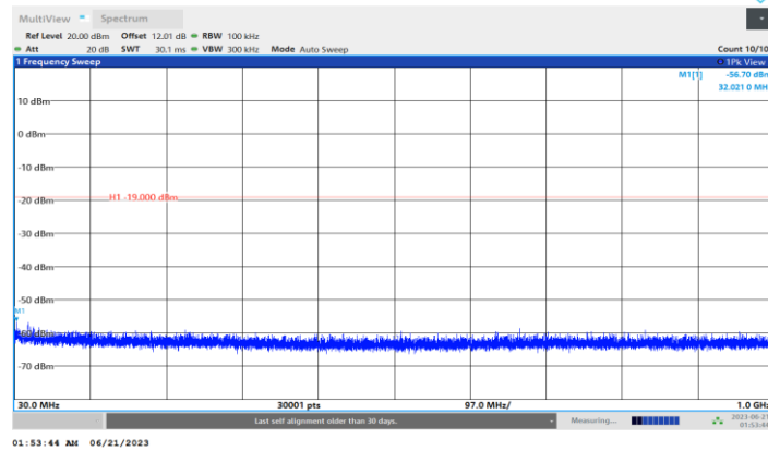
DH5_Ant1_2480_30-1000
